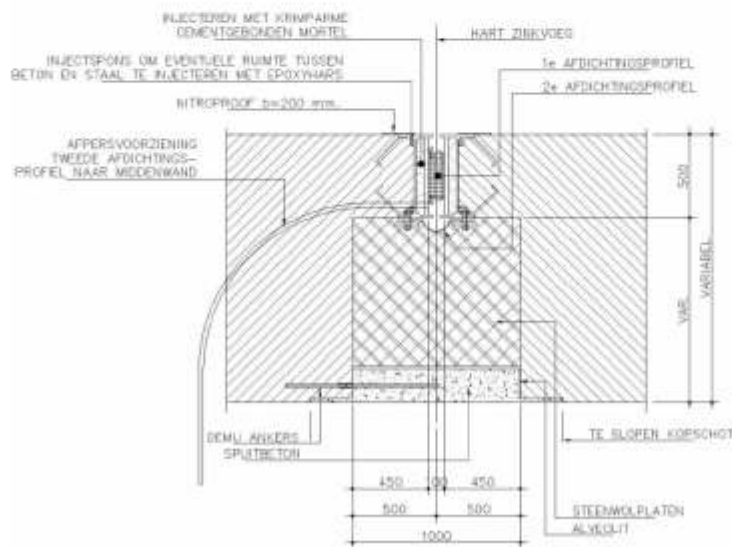
DETAILONTWERP AFWERKING ZINKVOEG DAK MIDDENKANAAL ( BIJ TOEPASSING STAAL DEUVEL IN VLOER VERKEERSKORDE )
