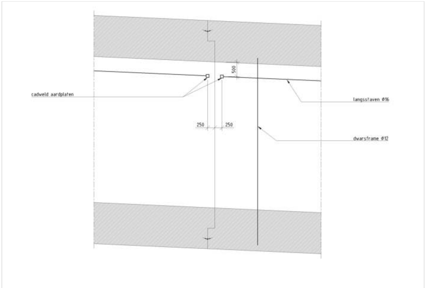
Figuur 288.2 - Aanzicht middenwandkanaal
