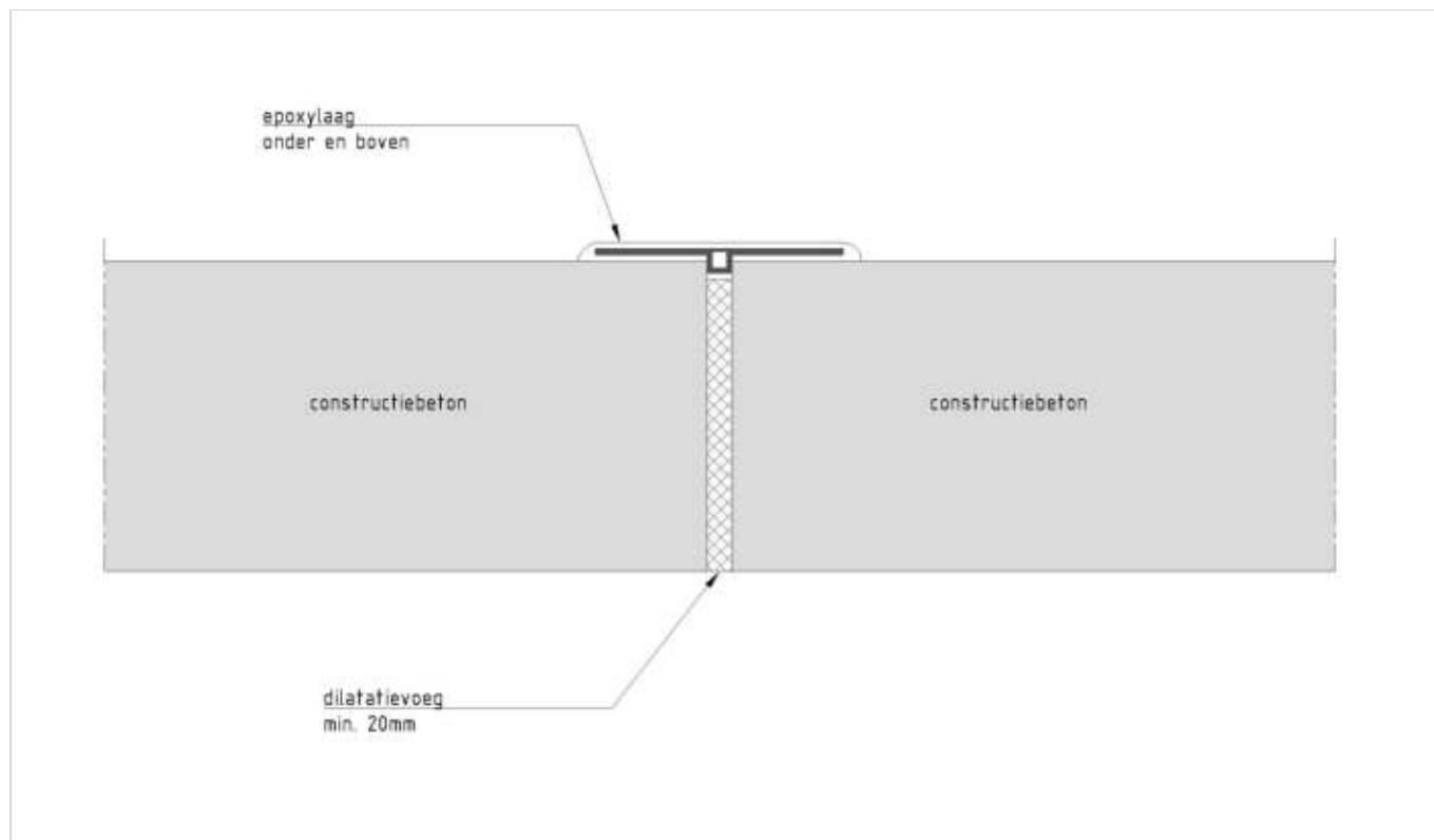
Figuur 257.2 - Buitenafdichting met epoxylaag
