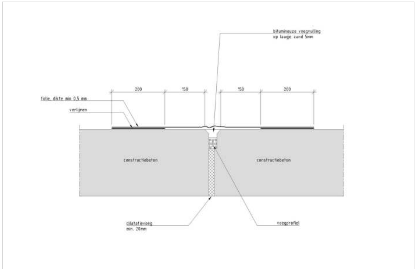
Figuur 257.1 - Voeg buitenzijde dak
