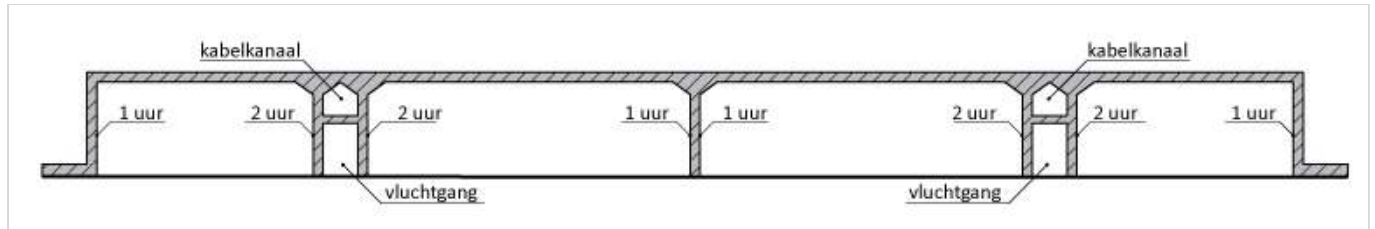
Figuur 554.1 - Voorbeeld geleidewanden
