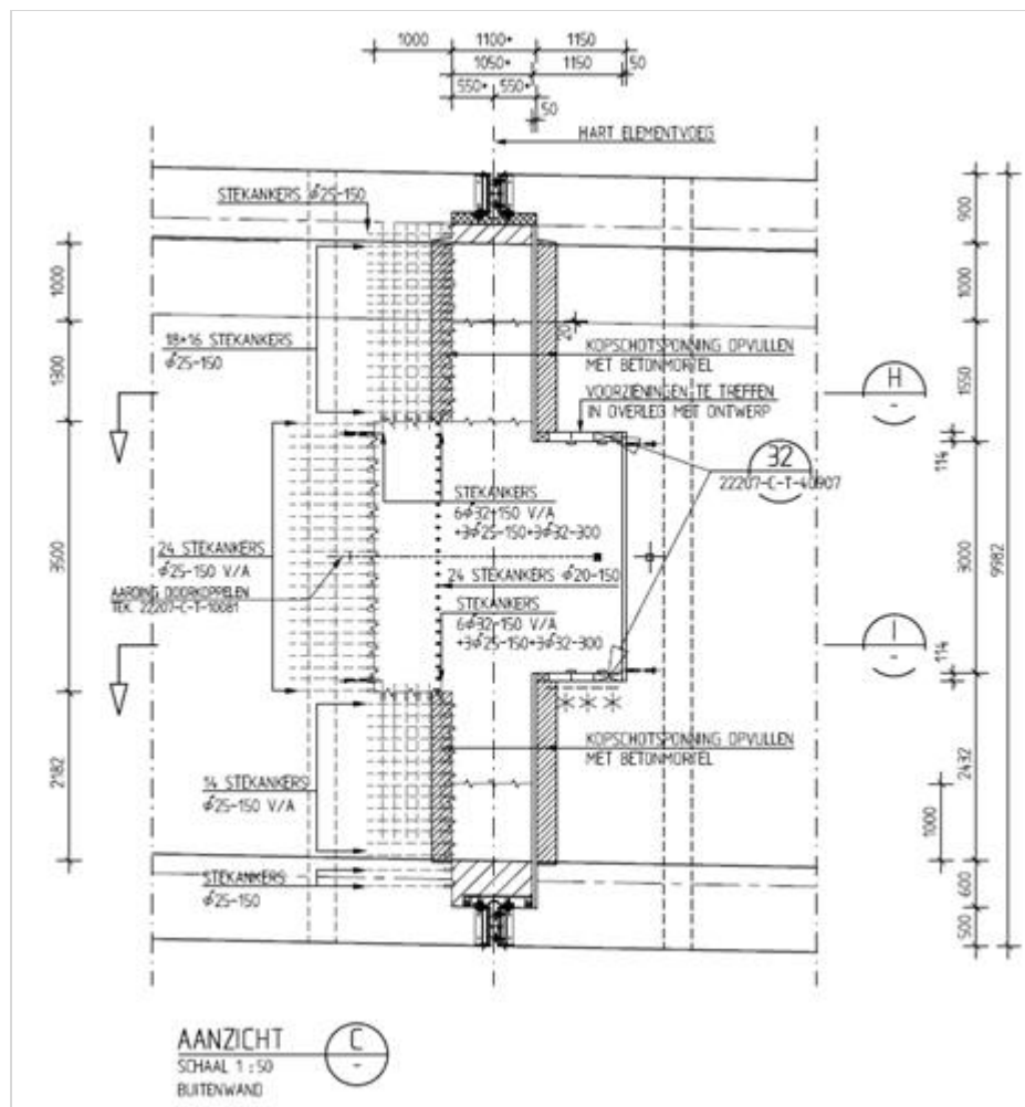
Figuur 370.2 - Zijaanzicht tand tussen de zinkvoegen in de buitenwand van de HSL tunnel onder de Oude Maas
