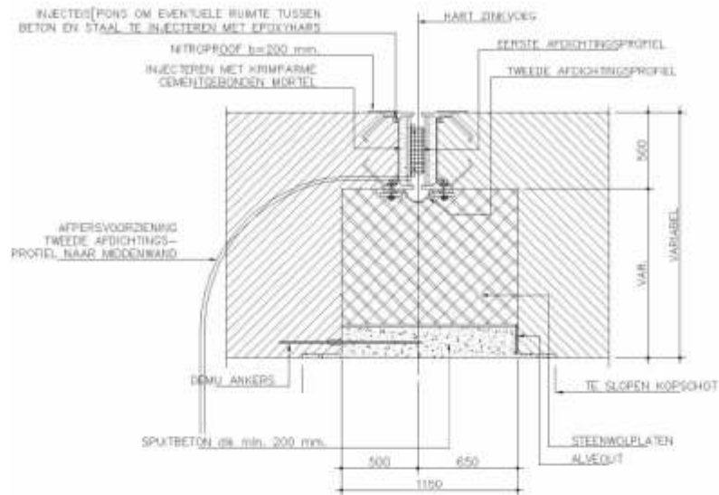
DETAILONTWERP AFWERKING ZINKVOEG DAK MIDDENKANAAL ( BIJ TOEPASSING TANDOPLOSSING IN VLOER VERKEERSKORDE )
