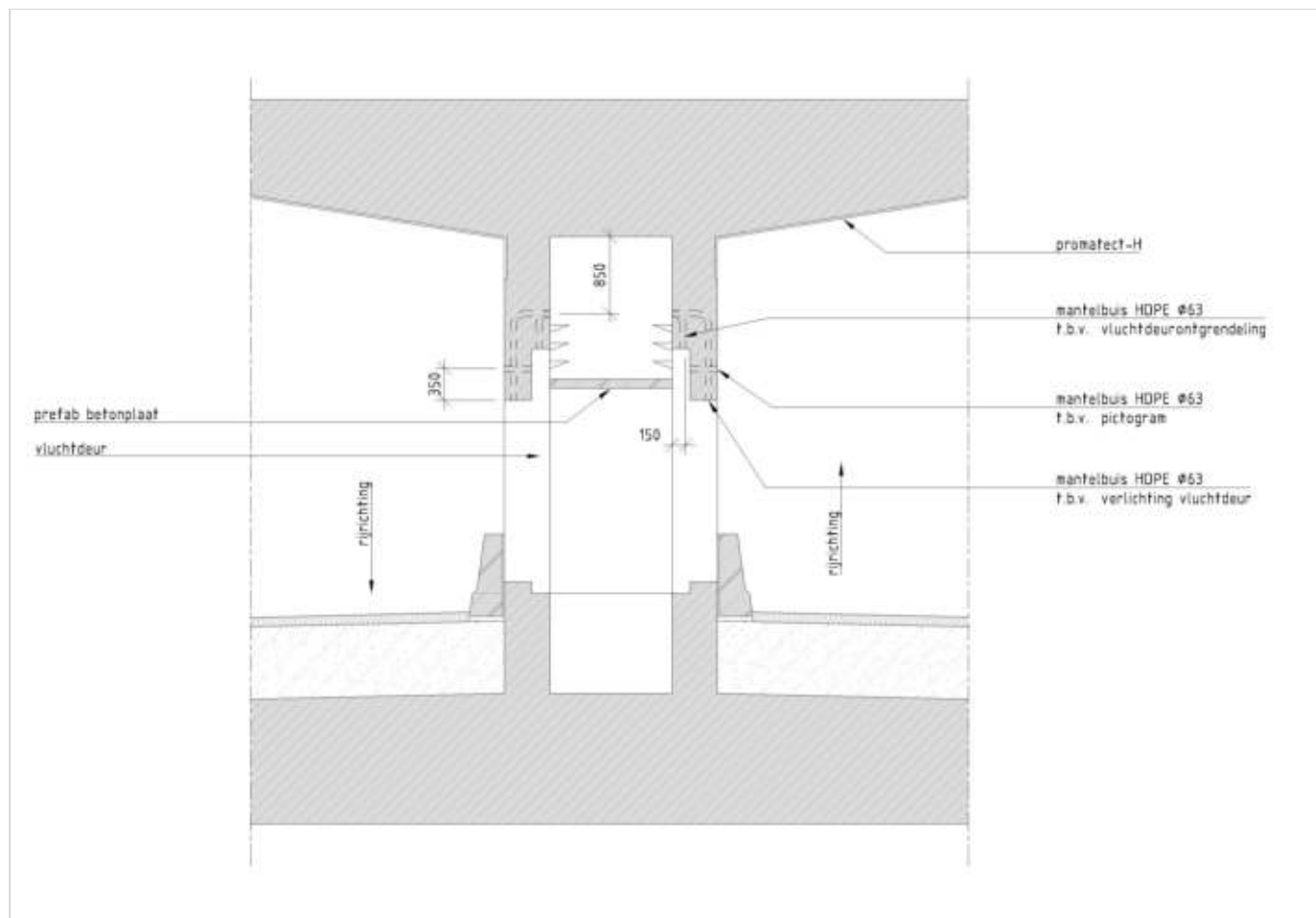
Figuur 282.1 - Doorsnede middenkanaal vluchtdoor (schuifdeur)
