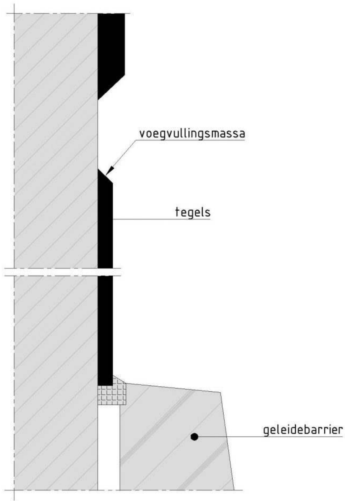
Figuur 507.2 - Principedetails wandafwerking tegels t.p.v. dilatatievoeg
