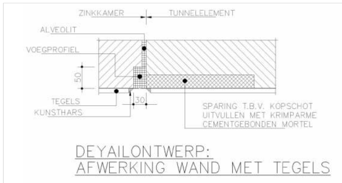
Figuur 362.1 - Detailontwerp: afwerking wand met tegels
