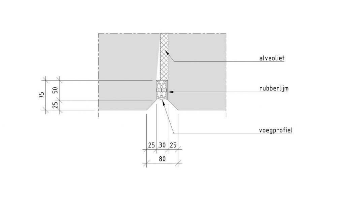
Figuur 263.1 - Detailontwerp voegprofiel
