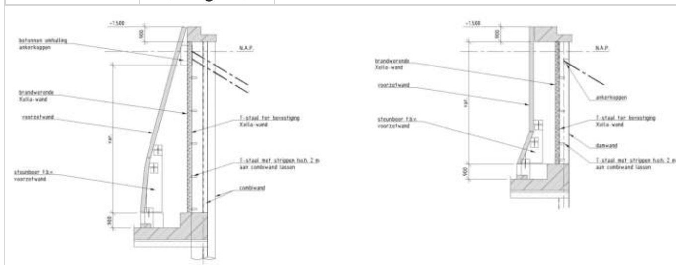
Figuur 314.1 - Voorzetwand A4 Leiderdorp
