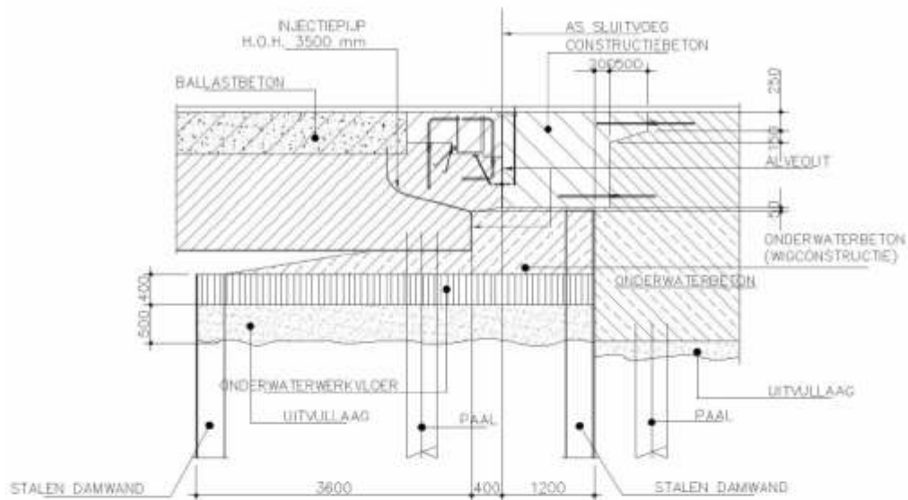
DETAILONTWERP AFWERKING VLOER ( OP PALEN )
