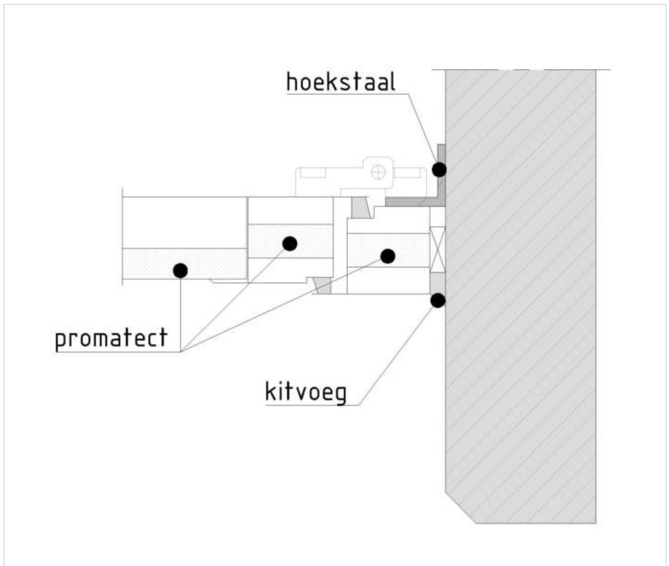
Figuur 491.1 - Detail montage kozijn vluchtdeur (draaideur)
