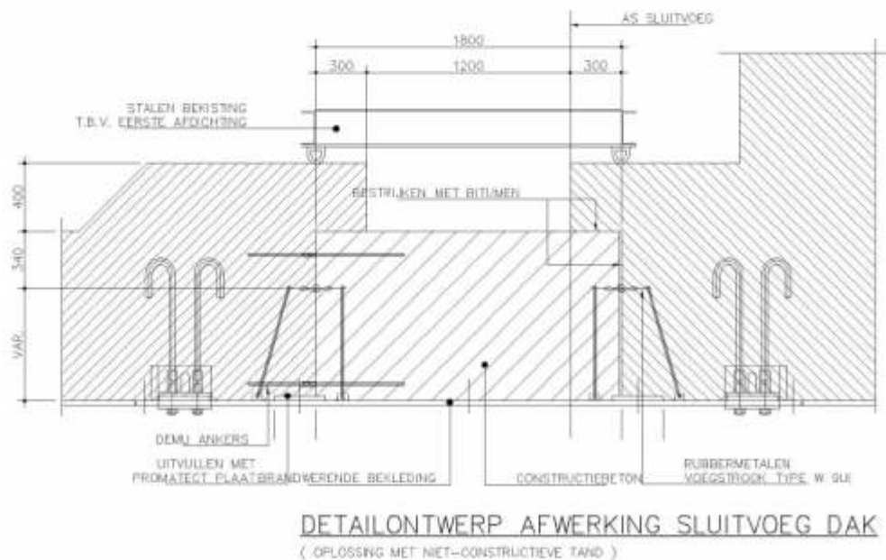
Figuur 347.1 - Detailontwerp afwerking sluitvoeg dak
