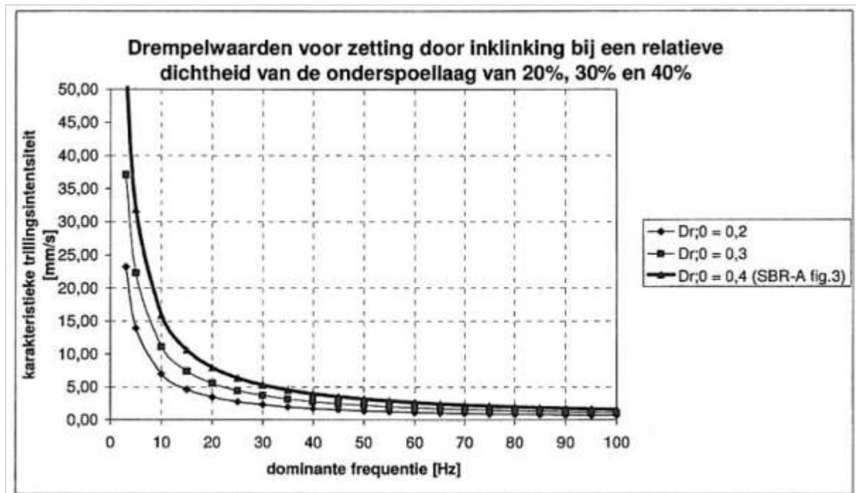
Figuur 530.1 - Voorbeeld gebruik van drempelwaarden met grafiek van Hergarden
