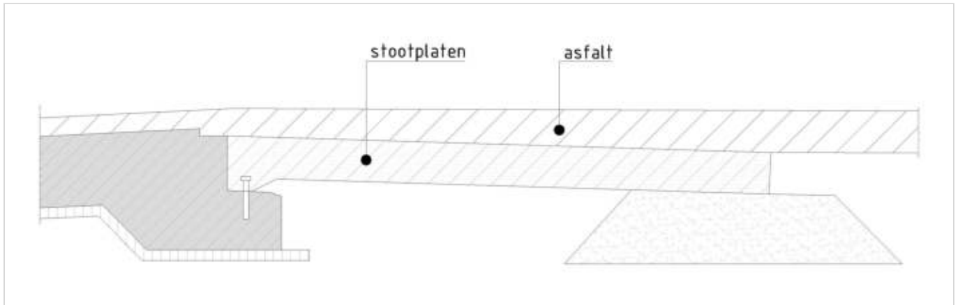
Figuur 470.1 - Detail stootplaat
