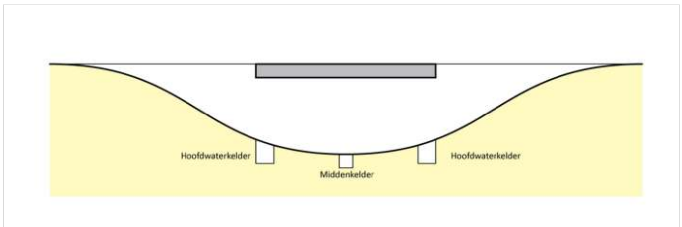
Figuur 382.2 - Lange tunnel met hoofdwatorkelders en middenkelder
