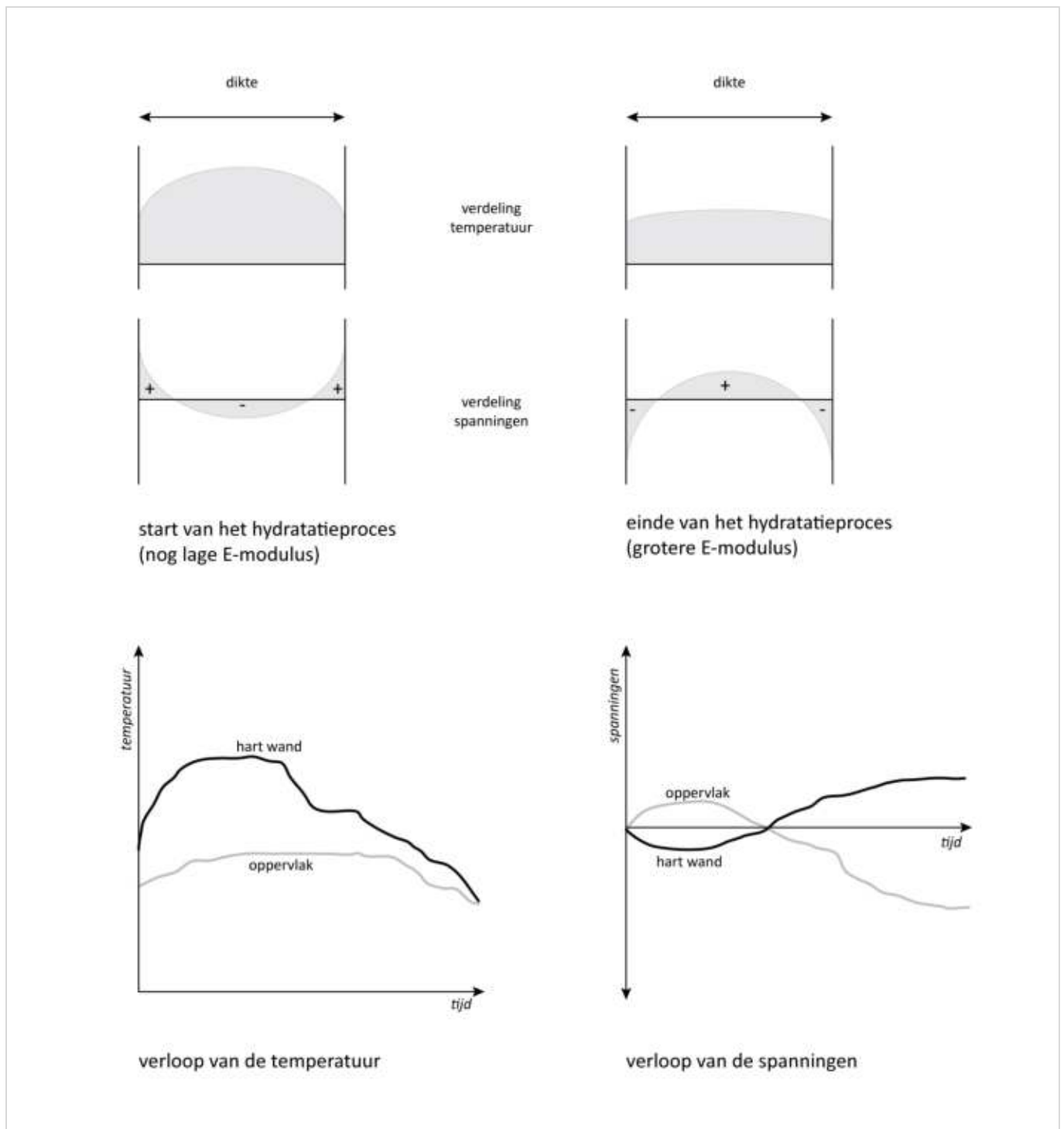
Figuur 664.1 - Principe van inwendige verhindering van hydratatievervormingen
