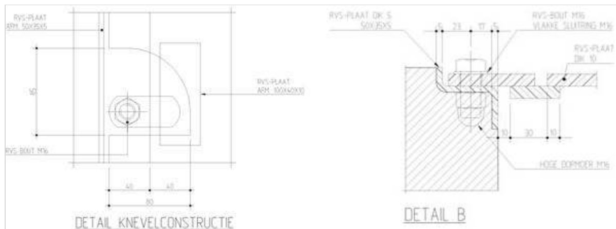
Figuur 456.2 - Details geleidebarrier middenkelder/hoofdwatorkelder
