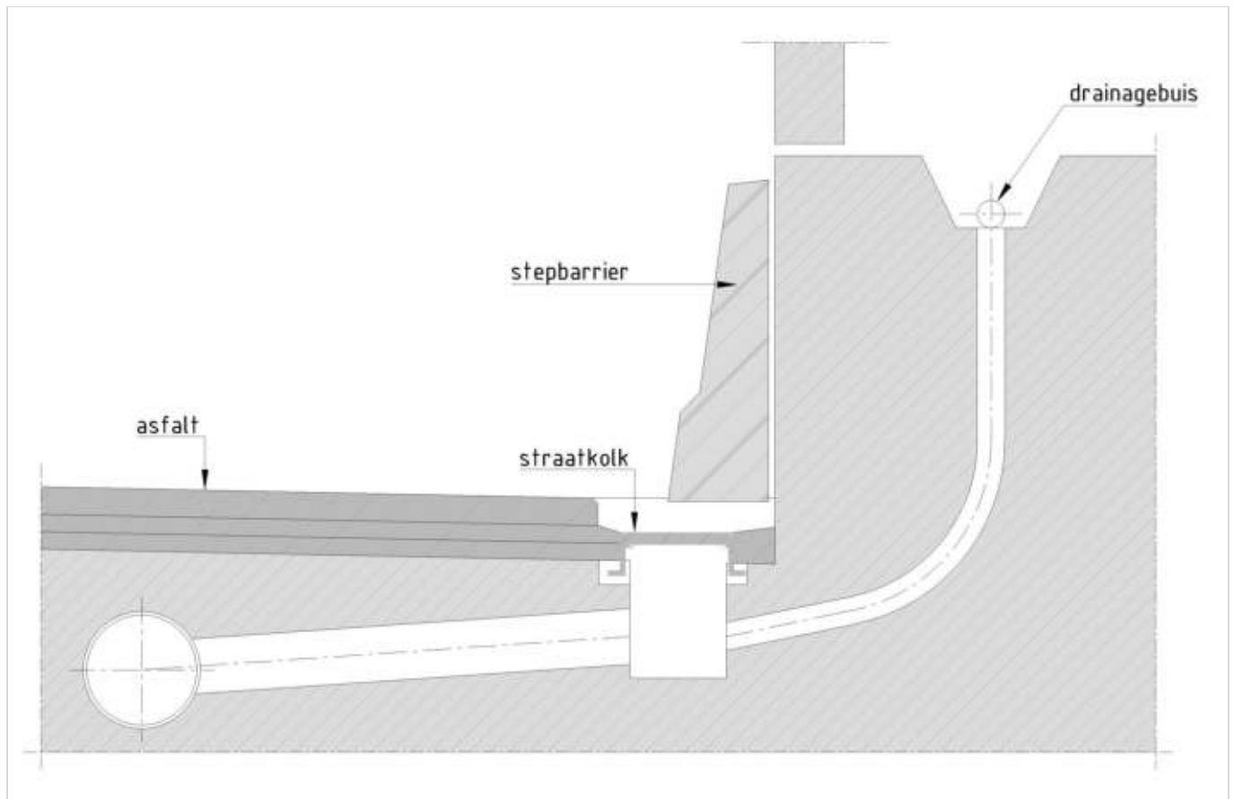
Figuur 412.1 - Aansluiting straatkolk op afvoerleiding
