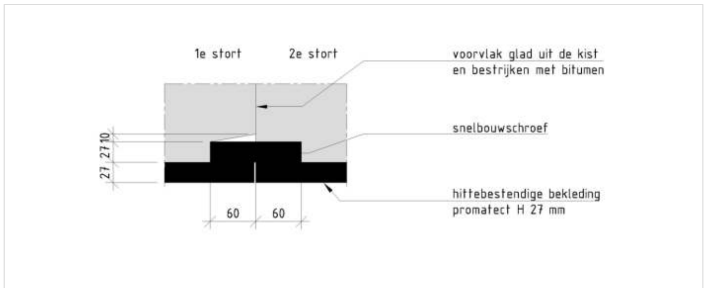
Figuur 268.1 - Detailontwerp hittewerende bekleding methode A;
