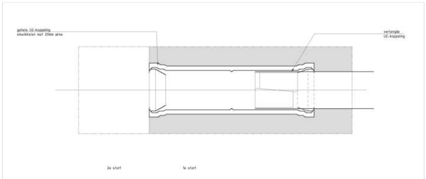
Figuur 270.3 - Verlengde U2-koppeling
