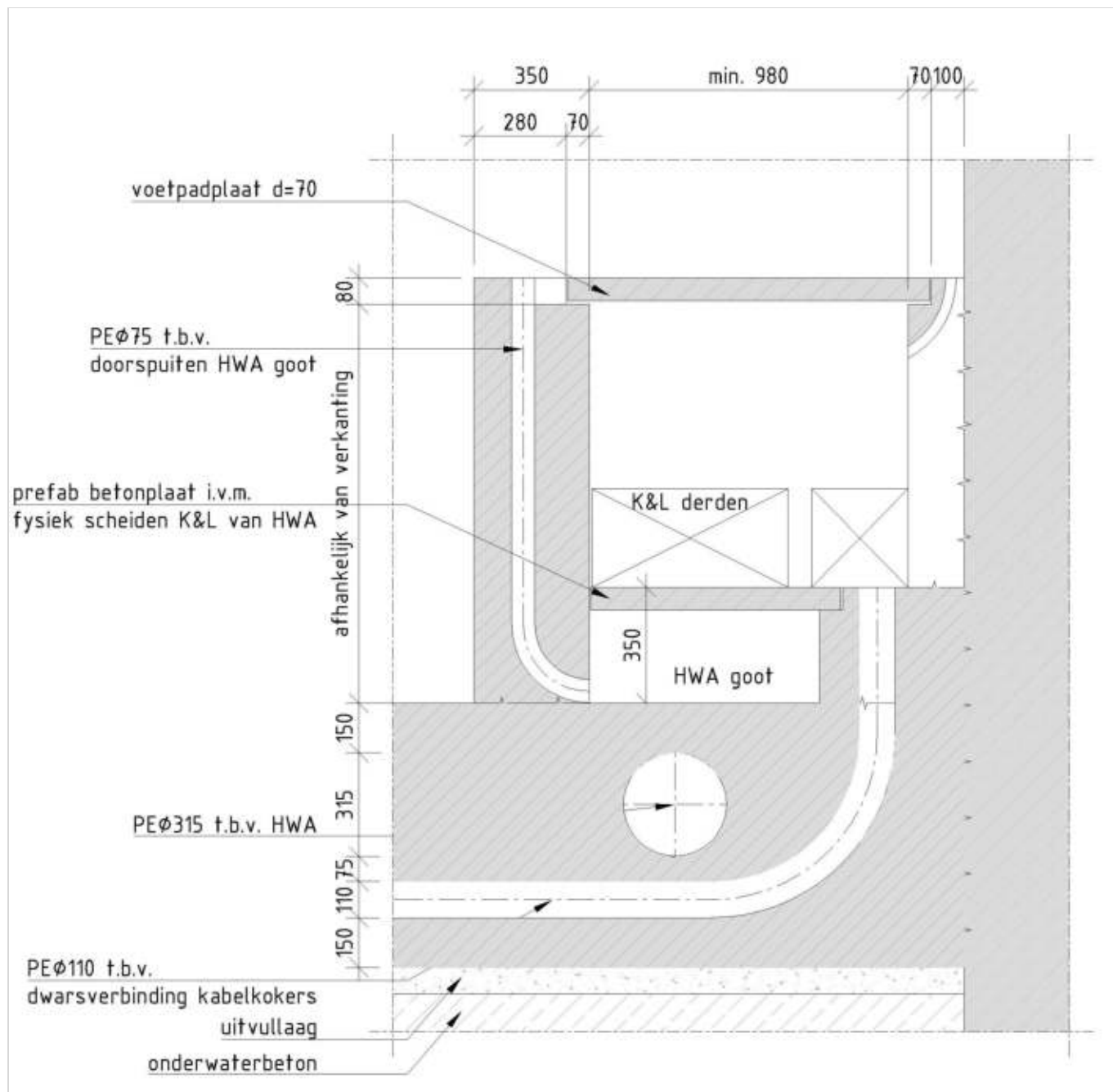
Figuur 398.3 - Afvoergoot met doorspuitleiding
