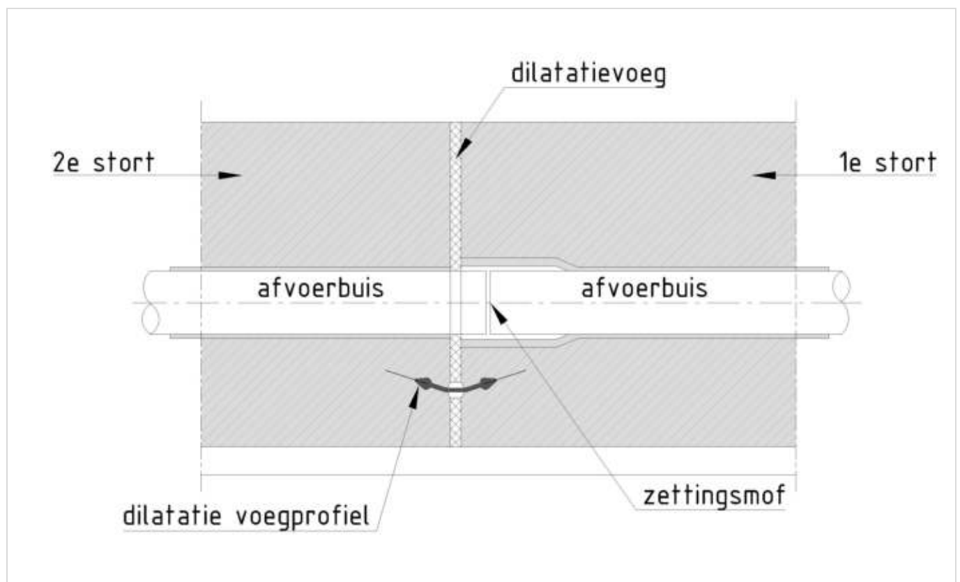
Figuur 502.1 - Principe doorsnede afvoerbuis t.p.v. voegovergang
