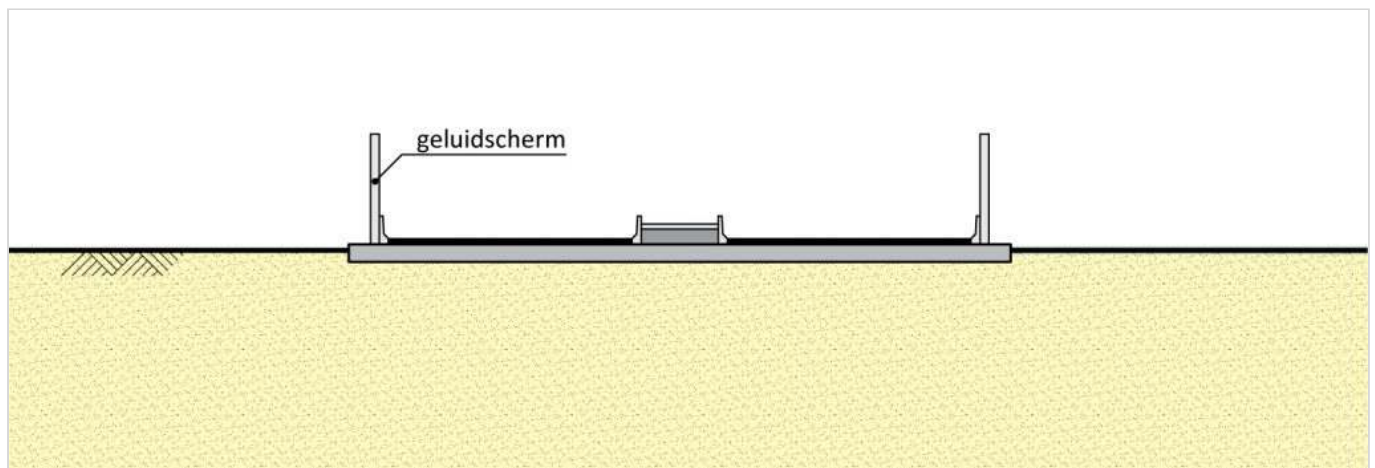
Figuur 10.3 - Weg voorzien van geluidsschermen (valt buiten de scope van dit handboek)
