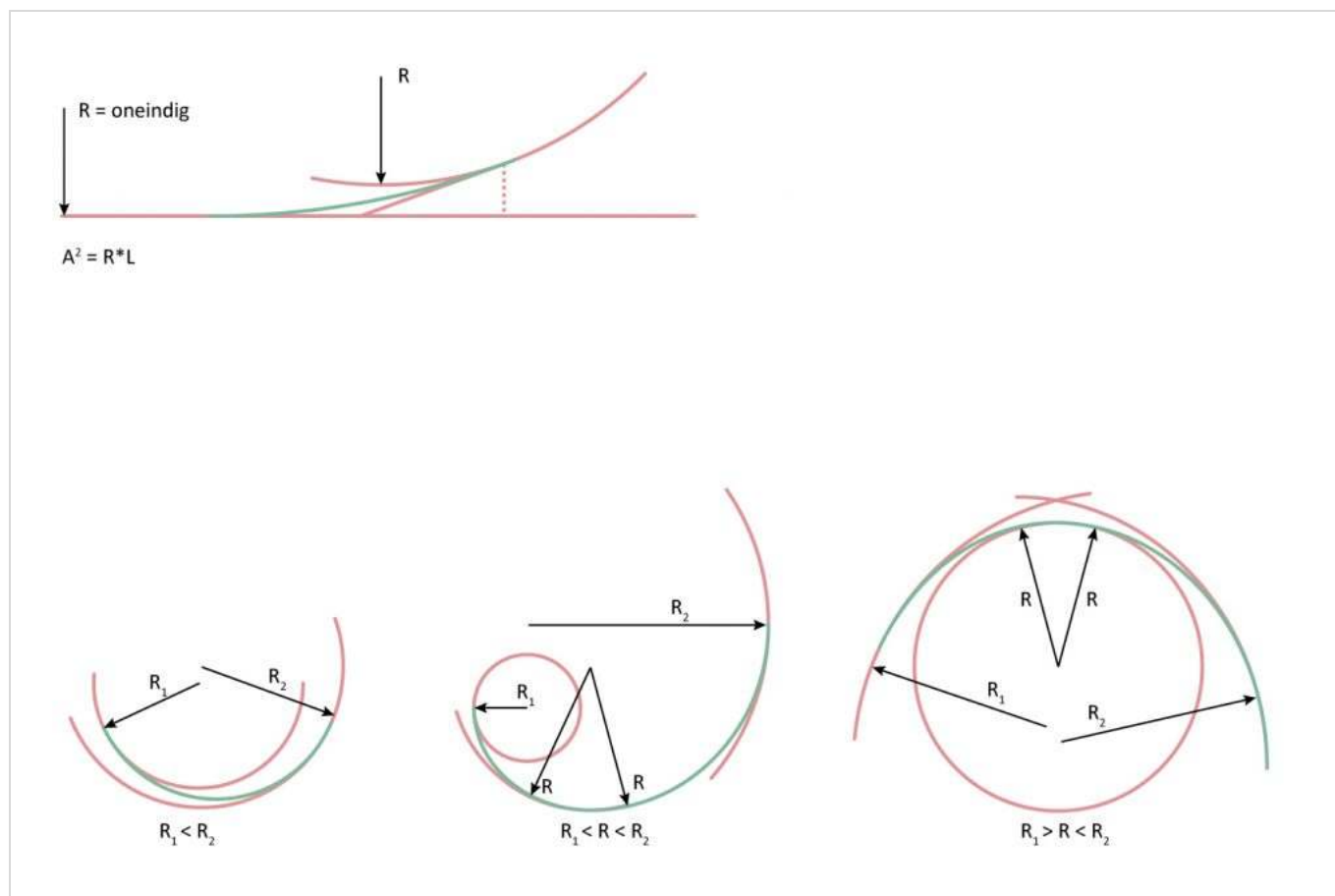
Figuur 19.1 - Clothoïde
