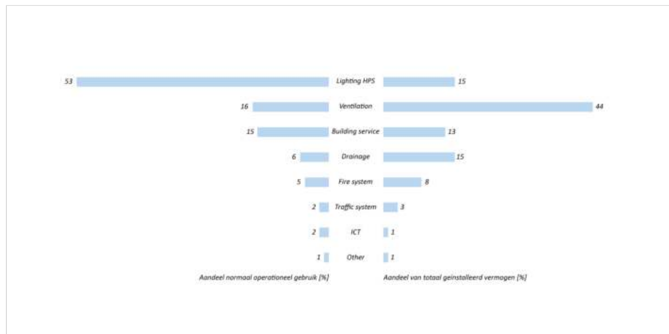
Figuur 415.1 - Aandeel van geïnstalleerd vermogen per installatie [%] van het totaal geïnstalleerd vermogen
