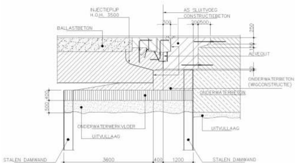
DETAILONTWERP AFWERKING VLOER ( OP STAAL )
