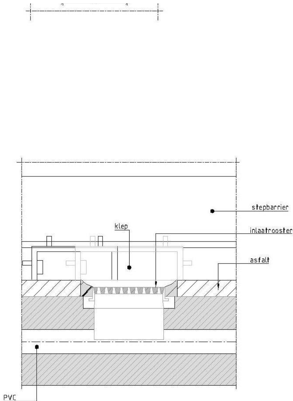
Figuur 388.1 - Inlaatputten bij toepassing ZOAB
