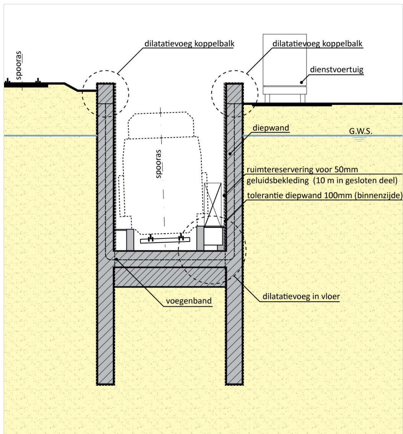
Figuur 413.1 - Doorsnede toerit dive-under Vleugel
