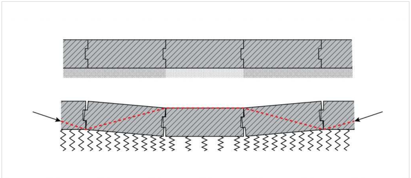
Figuur 100.3 - Verloop druklijn als gevolg van verschilzakking.
