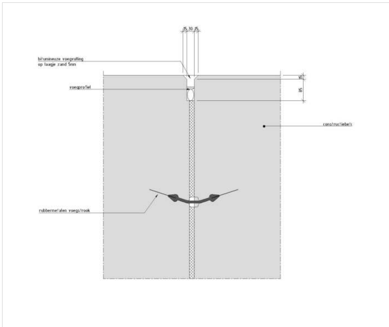
Figuur 265.1 - Voorbeeld afdichting ten behoeve van calamiteitendichting (gevaarlijke stoffen)
