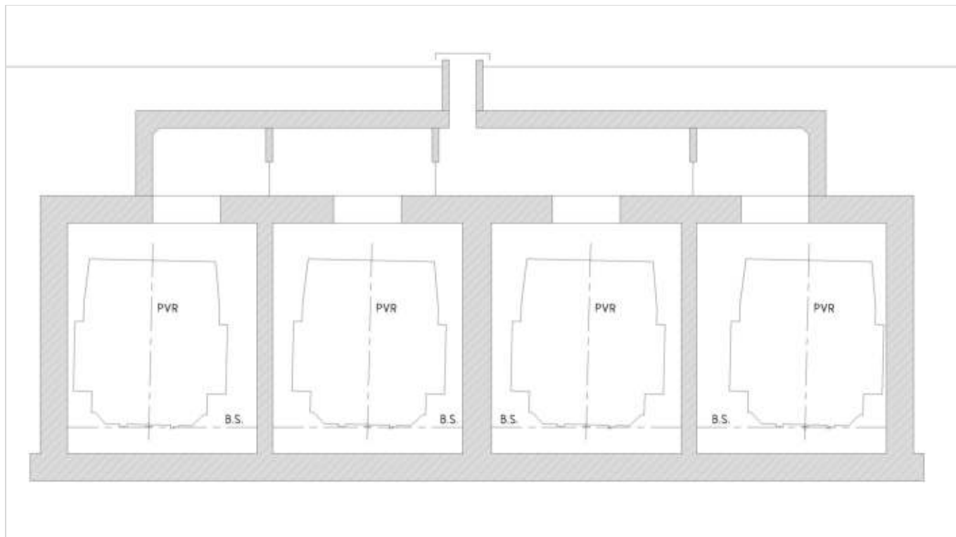
Figuur 497.1 - Drukvereffeningssysteem spoortunnel (gesloten systeem tussen tunnelbuizen onderling)
