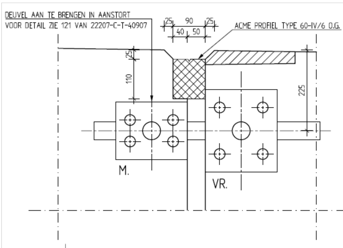
Figuur 370.7 - Horizontale stalen verdeuveling bij de zinkvoeg in de vloer van de HSL-tunnels
