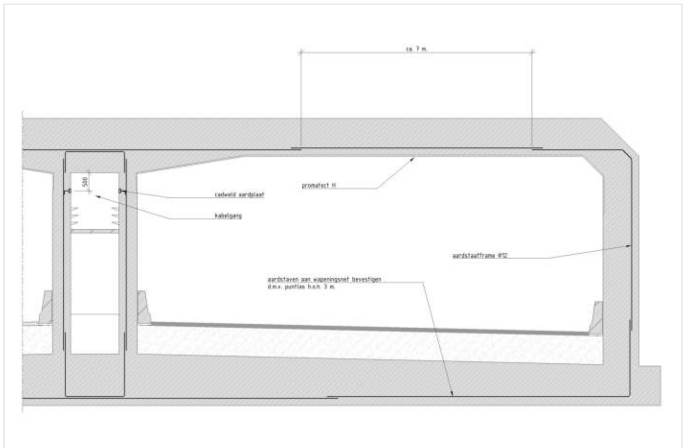
Figuur 288.1 - Doorsnede aardstaaf dwarsframe Ø 12 mm
