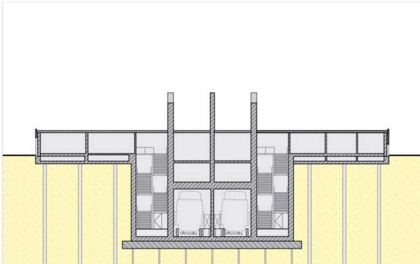
Figuur 446.4 - Dwarsdoorsnede dienstgebouw Drontermeertunnel
