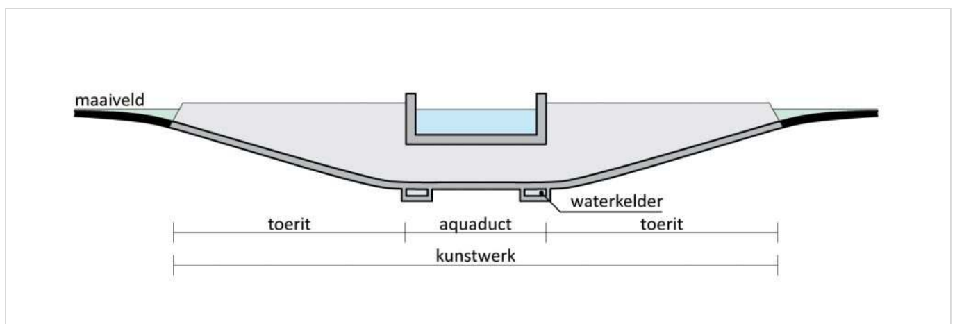
Figuur 8.1 - Aquaduct
