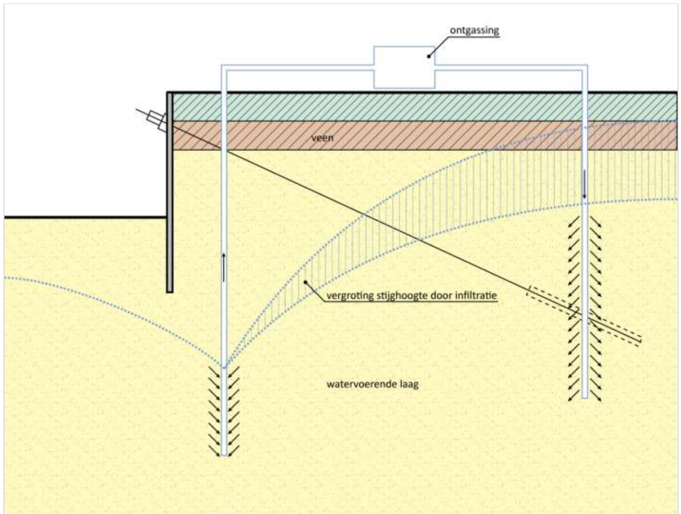
Figuur 166.5 - Retourbemaling
