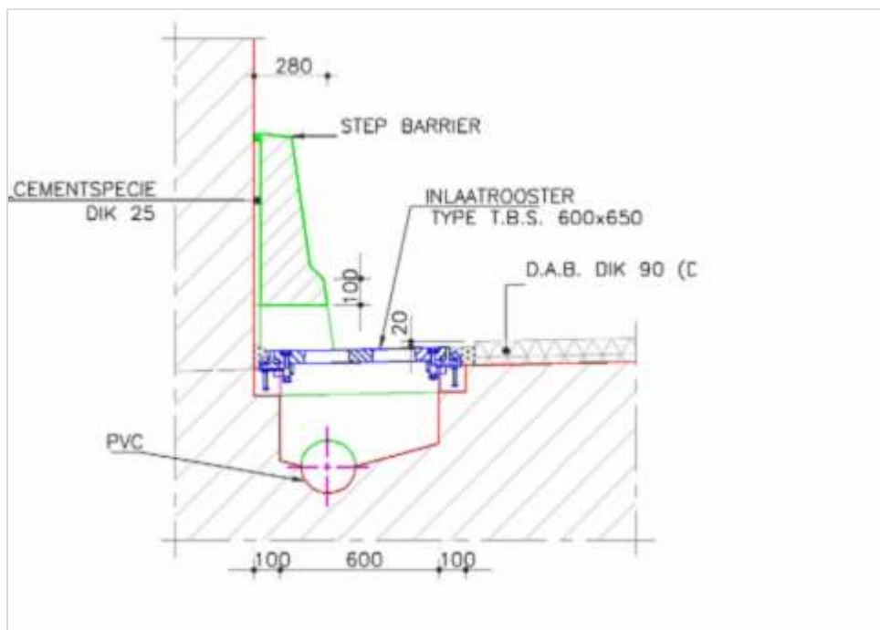
Figuur 387.3 - Inlaatputten (bij toepassing DAB), deel 2
