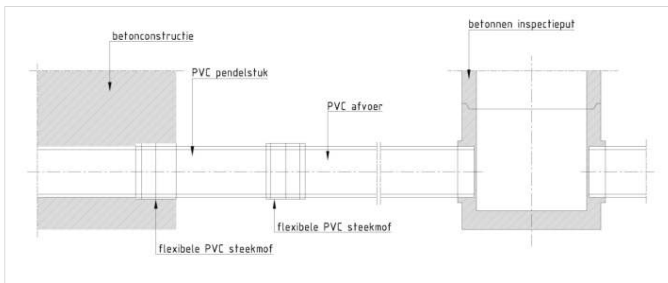
Figuur 391.1 - Aansluiting inspectieput-betonconstructie
