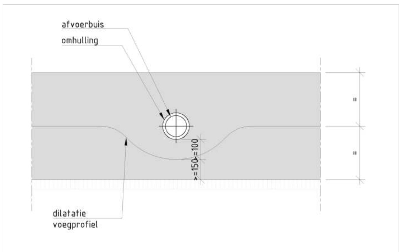
Figuur 251.1 - Dilatatatievoegprofiel nabij hemelwaterafvoerbuis in vloer
