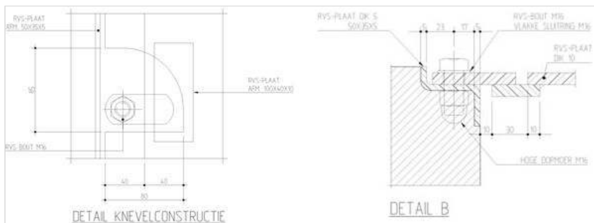
Figuur 456.2 - Details geleidebarrier middenkelder/hoofdwaterkelder
