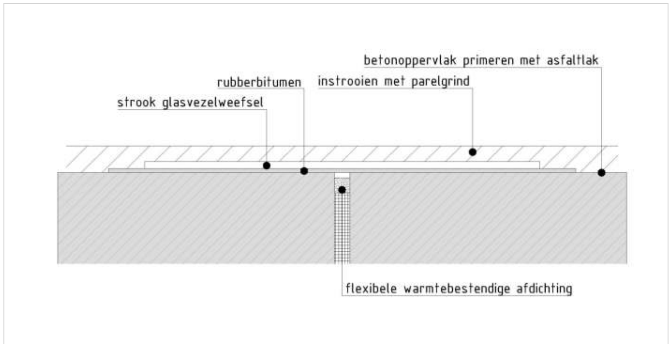
Figuur 471.1 - Detail voegafdekking
