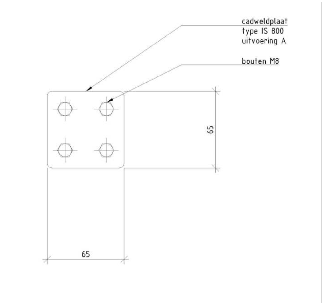
Figuur 288.4 - Detail aardplaat (anker is niet getekend)
