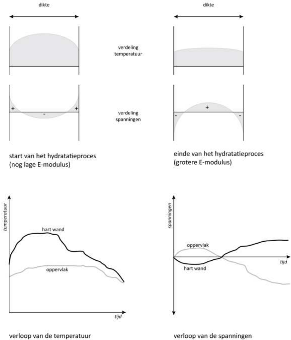
Figuur 664.1 - Principe van inwendige verhindering van hydratatievervormingen
