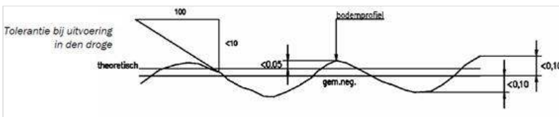
Figuur 591.2 - Tolerantie bij uitvoering in den droge
