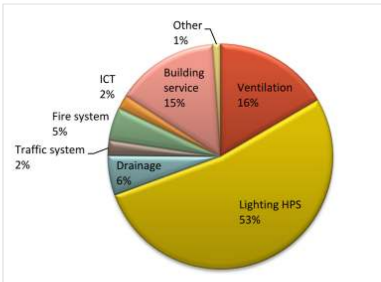
Figuur 415.2 - Aandeel van energieverbruik [%] bij normaal operationeel gebruik. Bron: Zero Energy Tunnel: renewable Energy Generation and Reduction of Energy Consumption van Rimma Dzhusupova
