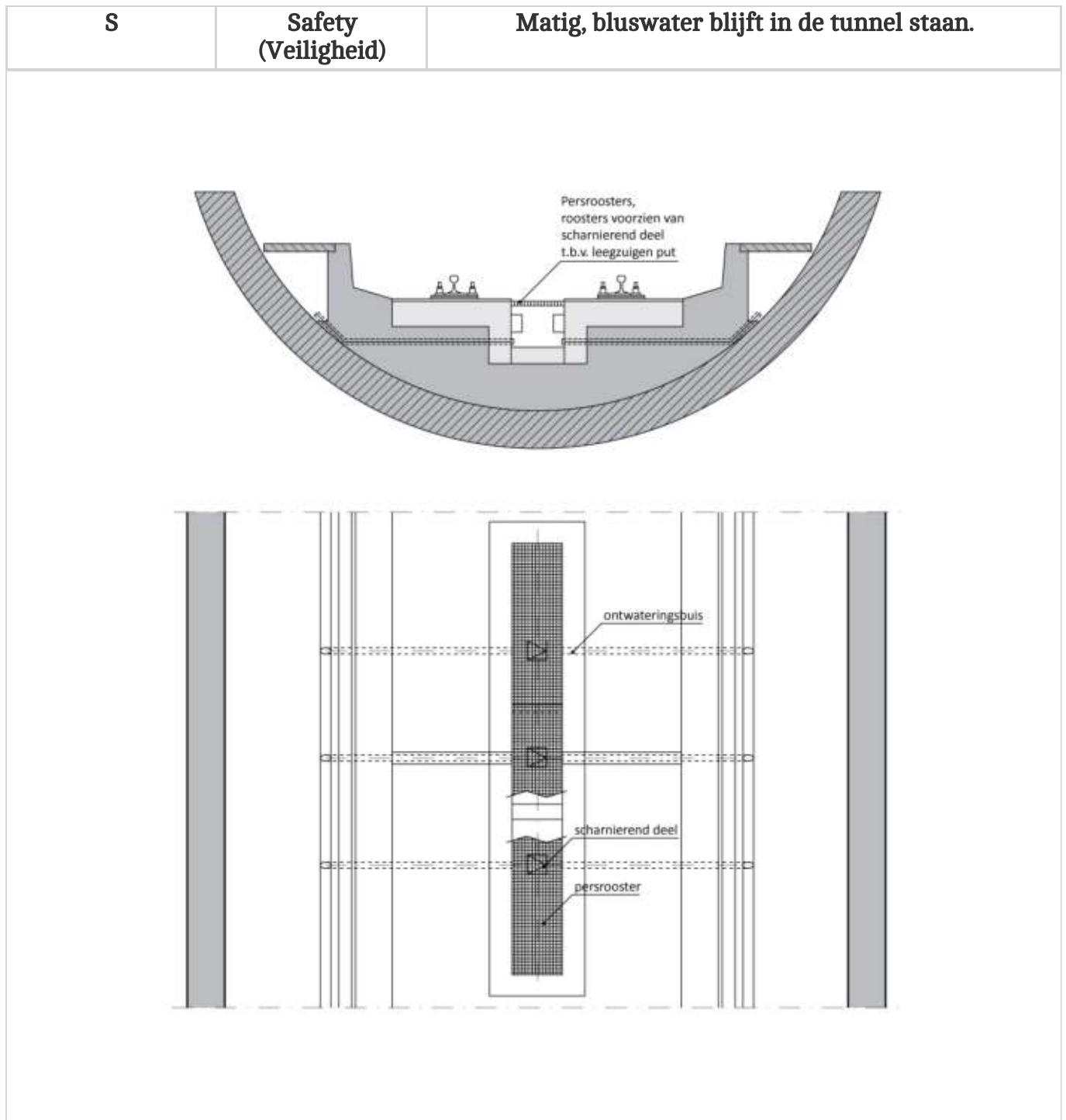
Figuur 400.2 - Pompput Boortunnel Noordzijdlijn Amsterdam
