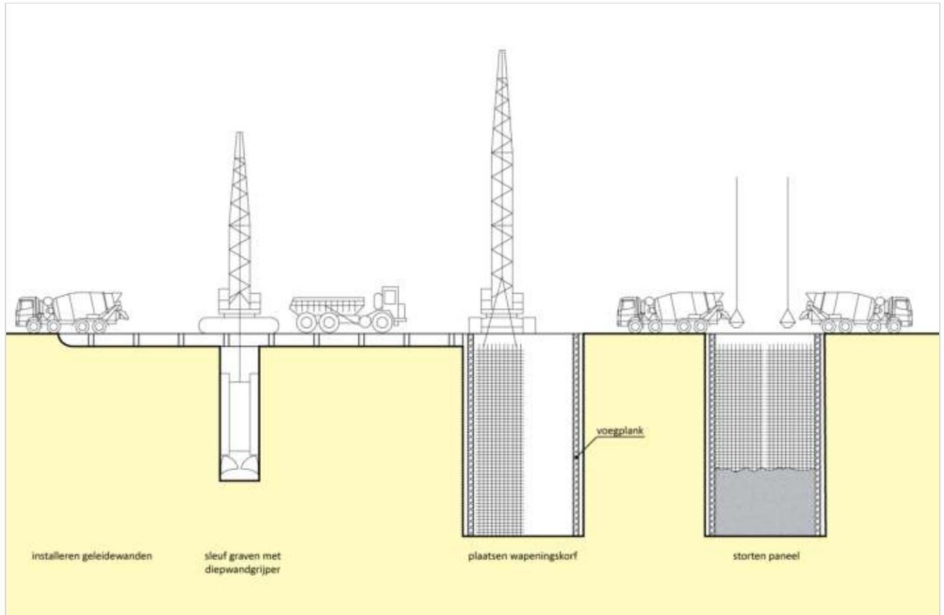
Figuur 555.1 - Methode diepwand
