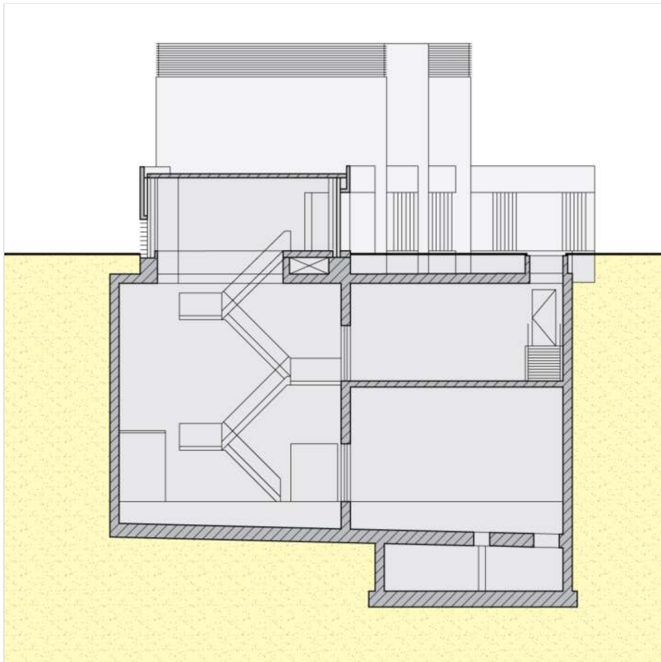
Figuur 446.3 - Langsdoorsnede dienstgebouw Drontermeertunnel
