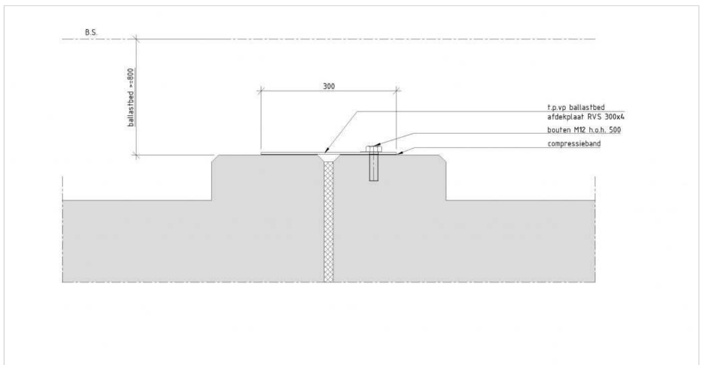
Figuur 266.2 - Voegovergang voor spoor in ballast zonder aanwezigheid van hemelwater
