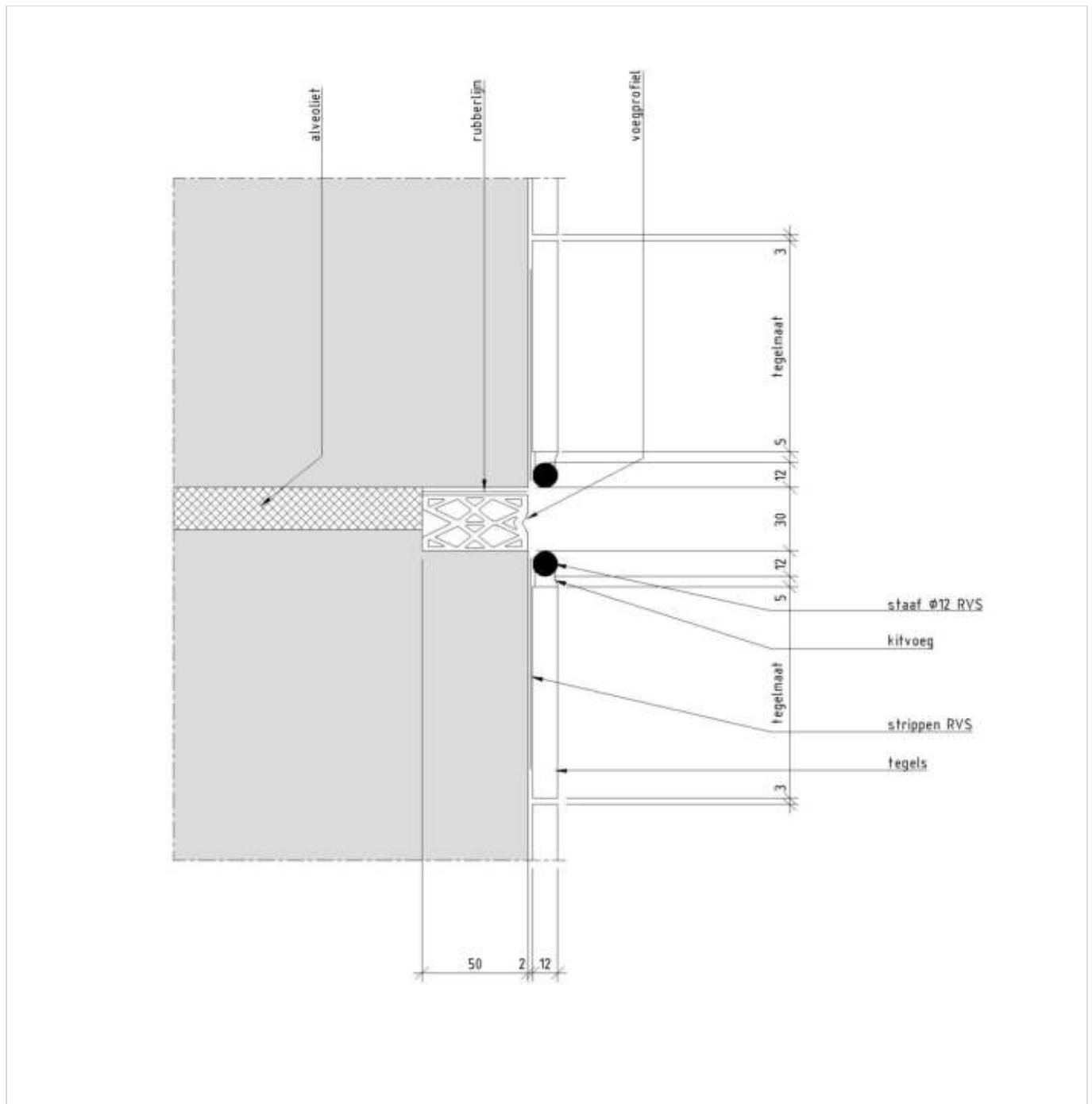
Figuur 264.2 - Detailontwerp tegelwerk - toepassing RVS staaf
