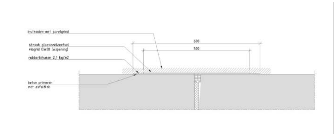
Figuur 265.2 - Voegovergang voor asfalt
