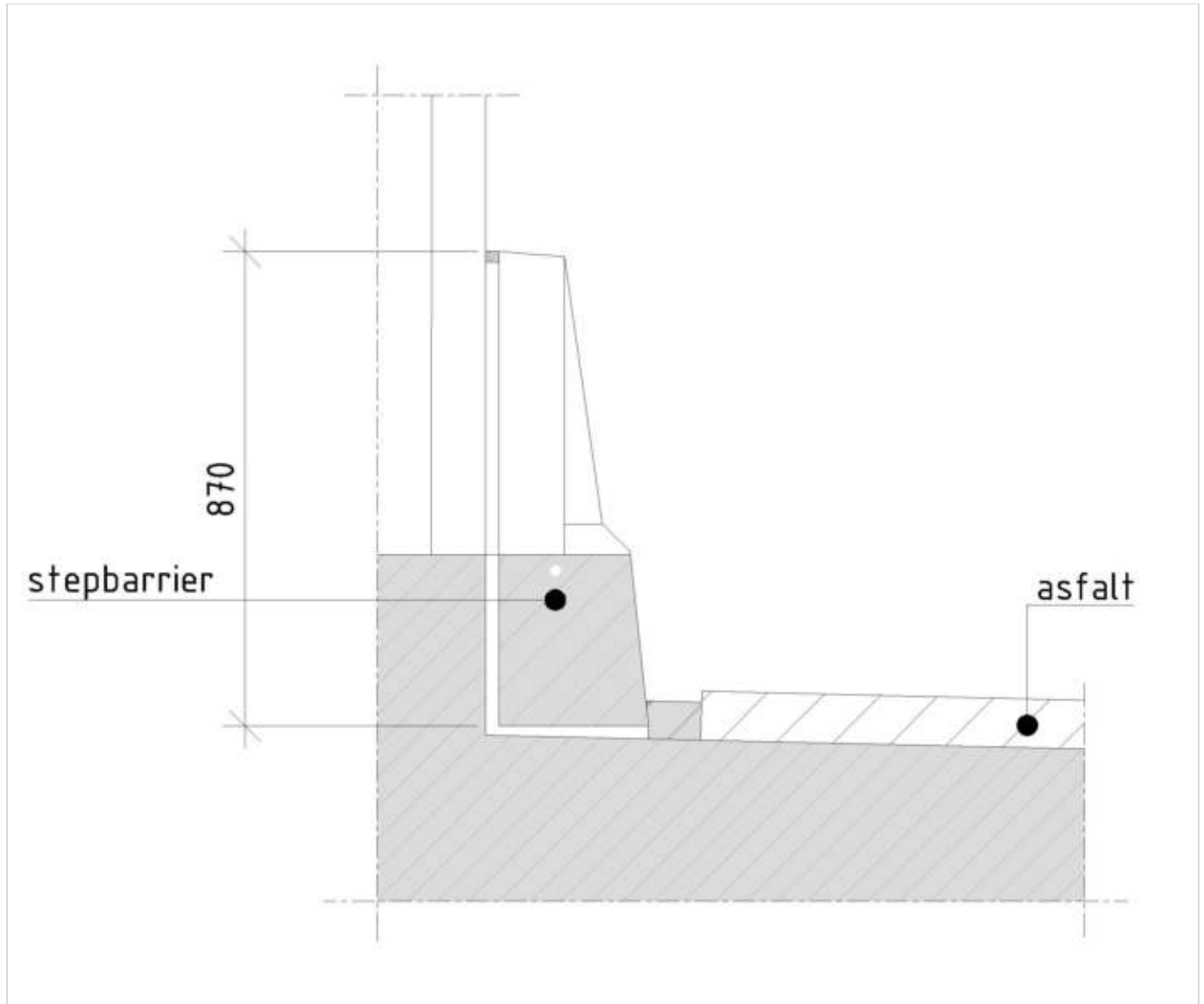
Figuur 455.2 - Doorsnede geleidebarrier t.p.v. vluchtdeur
