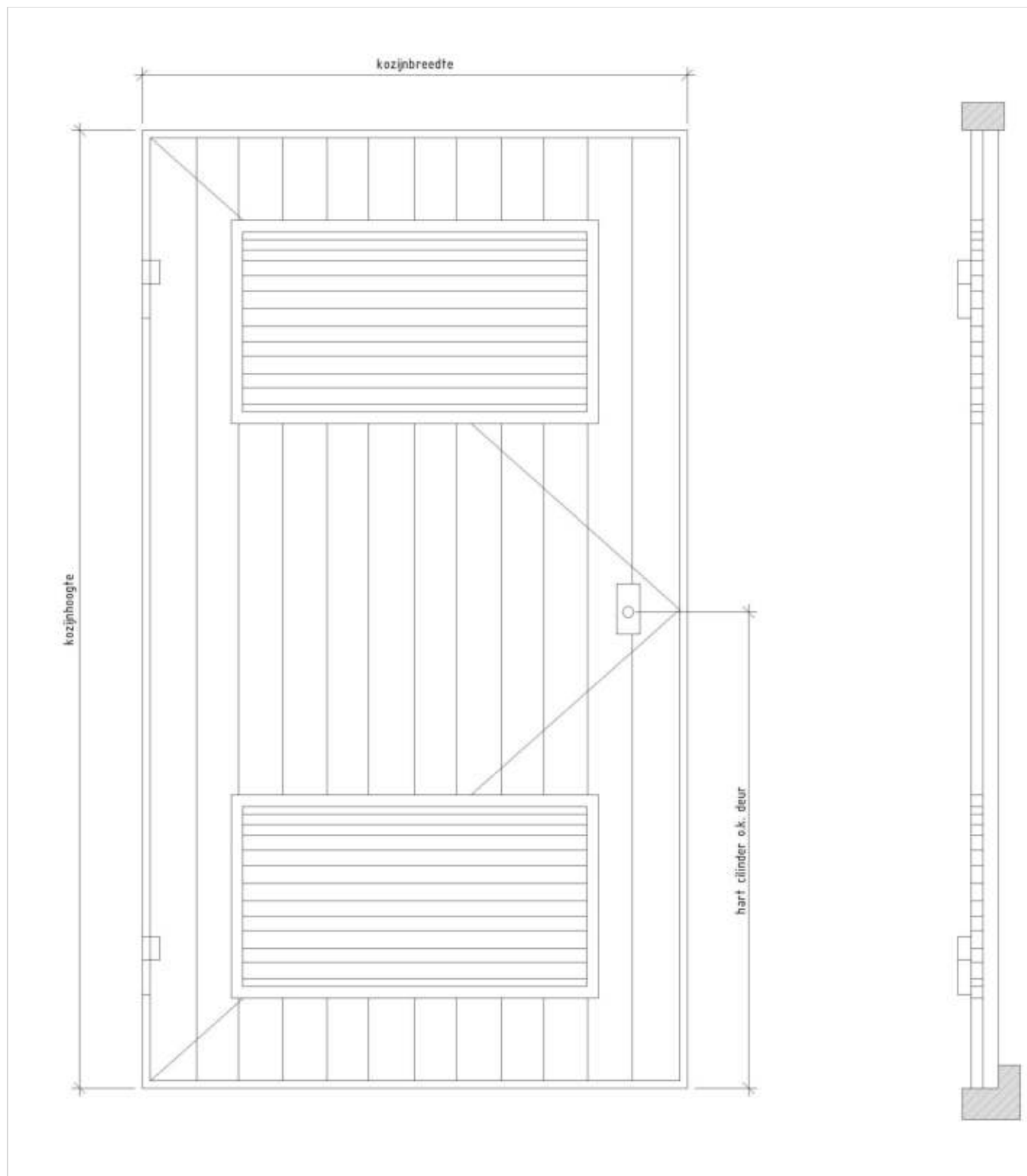
Figuur 439.1 - Trafodeur
