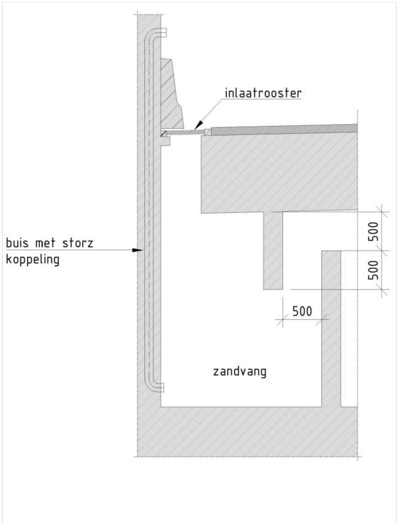
Figuur 410.1 - Zandvang
