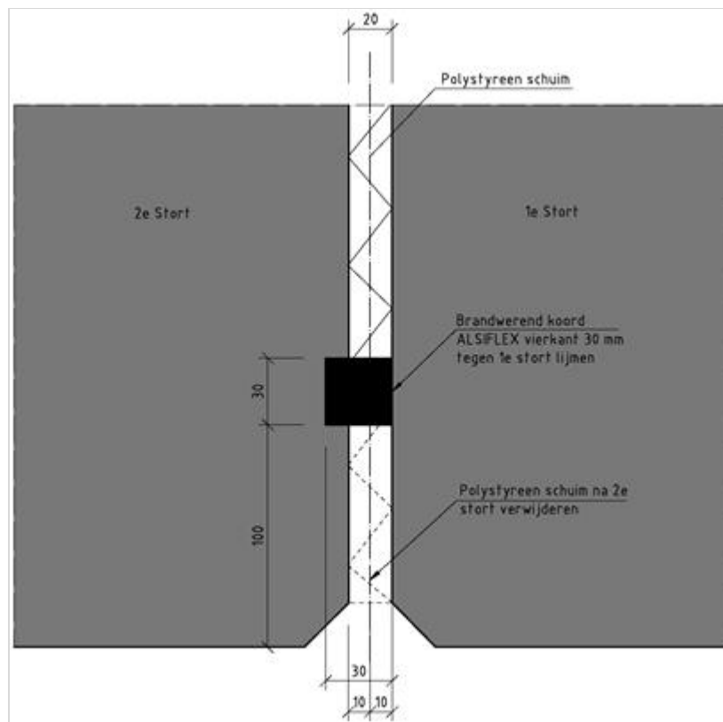
Figuur 267.1 - Brandwerend koord ter bescherming van het rubbermetalen dilatatievoegprofiel. Het aangegeven merk is slechts een voorbeeld. Ook de diepteligging van het koord kan minder zijn dan hier aangegeven.
