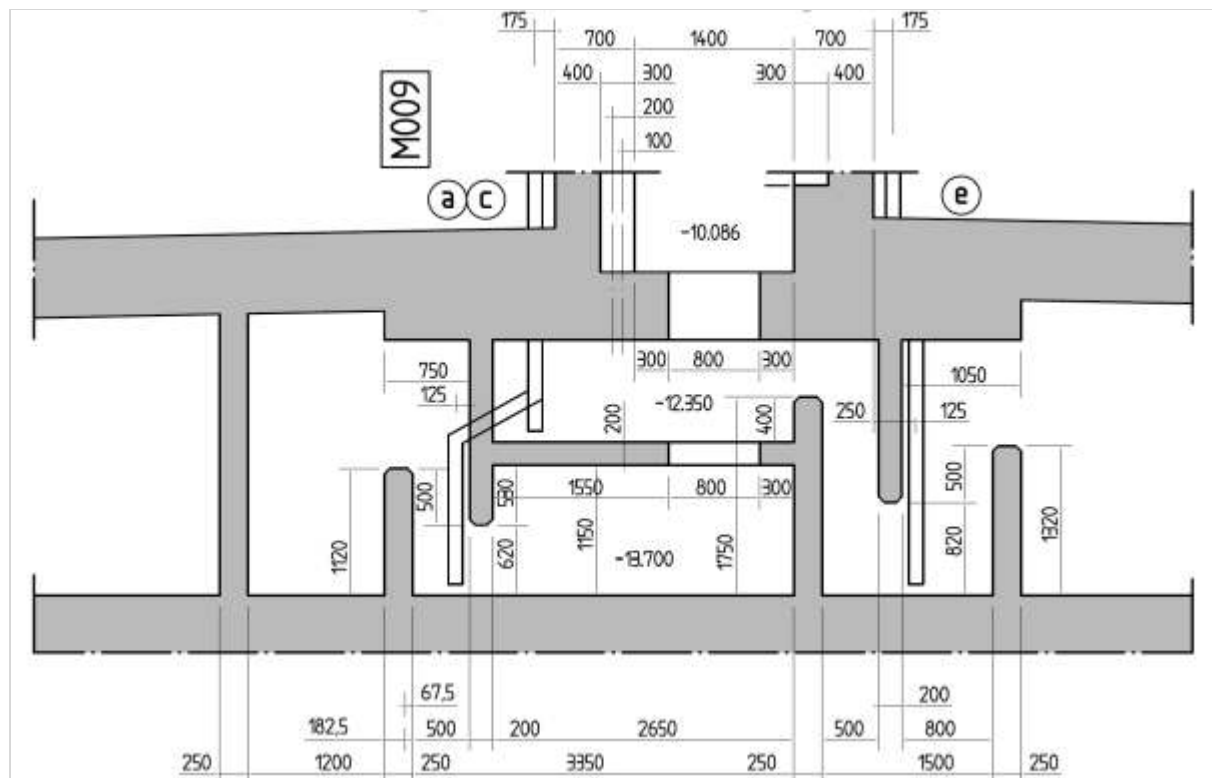
Figuur 412.7 - Verzamelruimte, zandvangen en watersloten
