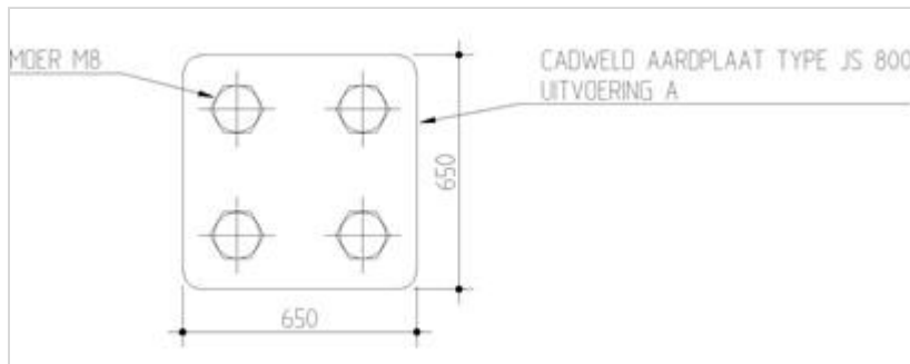
Figuur 288.4 - Detail aardplaat (anker is niet getekend)
