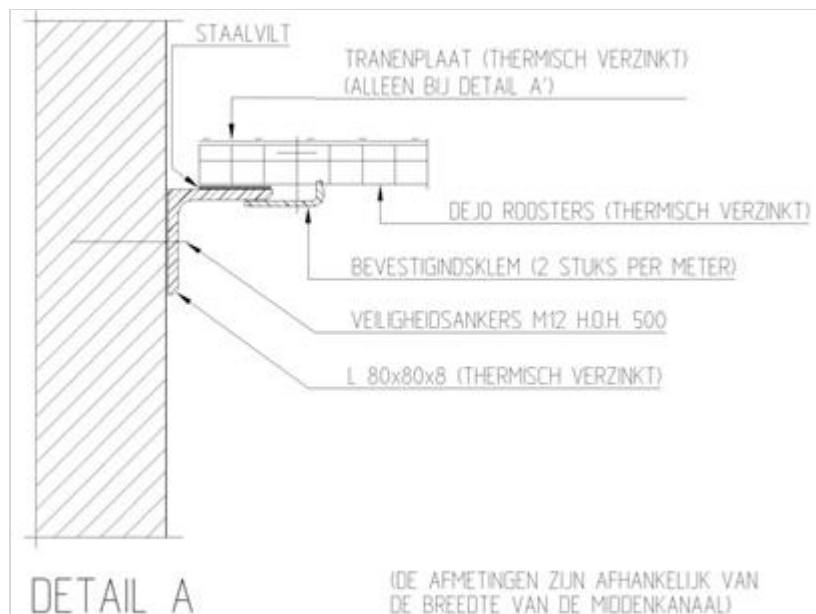
Figuur 468.2 - Roosters middentunnelkanaal
