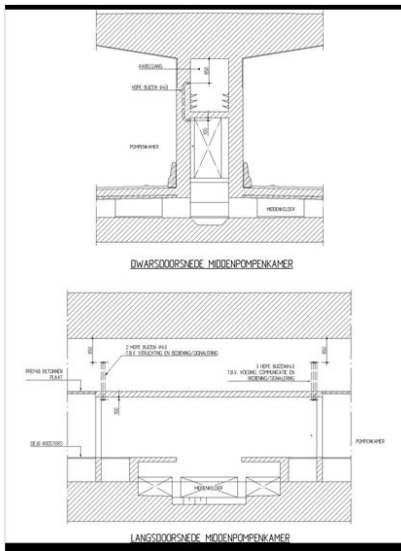
Figuur 299.1 - Dwars- en langsdoorsnede ter plaatse van middenpompkamer
