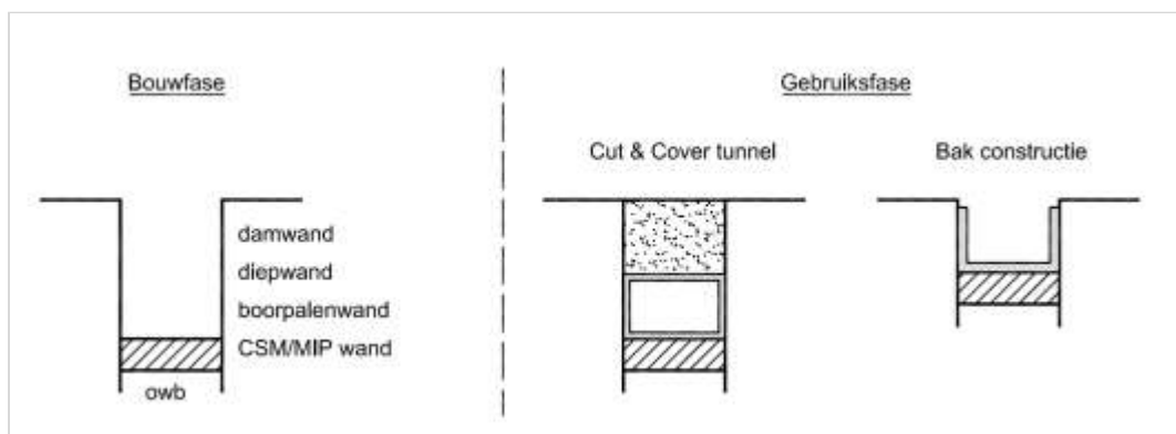
Figuur 46.1 - Bouwkuip met onderwaterbeton (OWB)
