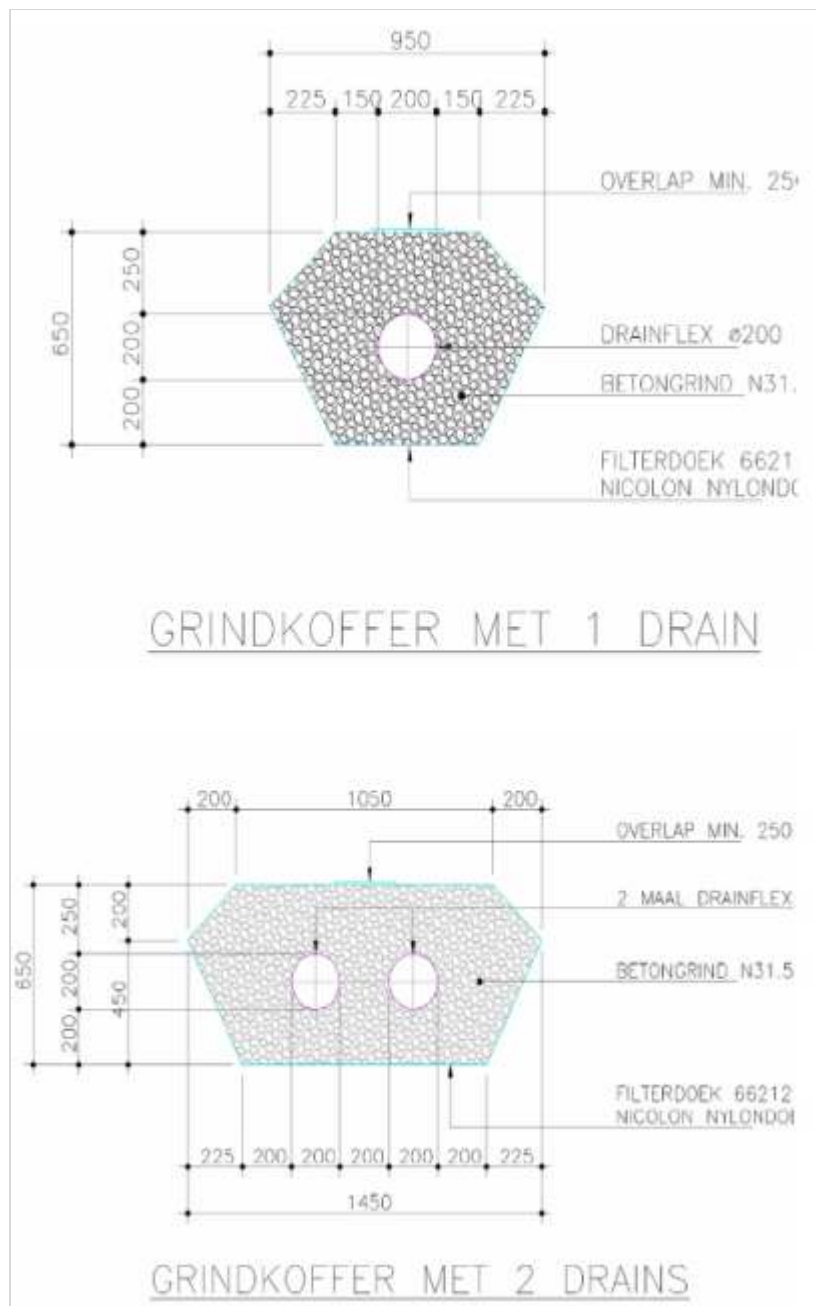
Figuur 394.1 - Drains met grindkoffer
