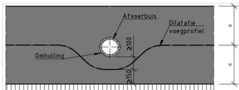
Figuur 251.1 - Dilatatievoegprofiel nabij hemelwaterafvoerbuis in vloer
