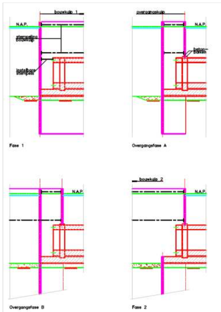
Figuur 213.3 - Fasering betonconstructie in bouwkuip - aansluitdetails variant II
