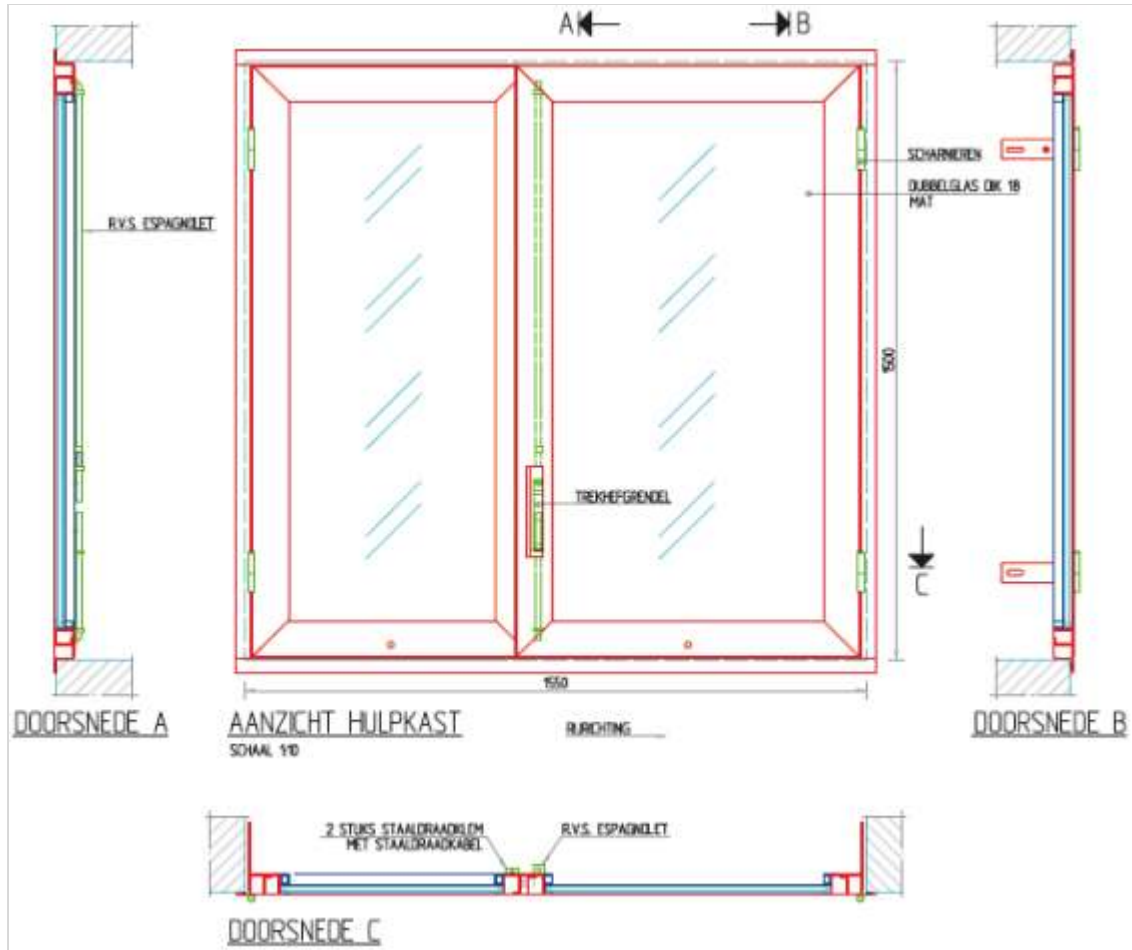
Figuur 461.1 - Kozijn en deuren grote hulppost
