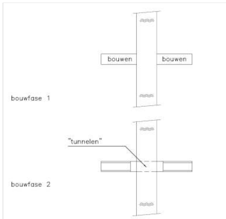
Figuur 210.4 - Principe fasering - variant C
