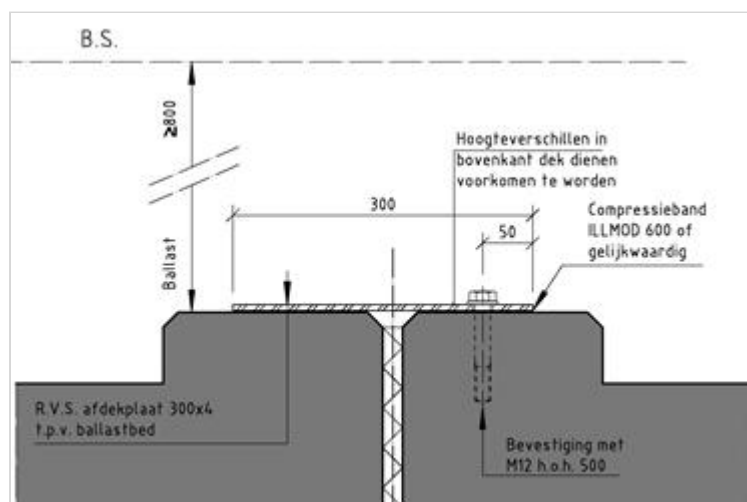
Figuur 266.1 - Voegovergang voor spoor in ballast bij aanwezigheid van hemelwater
