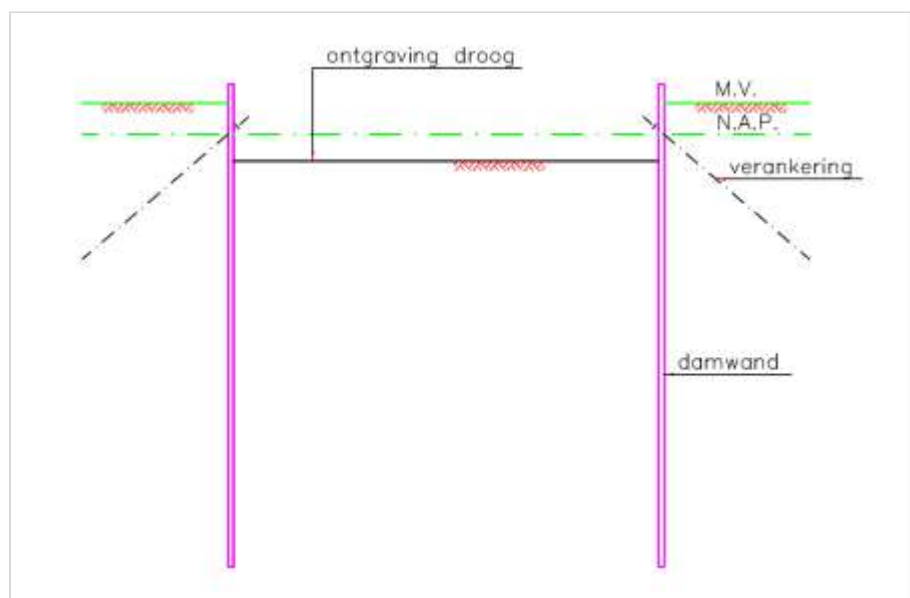
Figuur 177.1 - Bouwkuip met permanente damwanden en onderwaterbeton - fase 1
