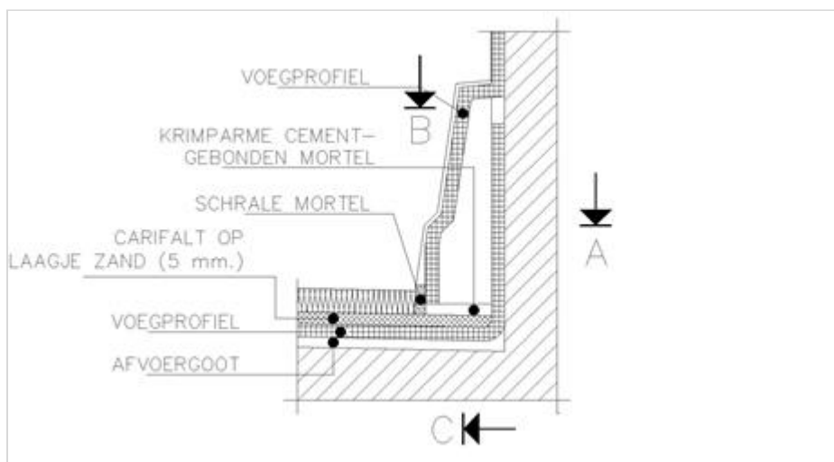
Figuur 258.1 - Aanzicht voegprofiel step barrier buitenwand; aandachtspunt is dat de dilatatievoegen moeten samenvallen met de voegen in de barrier
