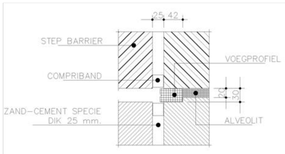
Figuur 258.2 - Voegprofiel step barrier buitenwand doorsnede A
