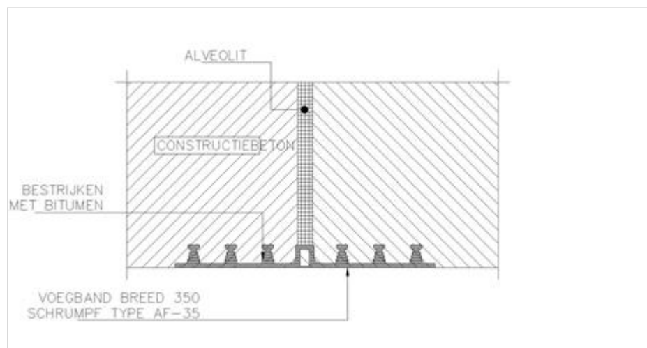
Figuur 262.1 - Detailontwerp onderkant vloer overgangsgedeelte
