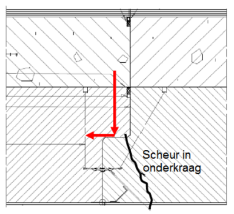
Figuur 84.2 - Gescheurde tandoplegging door verschilzetting
