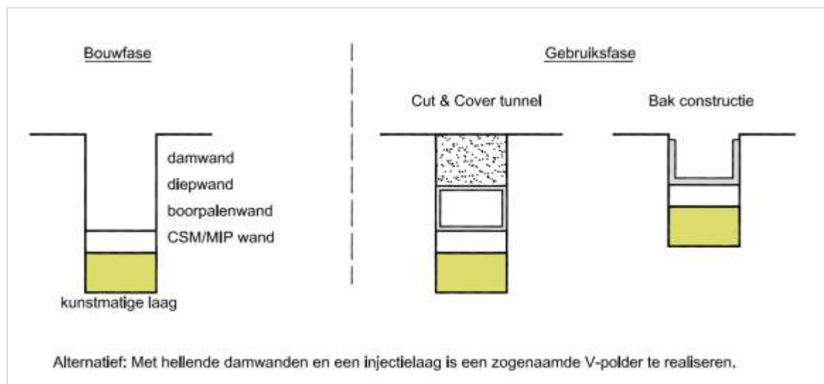
Figuur 46.3 - Bouwkuip met een kunstmatig aangebrachte waterremmende laag
