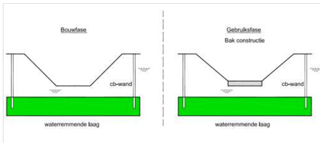
Figuur 46.6 - Polderconstructie met cement-betonietwand (cb-wand)
