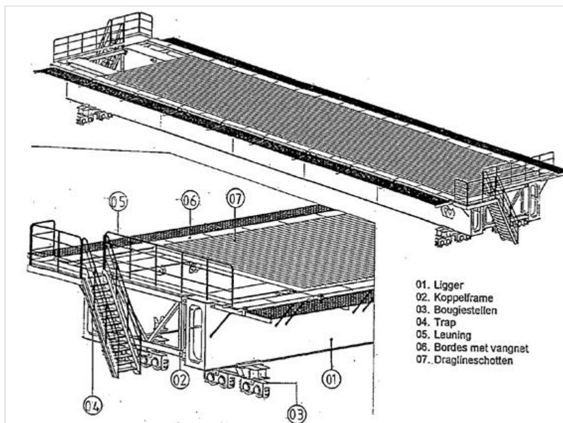
Figuur 624.1 - Voorbeeld traverse
