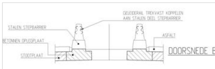
Figuur 459.1 - Aanzichten en details overgang geleidebarrier t.p.v. middenberm
