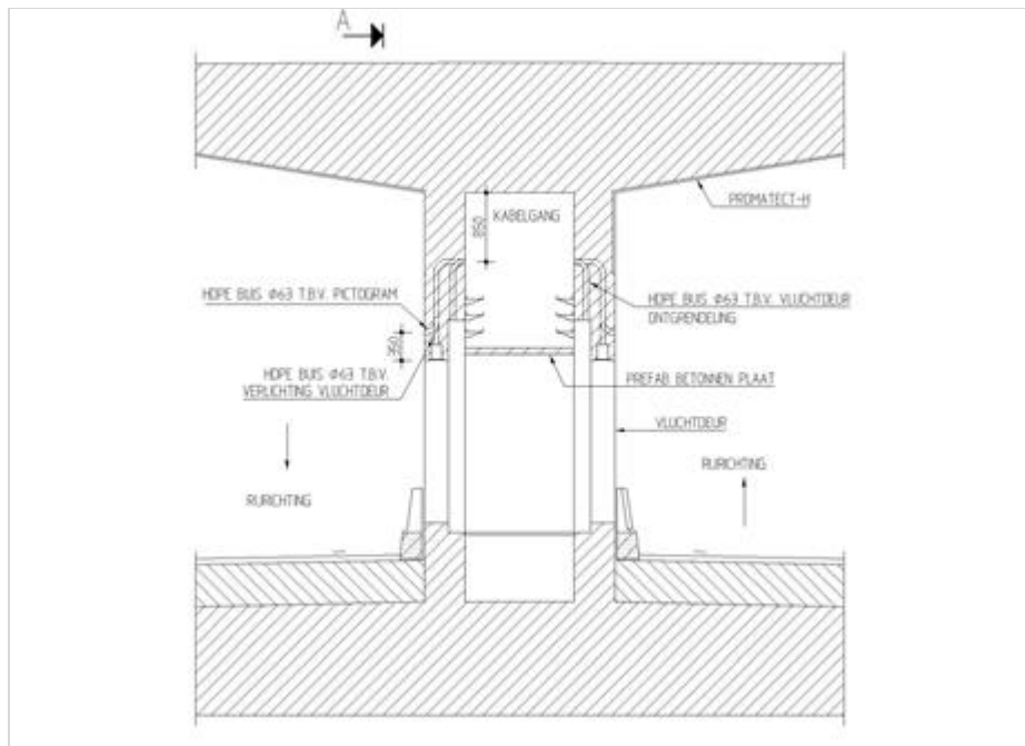
Figuur 282.1 - Doorsnede middenkanaal vluchtdeur (schuifdeur)
