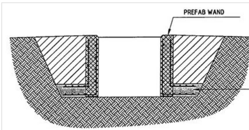
Figuur 554.1 - Voorbeeld geleidewanden
