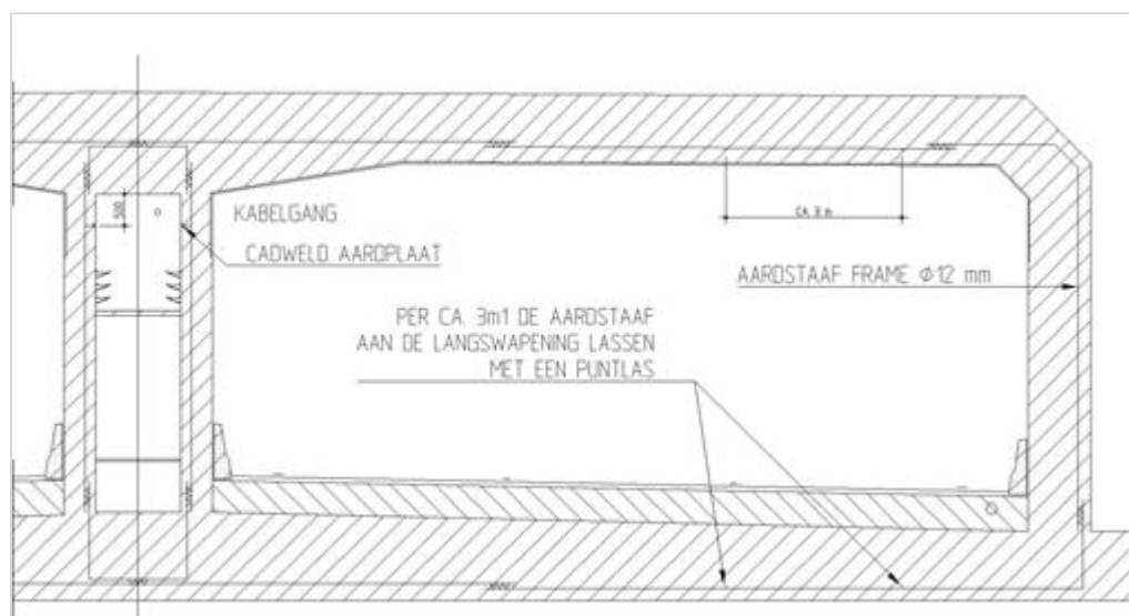
Figuur 288.1 - Doorsnede ssrdstaaf dwarsframe Æ 12 mm
