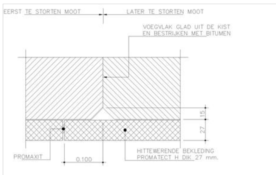
Figuur 268.2 - Detailontwerp hittewerende bekleding methode B
