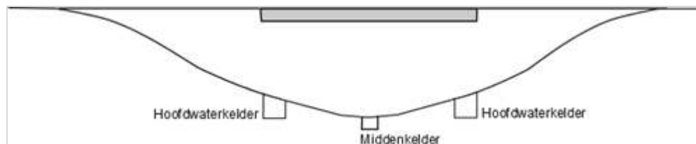
Figuur 382.2 - Lange tunnel met hoofdwaterkelders en middenkelder
