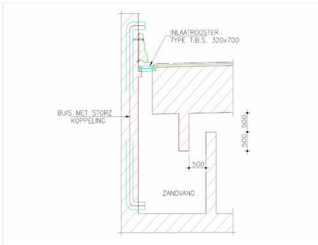
Figuur 410.1 - Zandvang
