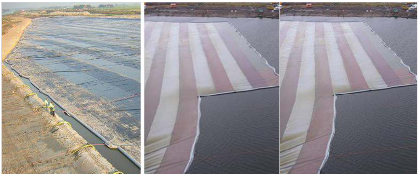
Figuur 193.1 - Afzinken folieconstructie met behulp van drijvers
