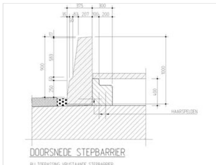
Figuur 452.3 - Doorsnede stepbarrier bij toepassing vrijstaande stepbarrier
