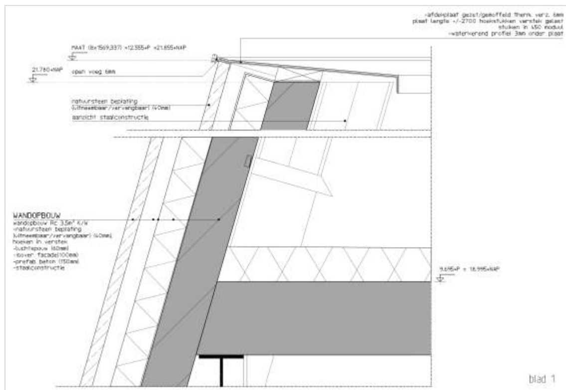
Figuur 441.1 - Gevelaansluiting met dak
