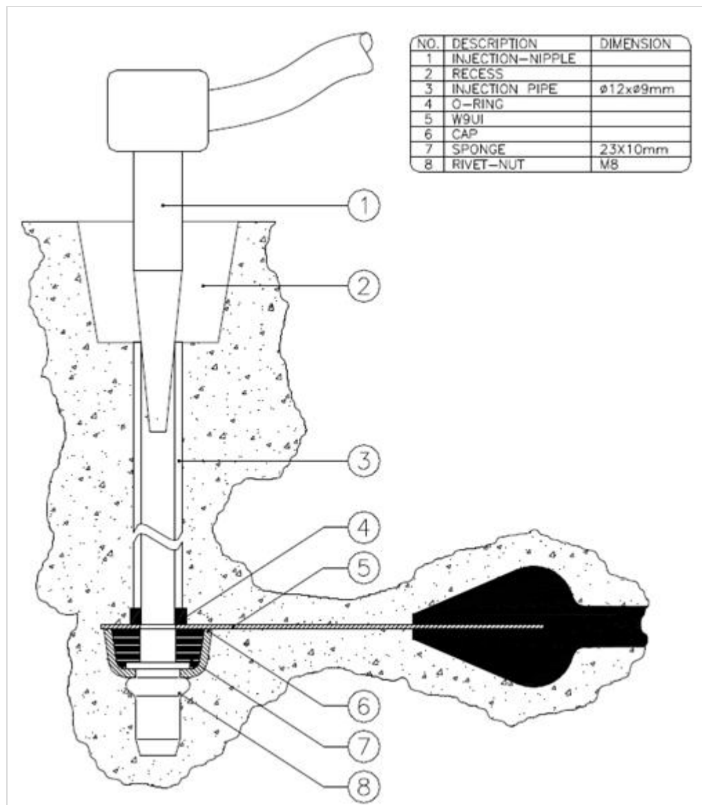
Figuur 248.2 - Voegprofiel met preventie injectiemogelijkheid
