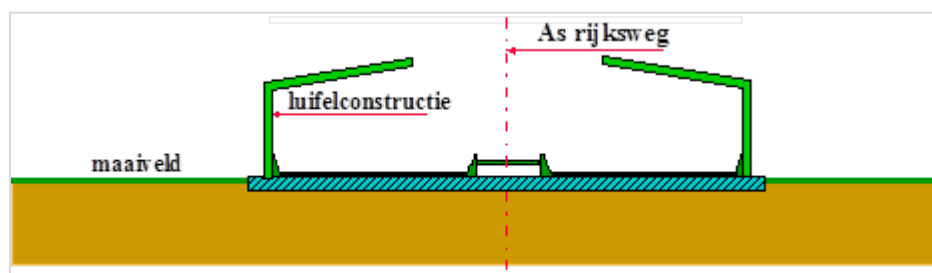
Figuur 9.2 - Doorsnede luifelconstructie
