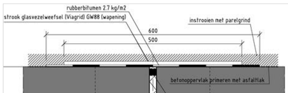
Figuur 265.2 - Voegovergang voor asfalt
