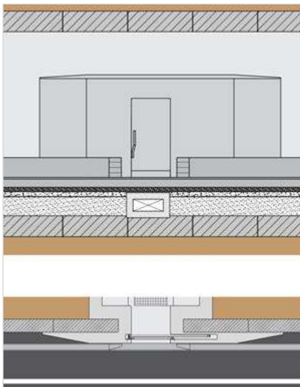
Figuur 379.1 - Halve barrier tegen tunnelwand bij nooduitgang
