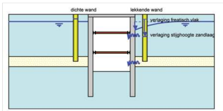
Figuur 139.1 - Grondwaterdaling door lekkage bouwkuipwand
