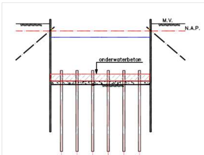
Figuur 172.4 - Bouwkuip met damwanden, onderwaterbeton (OWB) en trekpalen - fase 4
