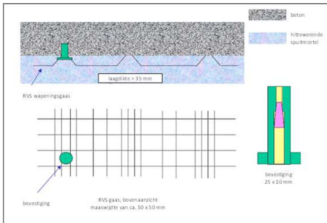
Figuur 316.1 - Passieve inwendige hittewerende maatregelen
