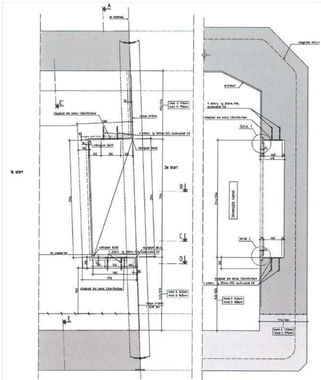
Figuur 370.5 - Aanzicht en doorsnede tandconstructie buitenwand 2e Coentunnel t.p.v. mootvoeg; 'vrouwtje'
