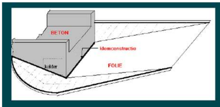
Figuur 228.5 - Aansluiting folie op betonconstructie
