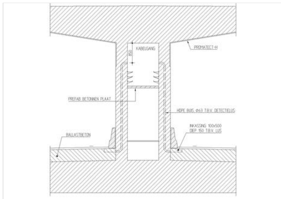
Figuur 284.1 - Doorsnede middenkanaal met mantelbuis voor detectielussen wegdek
