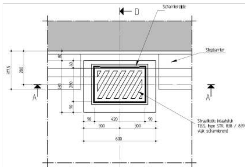
Figuur 412.2 - Inlaatput
