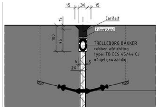
Figuur 265.1 - Voorbeeld afdichting ten behoeve van calamiteitendichting (gevaarlijke stoffen)
