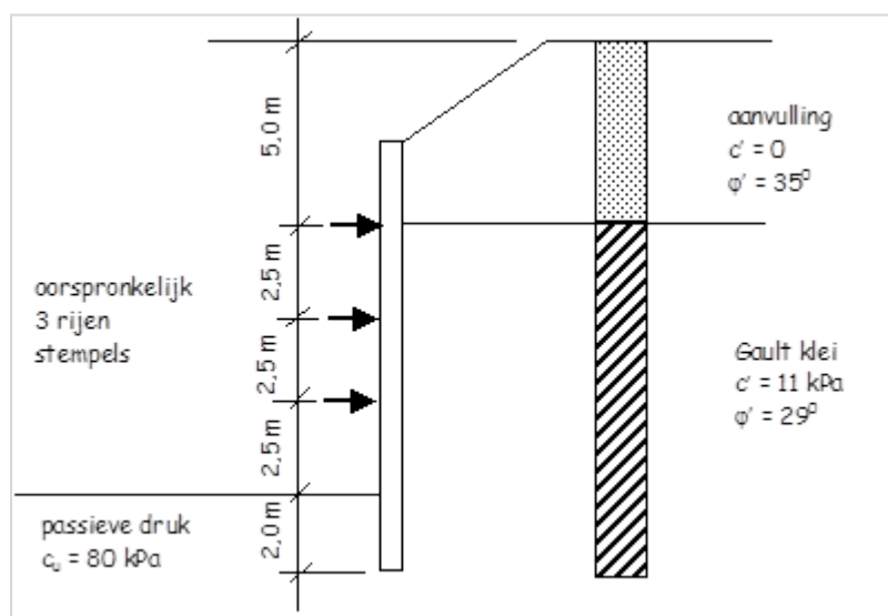
Figuur 159.1 - Toepassing observatiemethode bij ontwerp gestempelde bouwputwand (Kanaaltunnel, zie [7])
