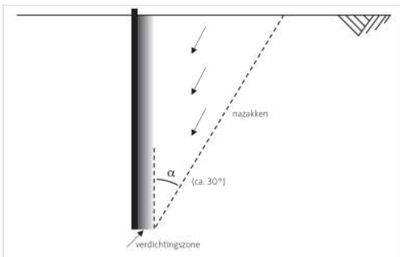
Figuur 151.1 - Vertaling lokale verdichting naar maaiveldzinking
