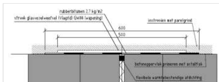
Figuur 471.1 - Detail voegafdekking
