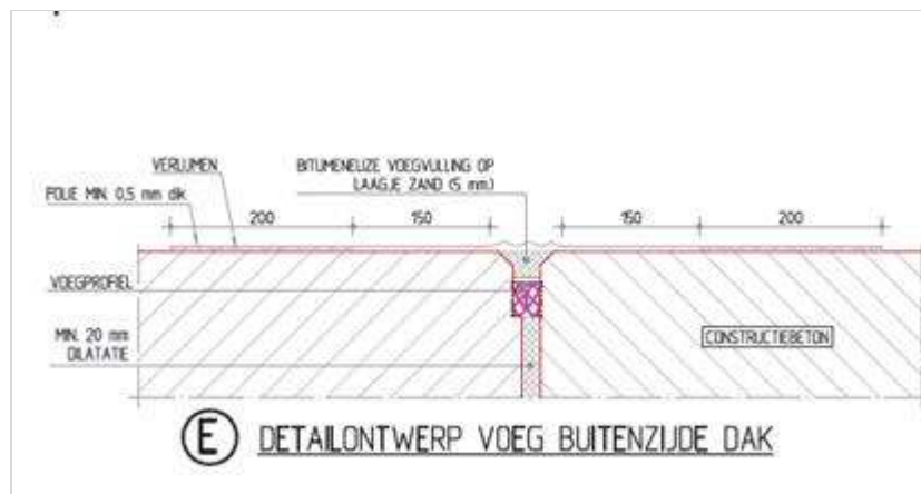
Figuur 257.1 - Voeg buitenzijde dak
