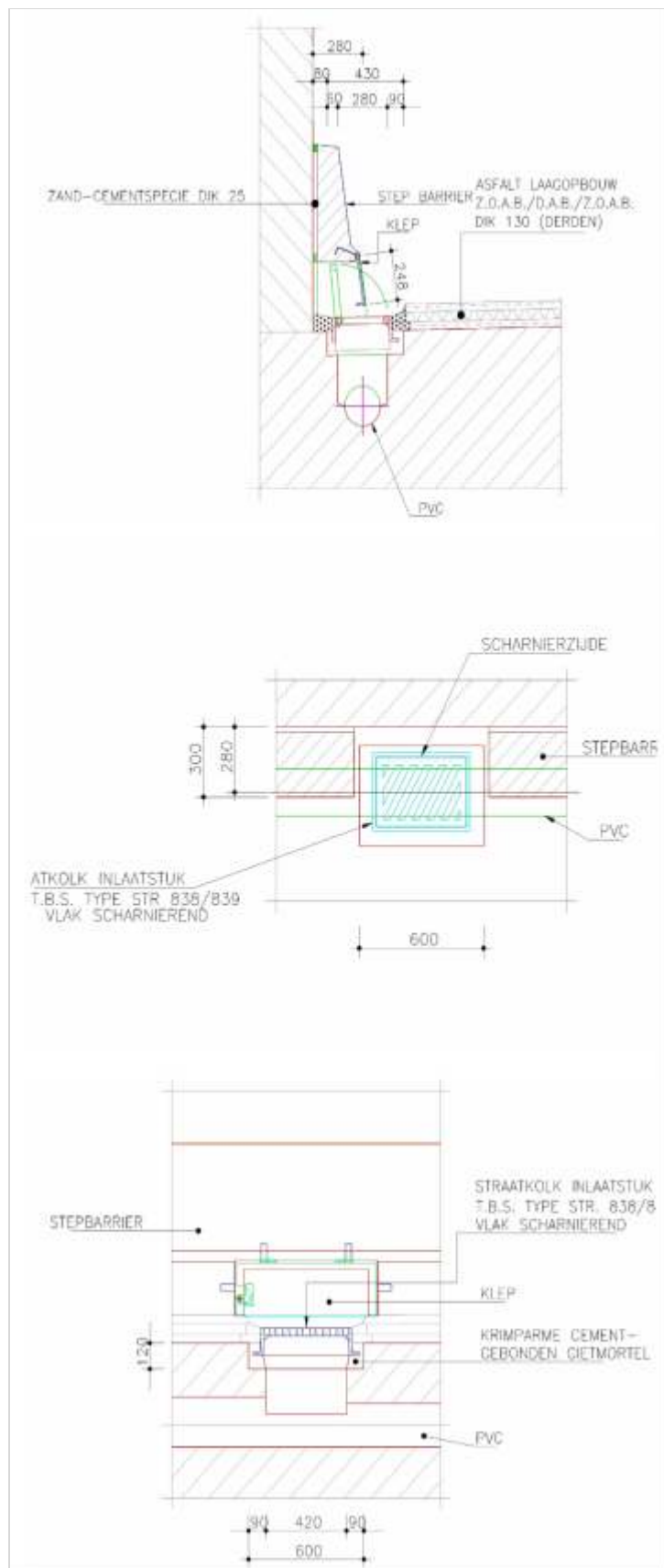
Figuur 388.1 - Inlaatputten bij toepassing ZOAB
