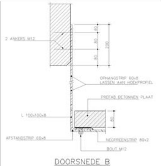
Figuur 468.1 - Aanzicht en details plaat in middenkanaal
