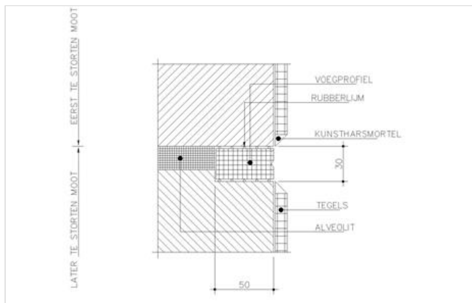
Figuur 264.1 - Detailontwerp tegelwerk - toepassing kunstharsmortel
