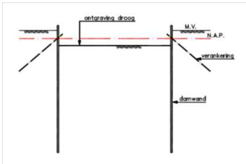
Figuur 172.1 - Bouwkuip met damwanden, onderwaterbeton (OWB) en trekpalen - fase 1
