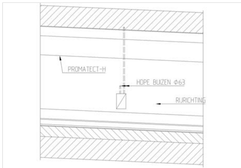
Figuur 281.2 - Aanzicht buitenwand van 4-46
