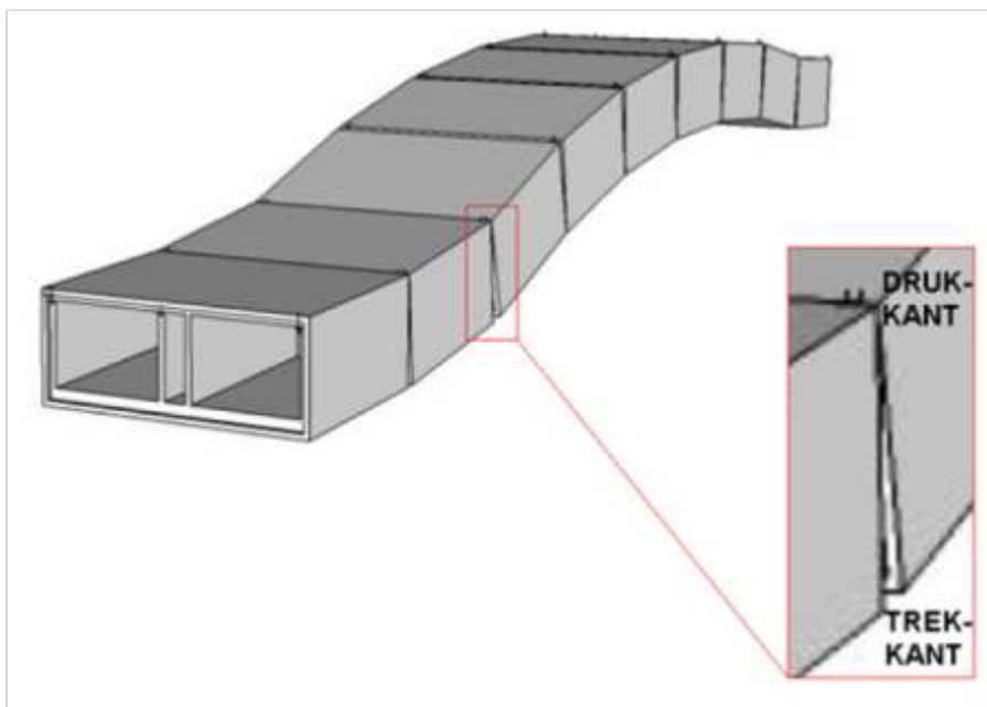
Figuur 85.1 - Rotatie van moten
