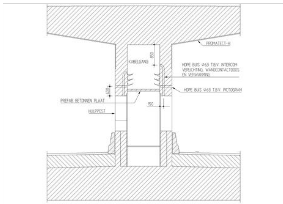
Figuur 280.1 - Doorsnede middenkanaal hulppost type A
