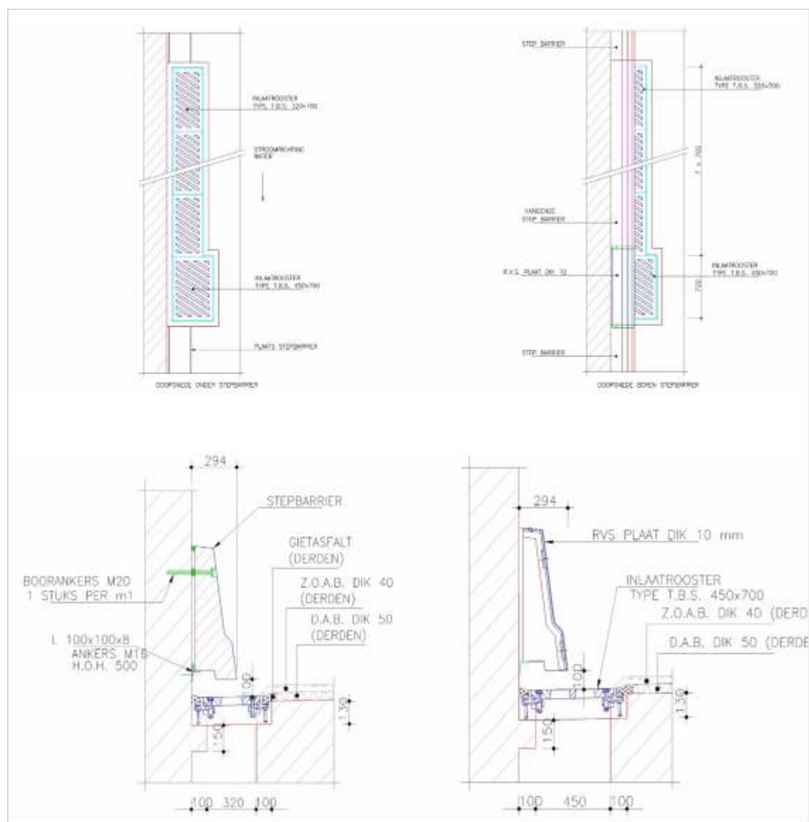
Figuur 409.1 - Inlaatrooster hoofdwaterkelder bij toepassing ZOAB
