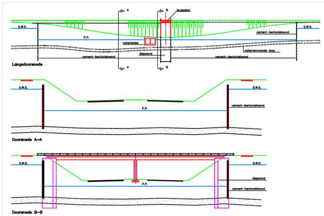
Figuur 201.1 - Kunstmatige polder met cement-bentoniet wand (voorbeeld)
