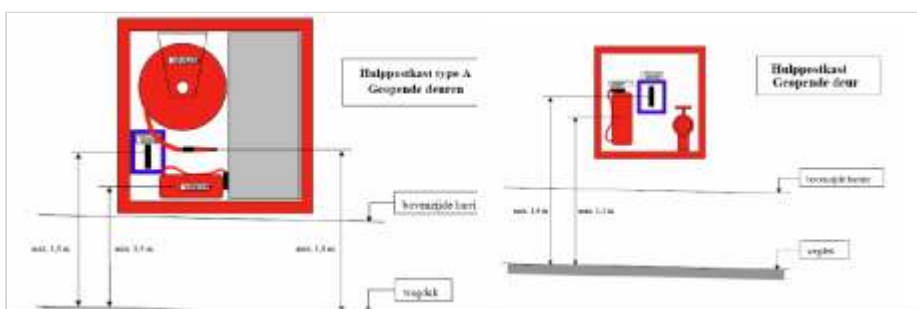
Figuur 278.1 - Voorbeelden van hulpposten
