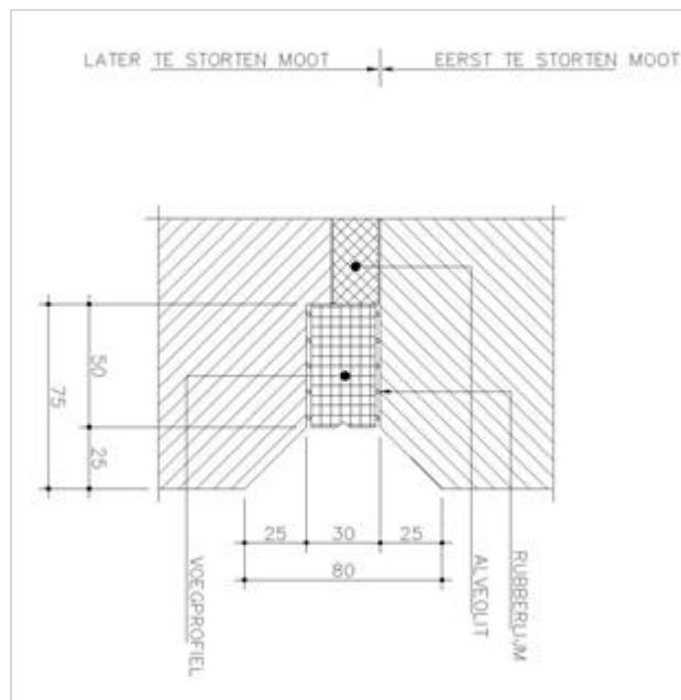
Figuur 263.1 - Detailontwerp voegprofiel
