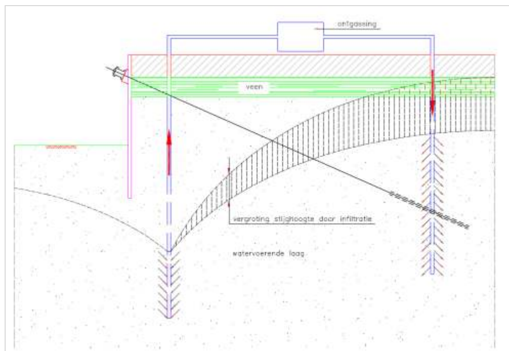
Figuur 166.5 - Retourbemaling
