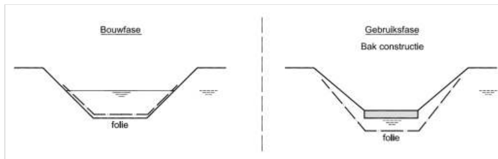
Figuur 46.5 - Polderconstructie met taluds en folie (schematische weergave)
