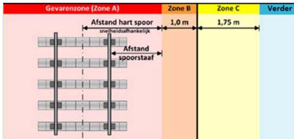
Figuur 515.1 - Zoneverdeling spoor
