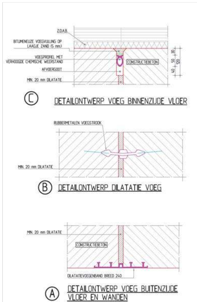
Figuur 246.1 - Detailontwerp voeg vloeren.
