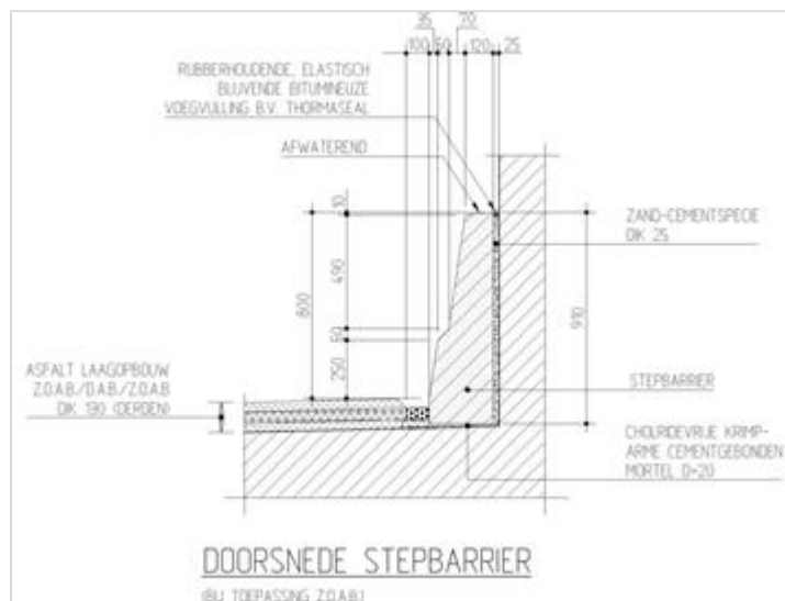
Figuur 452.2 - Doorsnede Stepbarrier bij toepassing ZOAB
