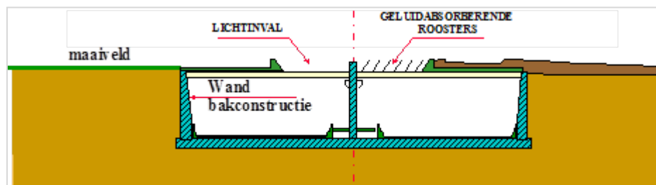
Figuur 9.1 - Doorsnede overkapte bakconstructie
