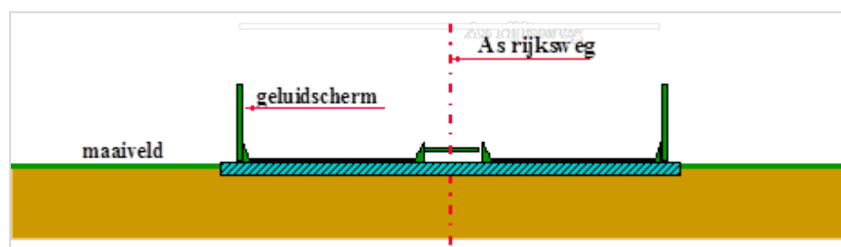
Figuur 10.3 - Weg voorzien van geluidsschermen (valt buiten de scope van dit handboek)
