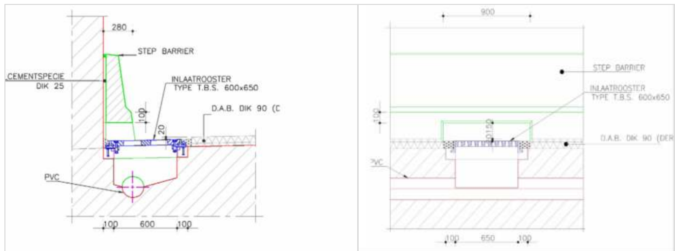
Figuur 387.2 - Inlaatputten (bij toepassing DAB)
