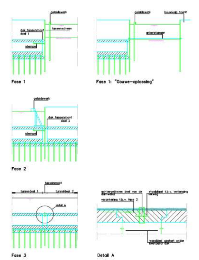
Figuur 213.2 - Fasering betonconstructie in bouwkuip - aansluitdetails variant I
