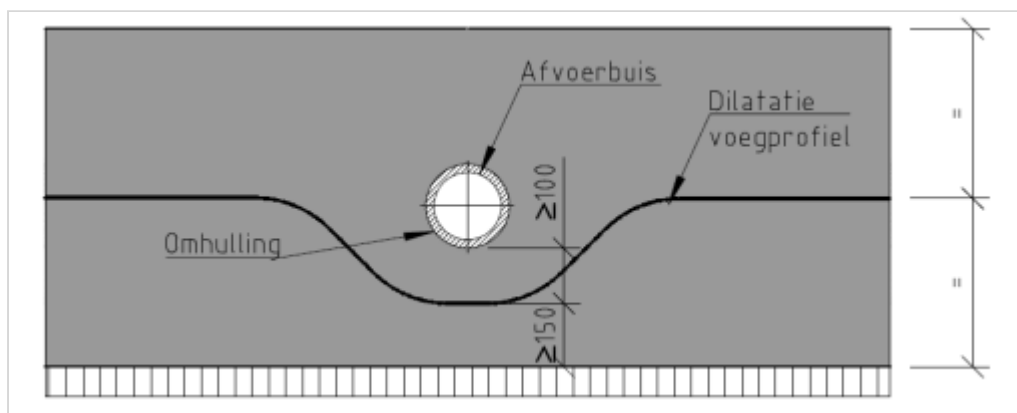
Figuur 502.2 - Principe aanzicht afvoerbuĳs t.p.v. voegovergang
