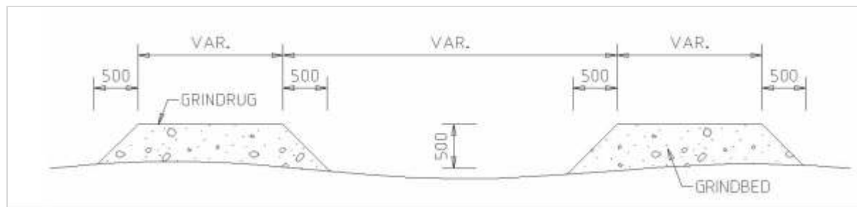
Figuur 242.1 - Fundering afgezonken tunnel op grindruggen
