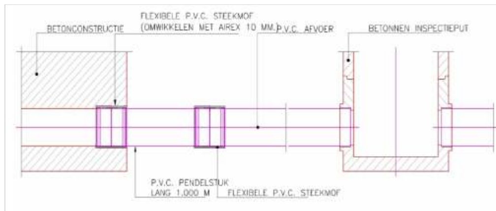
Figuur 391.1 - Aansluiting inspectieput-betonconstructie
