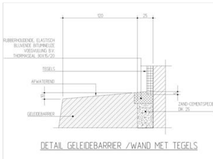
Figuur 454.2 - Detail geleidebarrier/wand met tegels
