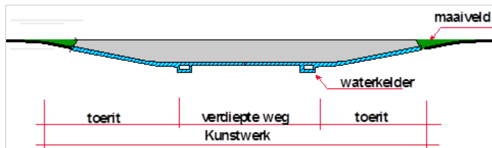
Figuur 10.1 - Verdiepte weg - langsdoorsnede
