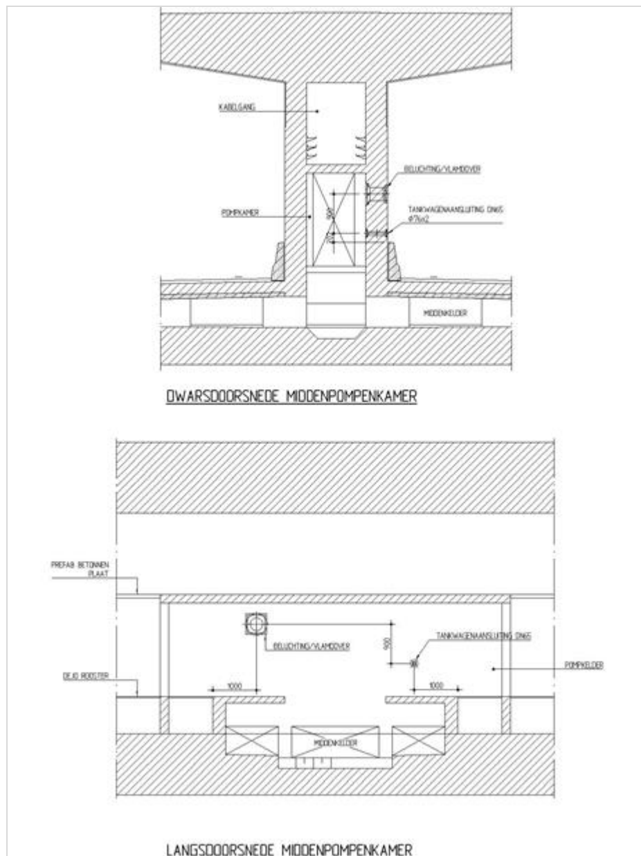
Figuur 302.1 - Dwars- en langsdoorsnede middenpompkamer - vlamdover en tankwagenaansluiting
