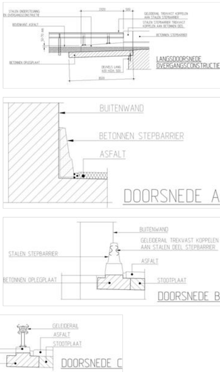
Figuur 458.1 - Aanzichten en details overgang geleidebarrier t.p.v. buitenwand
