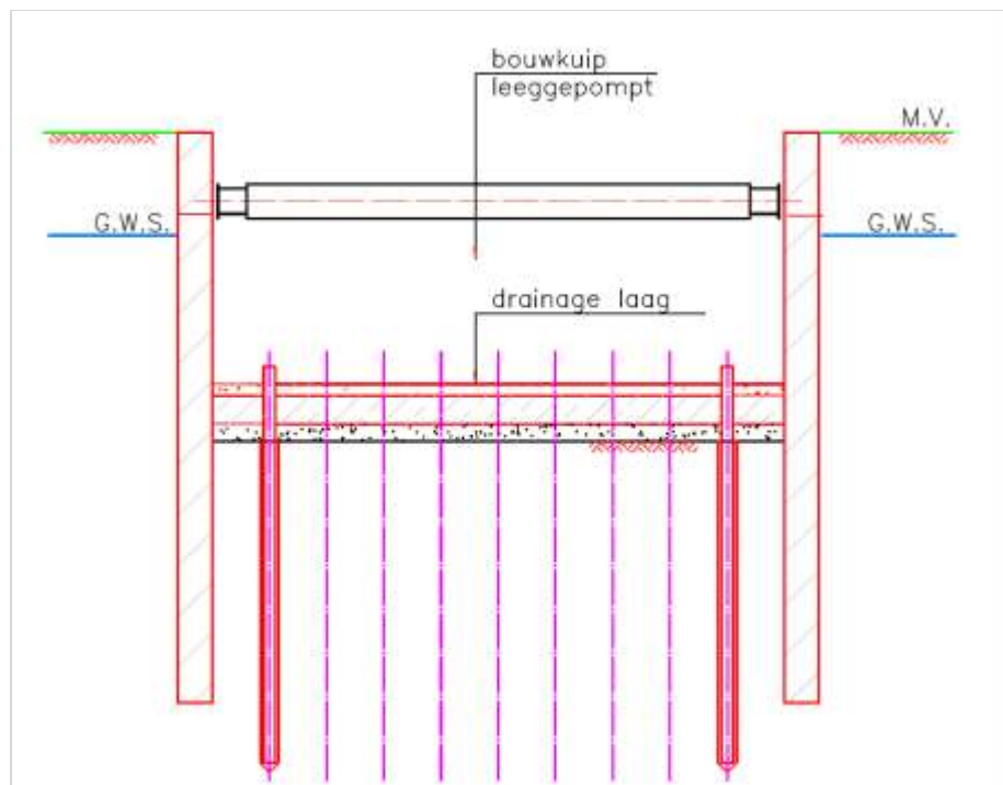
Figuur 181.4 - Bouwkuip met diepwanden en onderwaterbeton - fase 5
