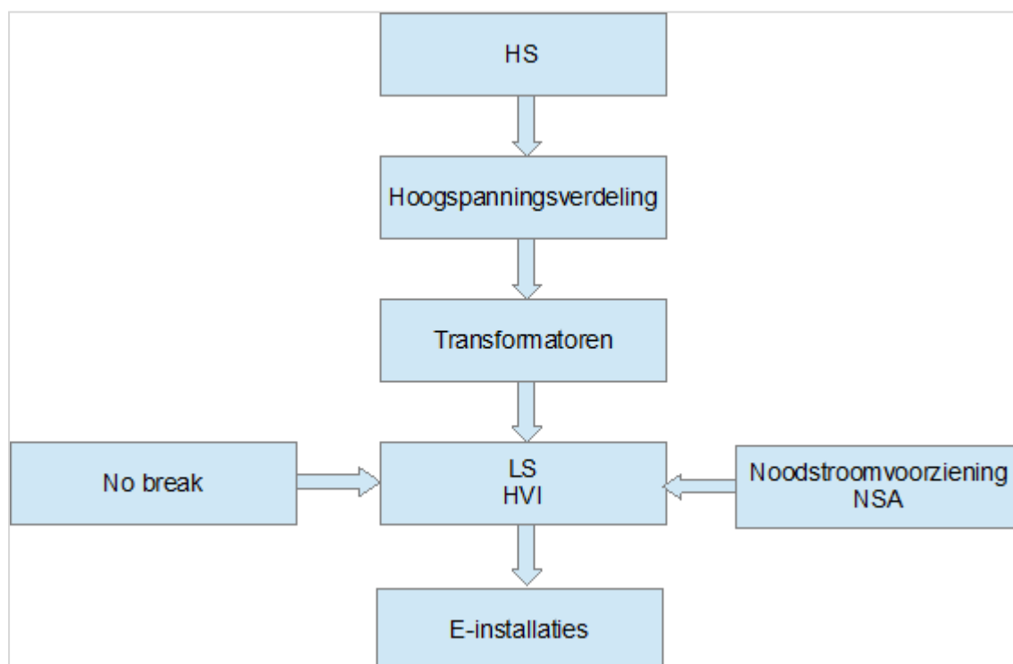
Figuur 417.1 - Verloop van de elektrische energie.
