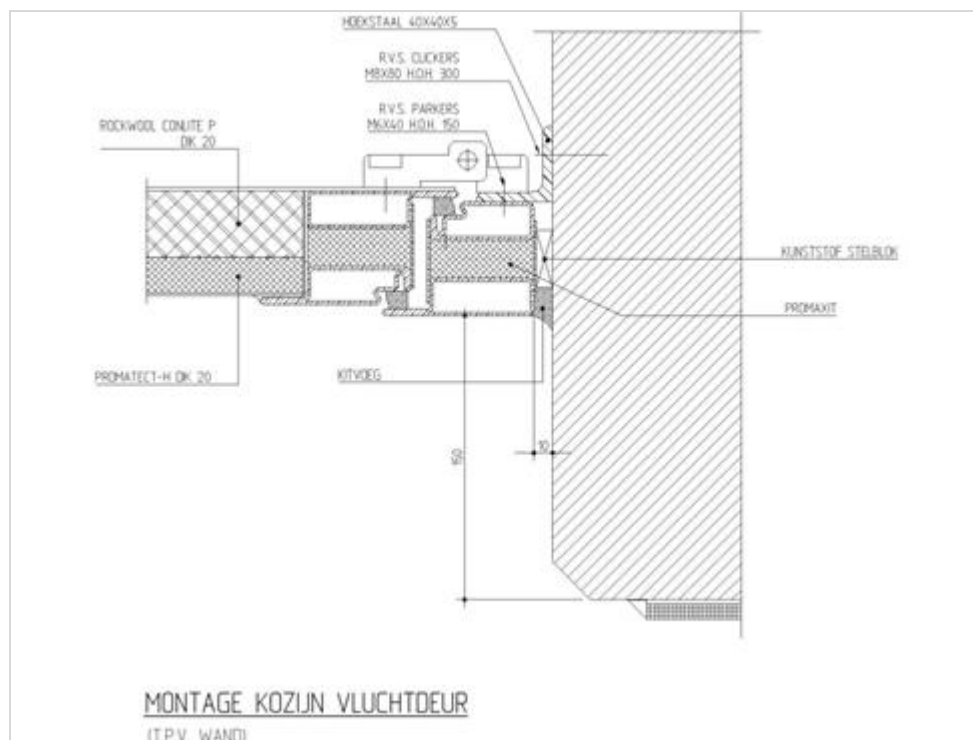
Figuur 491.1 - Detail montage kozijn vluchtdeur (draaideur)
