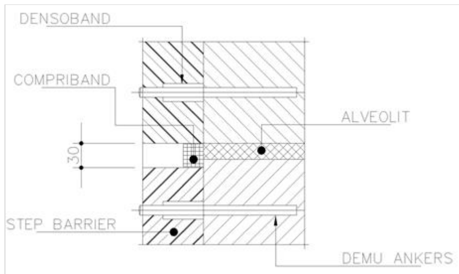
Figuur 259.2 - Voegprofiel step barrier middenberm doorsnede A
