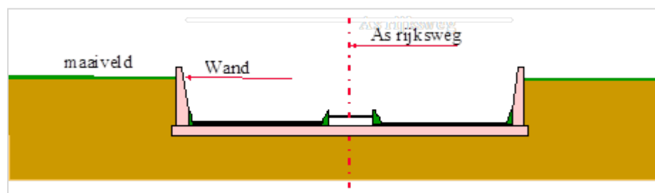
Figuur 10.2 - Verdiepte weg - dwarsdoorsnede
