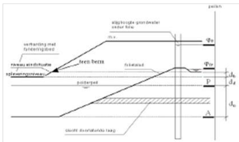
Figuur 234.1 - verticaal evenwicht
