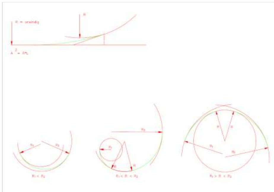
Figuur 19.1 - Clothoïde
