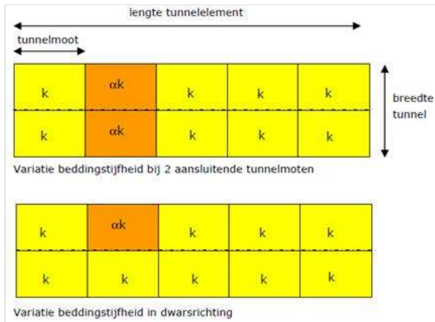
Figuur 100.2 - Aan te houden variaties in beddingstijfheid
