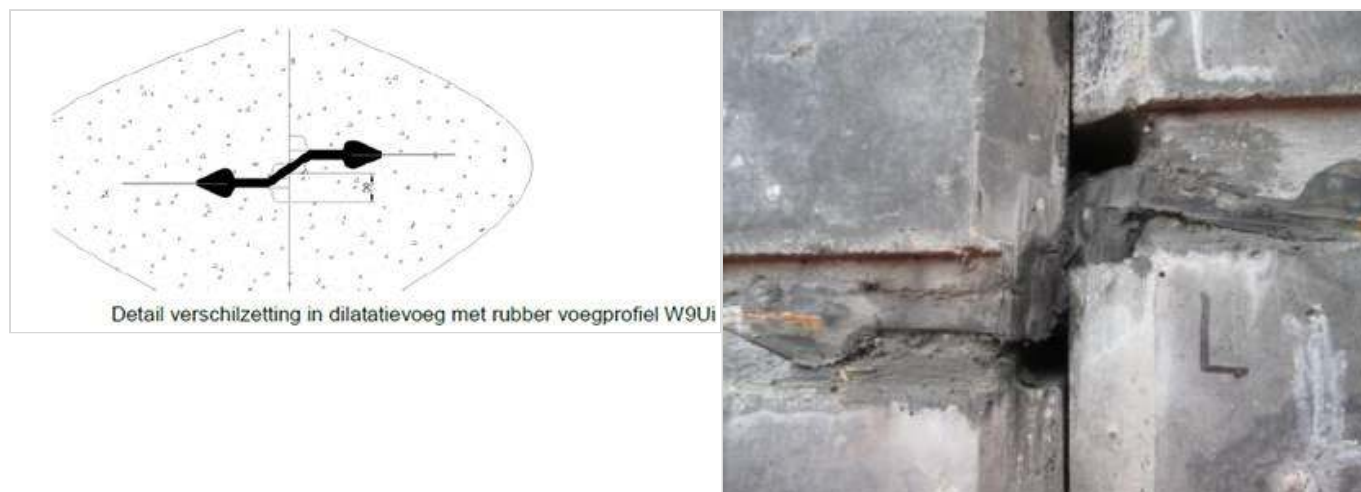
Figuur 369.1 - Beschadiging waterkerend profiel als gevolg van verschilverplaatsing bij zeer geringe voegbreedte
