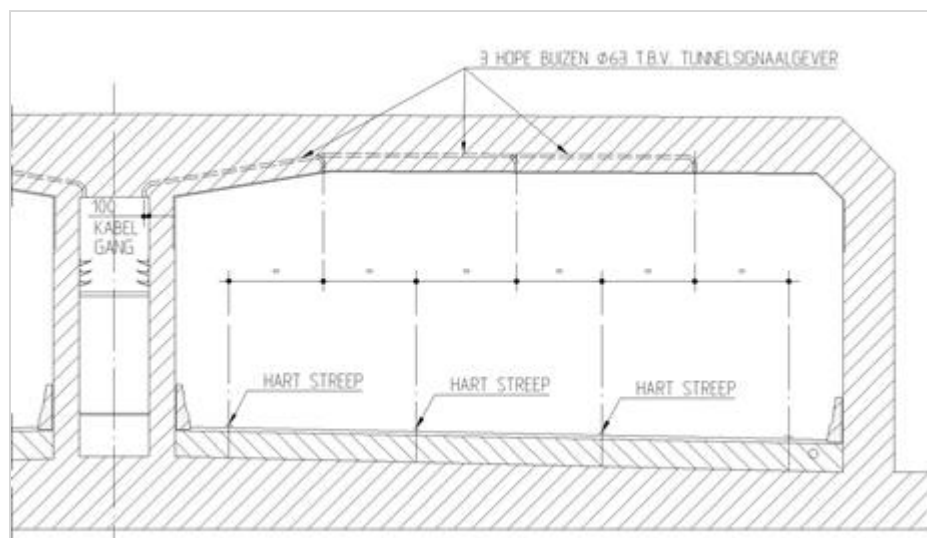
Figuur 293.1 - Doorsnede tunnel ter plaatse van matrixsignaalgever (dak)
