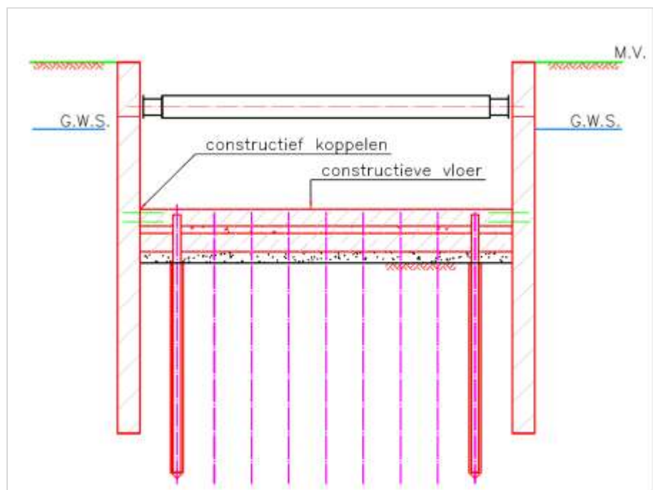
Figuur 181.5 - Bouwkuip met diepwanden en onderwaterbeton - fase 6
