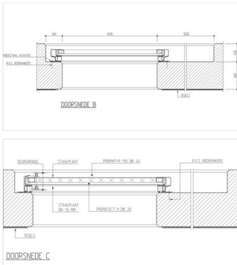
Figuur 490.1 - Kozijn en deur vluchtdeur (schuifdeur)
