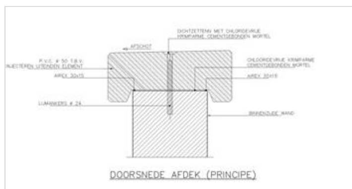
Figuur 467.1 - Principe doorsnede afdekband
