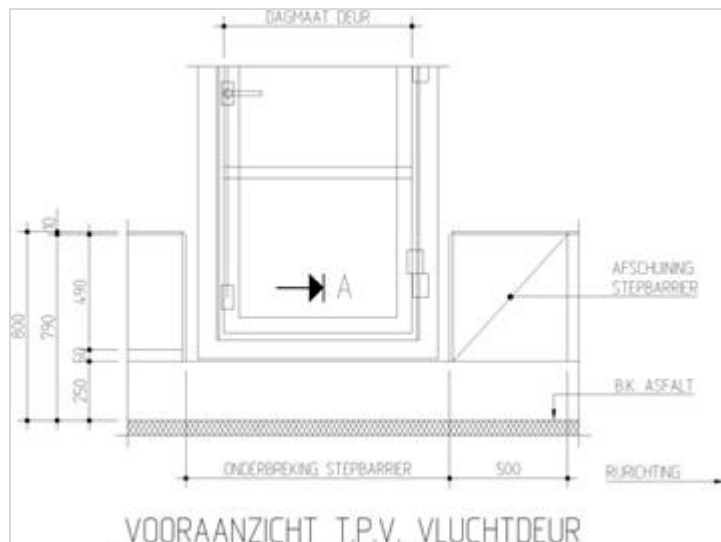
Figuur 455.1 - Vooraanzicht geleidebarrier t.p.v. vluchtdeur (plaatje voldoet niet aan Rarvw)
