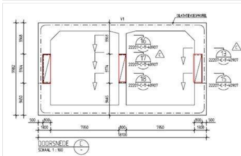
Figuur 370.1 - Tandconstructies tussen de mootvoegen in de wanden van de HSL tunnel onder de Oude Maas.
