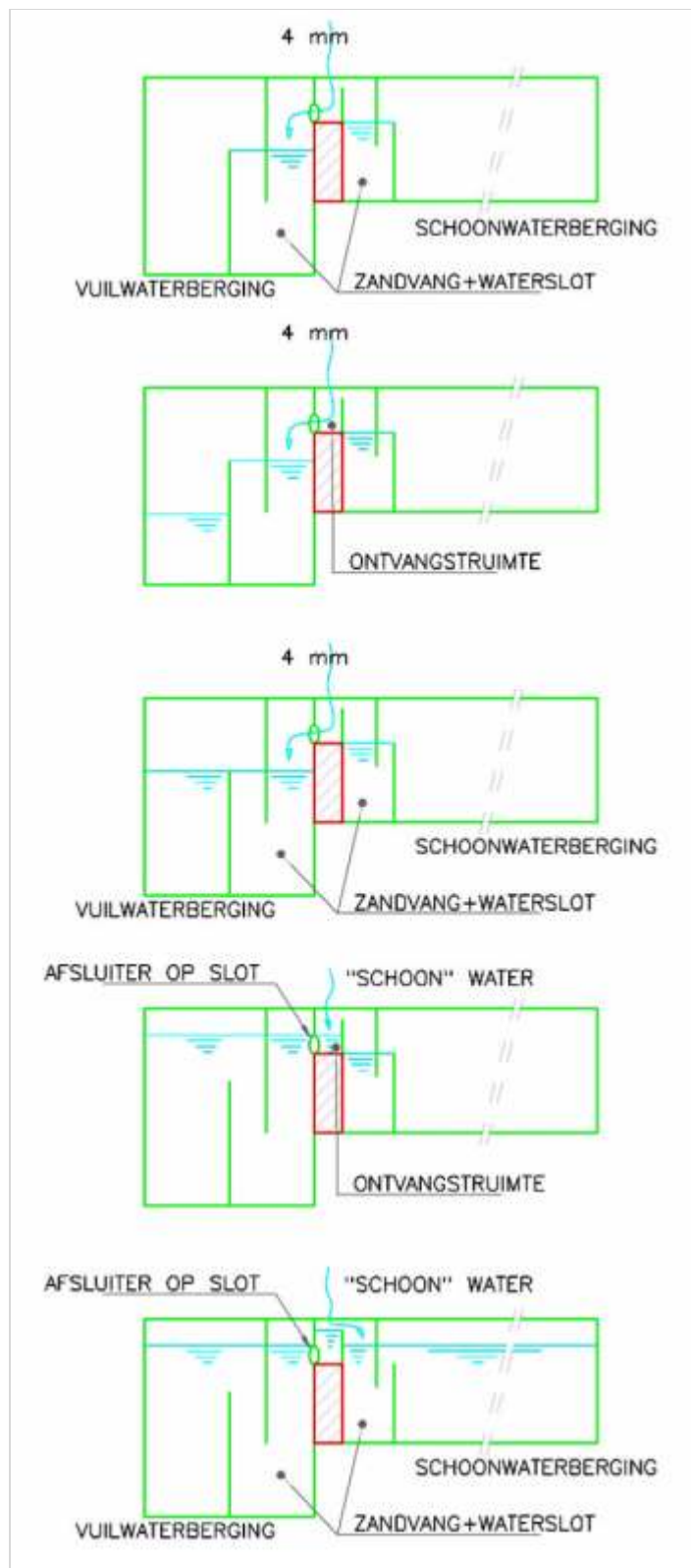
Figuur 406.1 - Principe-indeling hoofdwatertank met verbeterd gescheiden systeem
