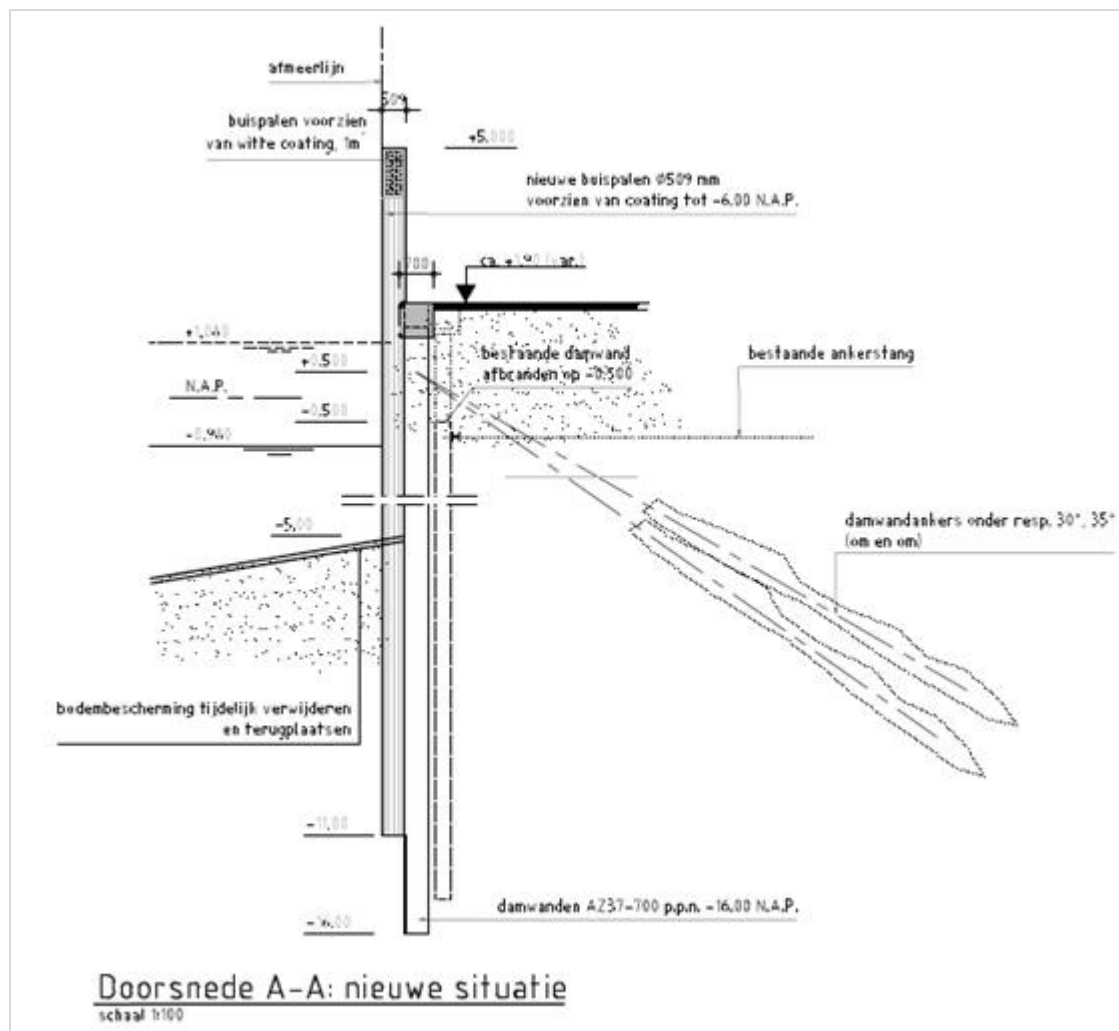
Figuur 138.1 - Voorbeeld van het rehabiliteren van een oude door corrosie verzwakte damwand (kadeconstructie Harlingen)
