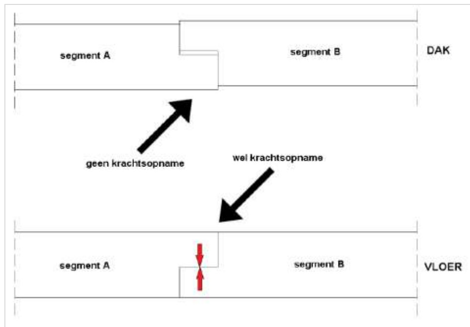
Figuur 84.1 - Verhinderend vervorming bij verschilzakking tussen tunnelsegmenten
