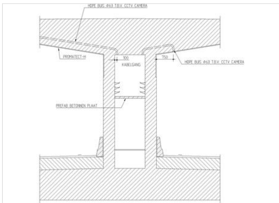
Figuur 285.1 - Doorsnede middenkanaal met mantelbuis voor CCTV camera
