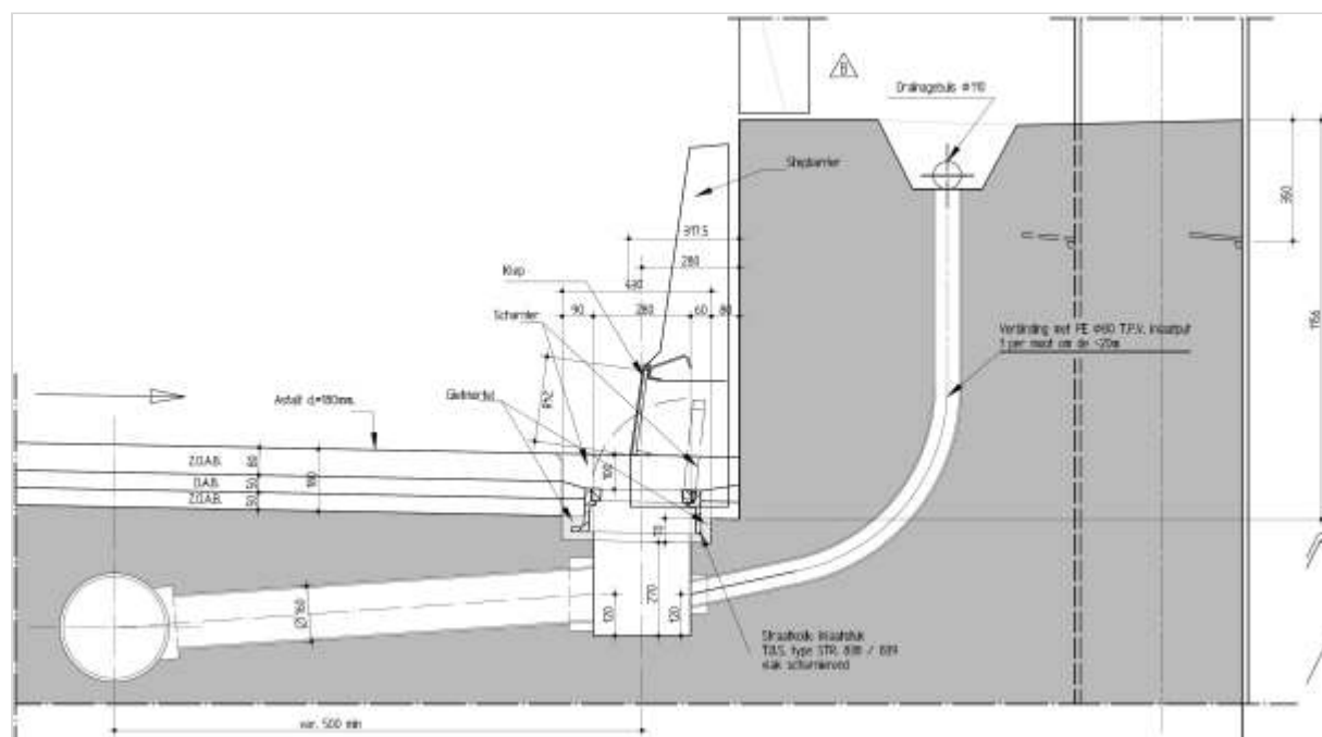
Figuur 412.1 - Aansluiting straatkolk op afvoerleiding
