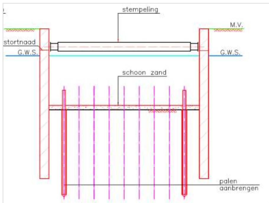
Figuur 181.2 - Bouwkuip met diepwanden en onderwaterbeton - fase 3
