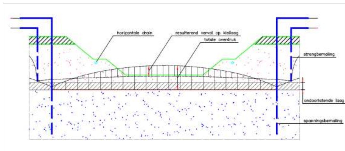
Figuur 166.3 - Gecombineerde spannings- en strengebemaling
