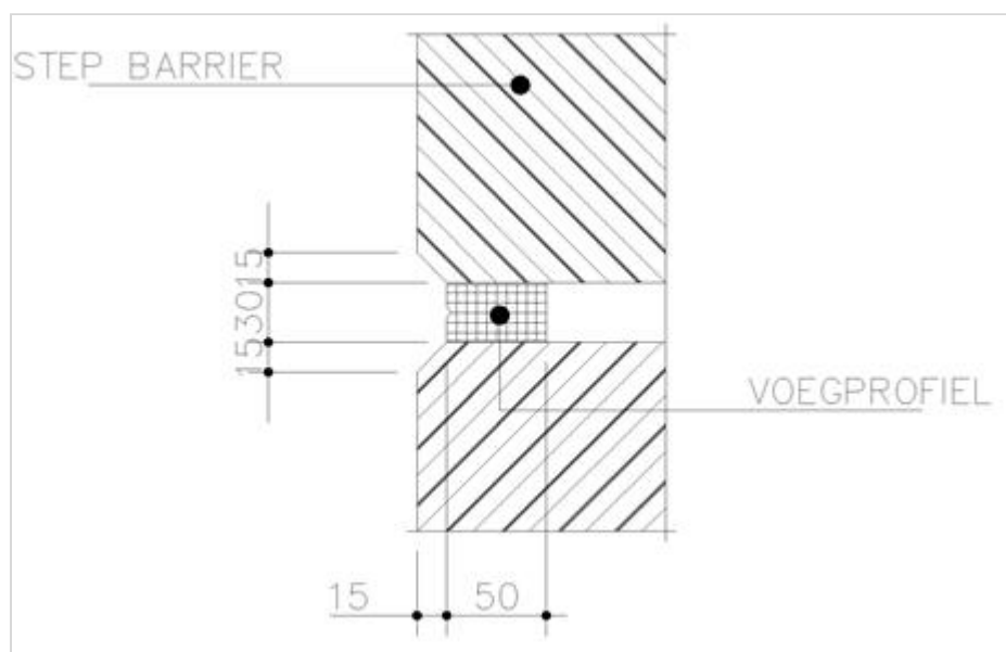
Figuur 259.3 - Voegprofiel step barrier middenberm doorsnede B
