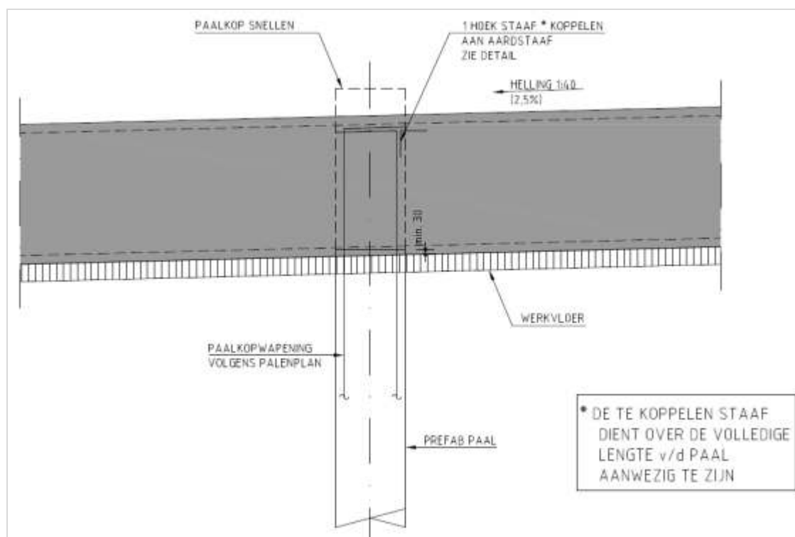
Figuur 480.3 - Detail koppeling aarding t.p.v. palen
