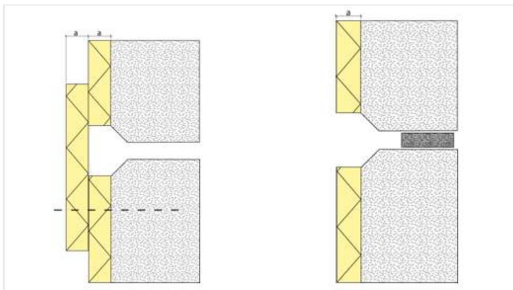
Figuur 315.4 - Voegen en dilataties ter voorkoming van branddoorslag
