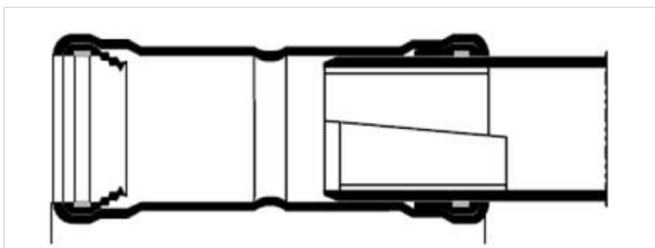
Figuur 270.3 - Verlengde U2-koppeling
