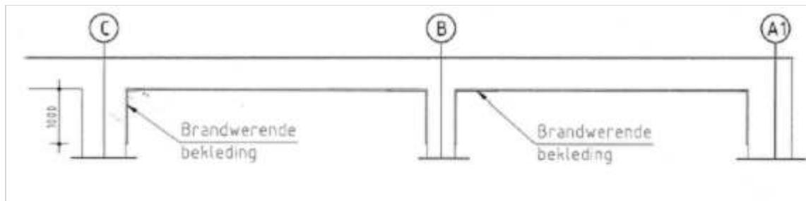
Figuur 498.4 - Principe doorsnede tunnel met brandwerende bekleding
