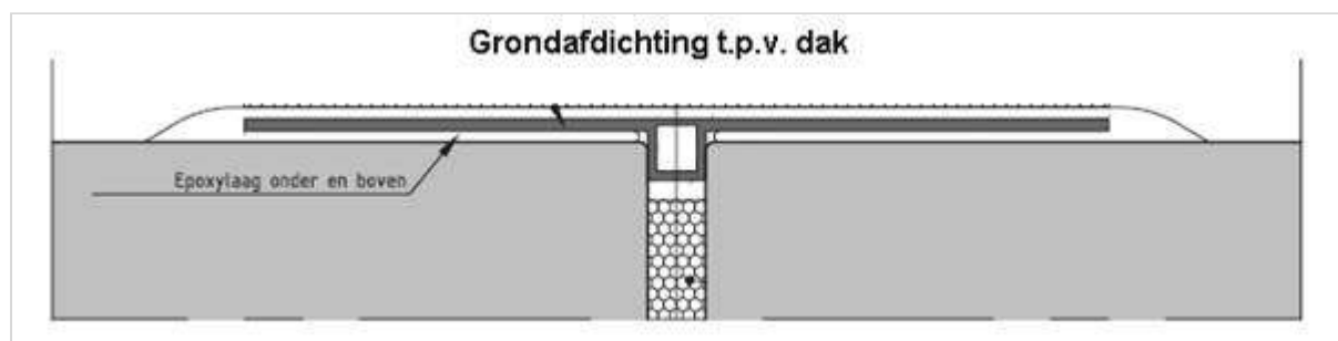
Figuur 257.2 - Buitenaafdichting met epoxylaag
