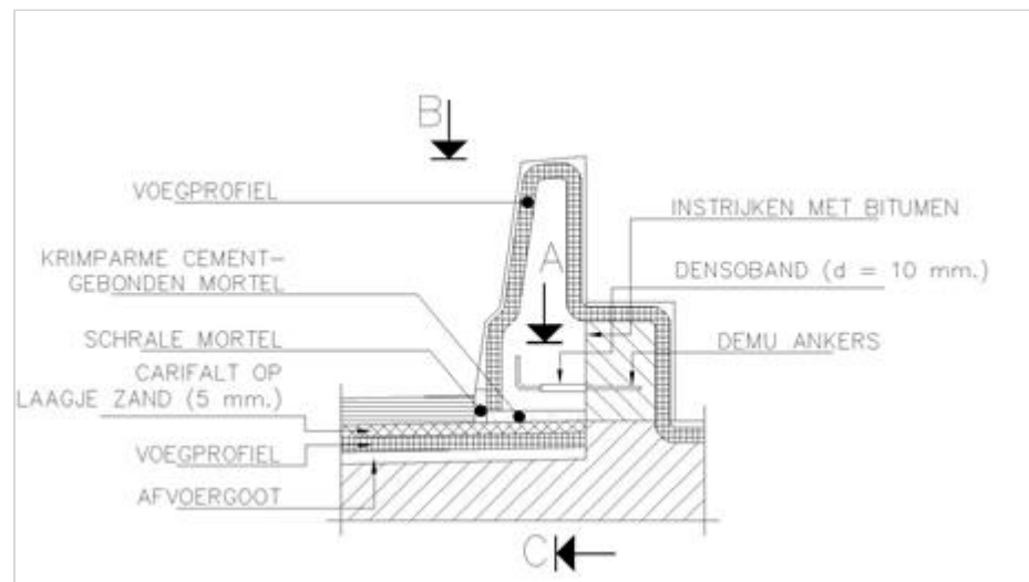
Figuur 259.1 - Aanzicht voegprofiel step barrier middenberm
