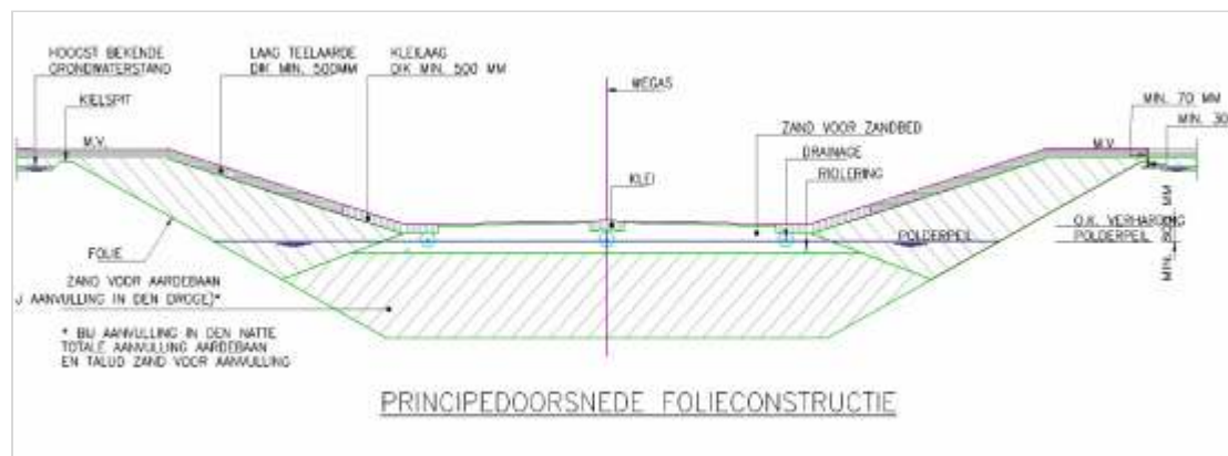
Figuur 228.1 - Oplossing met taluds
