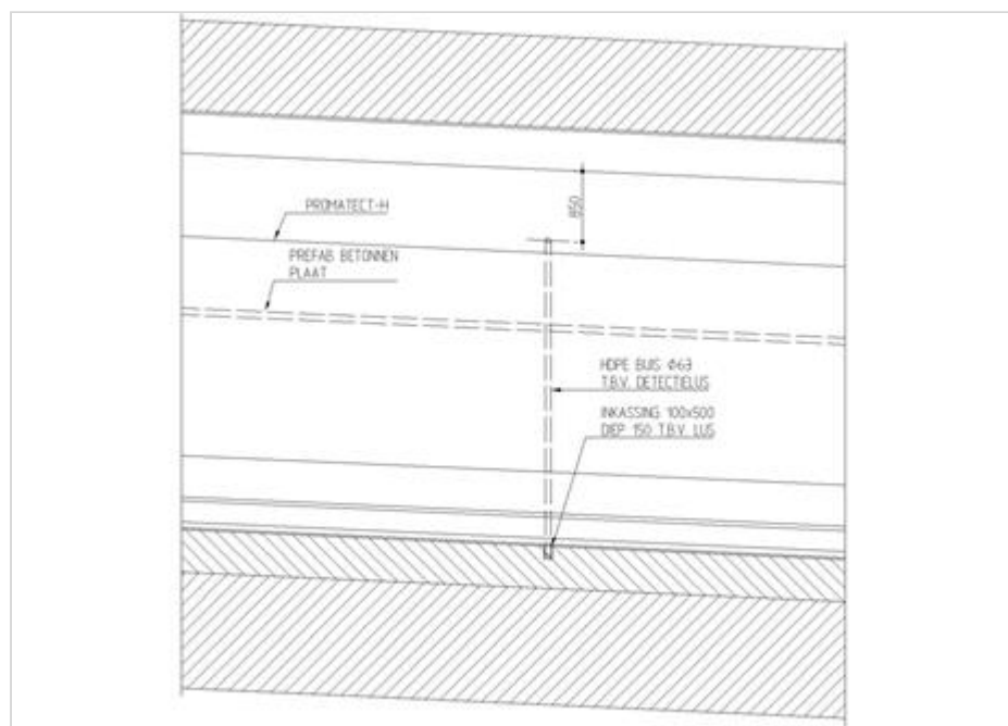
Figuur 284.2 - Aanzicht middenwand van 4-53
