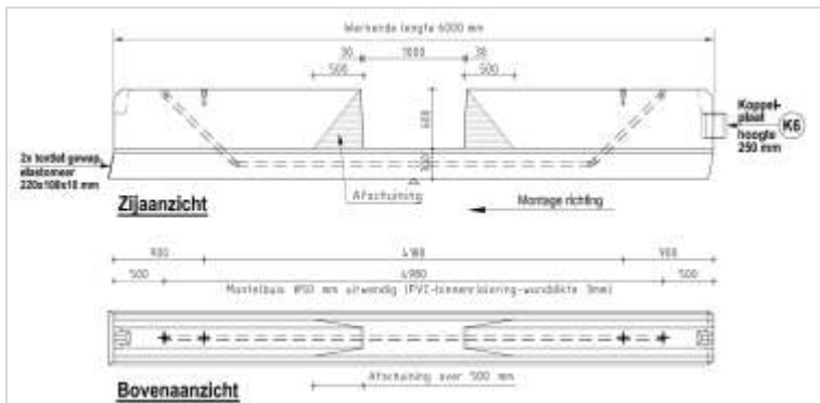
Figuur 378.1 - Locatie en ontwerp stepbarriers A2 Leidsche Rijntunnel
