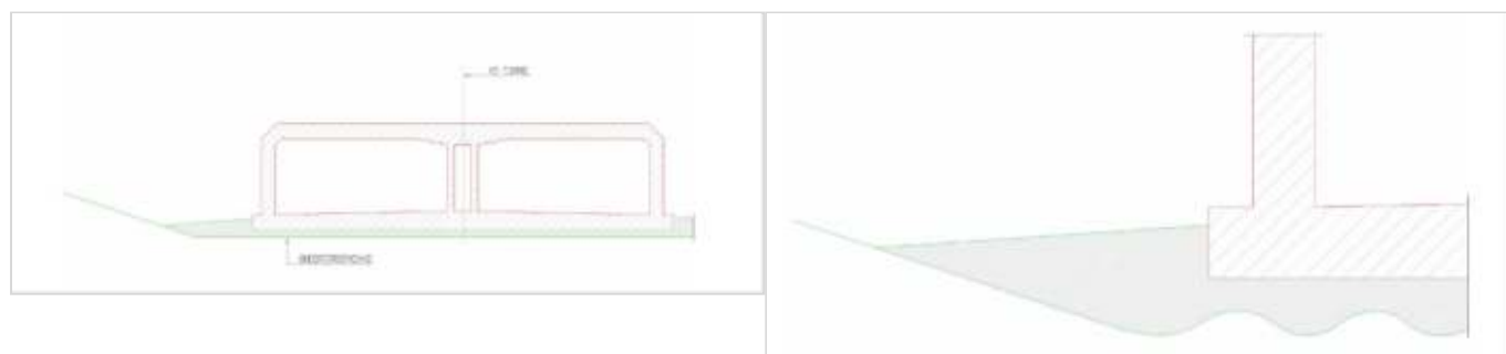
Figuur 241.1 - Fundering afgezonken tunnel op op onderspoelzand
