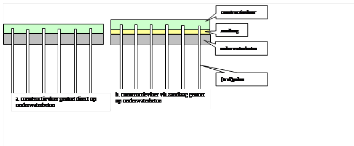
Figuur 664.3 - Principe constructievloer op onderwaterbetonvloer
