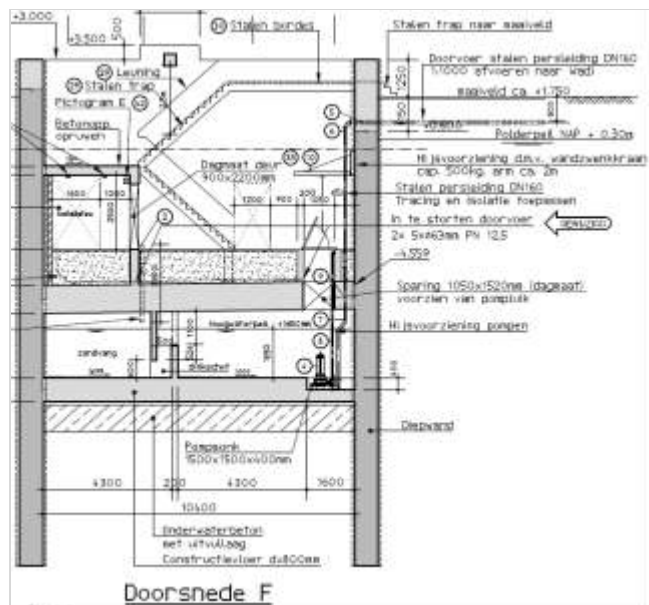
Figuur 413.4 - Langsdoorsnede waterkelder
