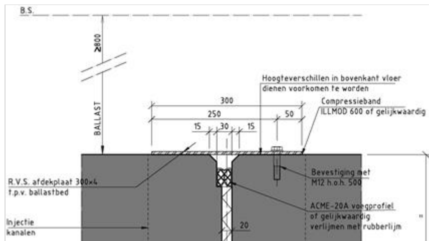
Figuur 266.2 - Voegovergang voor spoor in ballast zonder aanwezigheid van hemelwater
