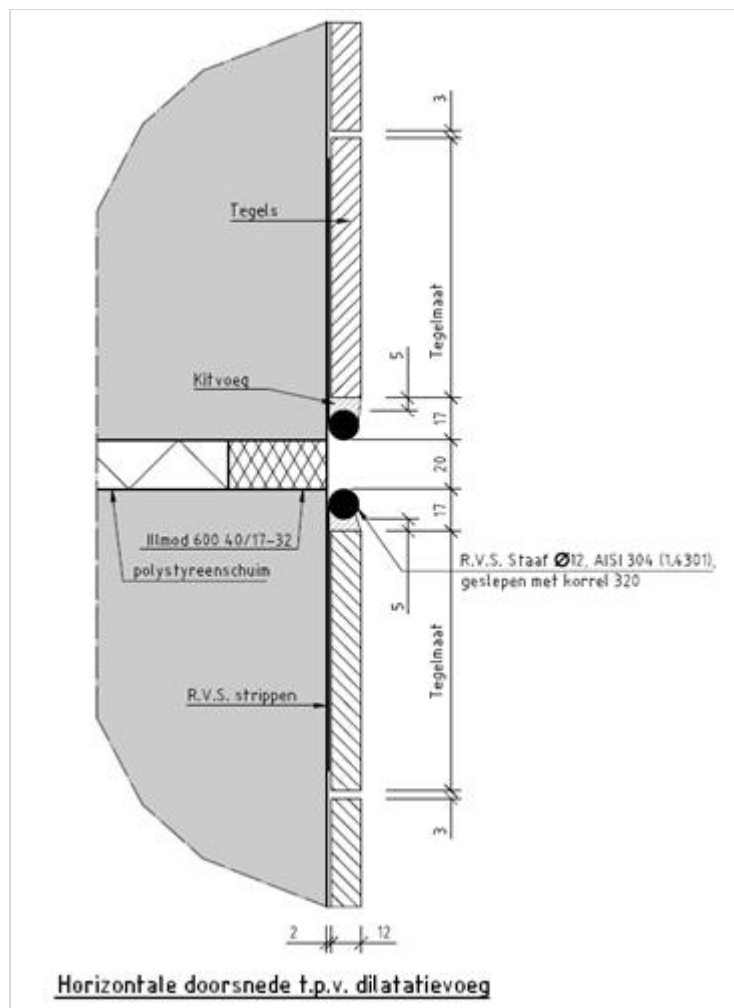
Figuur 507.2 - Principedetails wandafwerking tegels t.p.v. dilatievoeg
