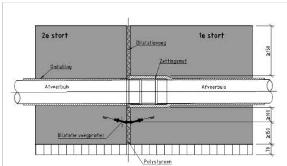
Figuur 502.1 - Principe doorsnede afvoerbuiss t.p.v. voegovergang
