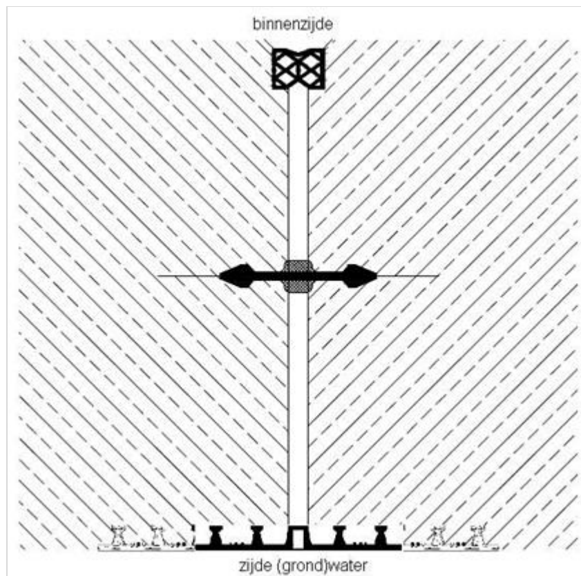
Figuur 255.1 - Detaillering wand
