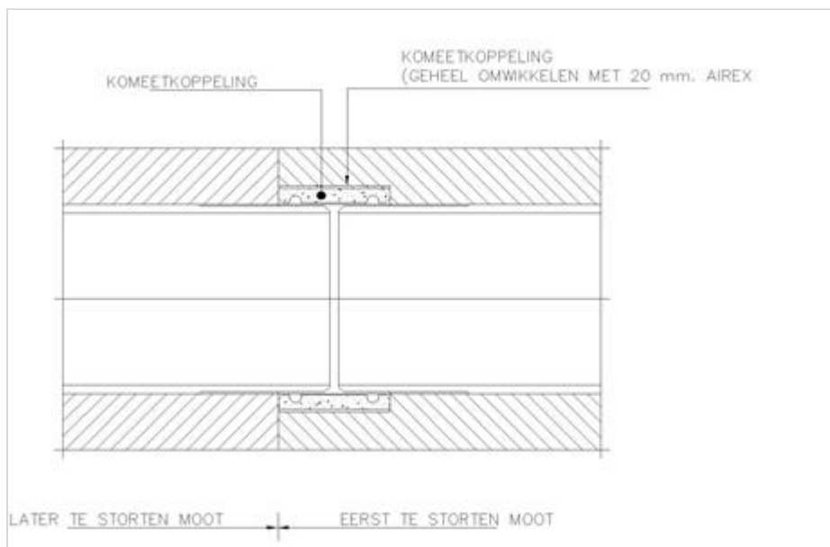
Figuur 270.1 - Detailontwerp buis met U2-koppeling
