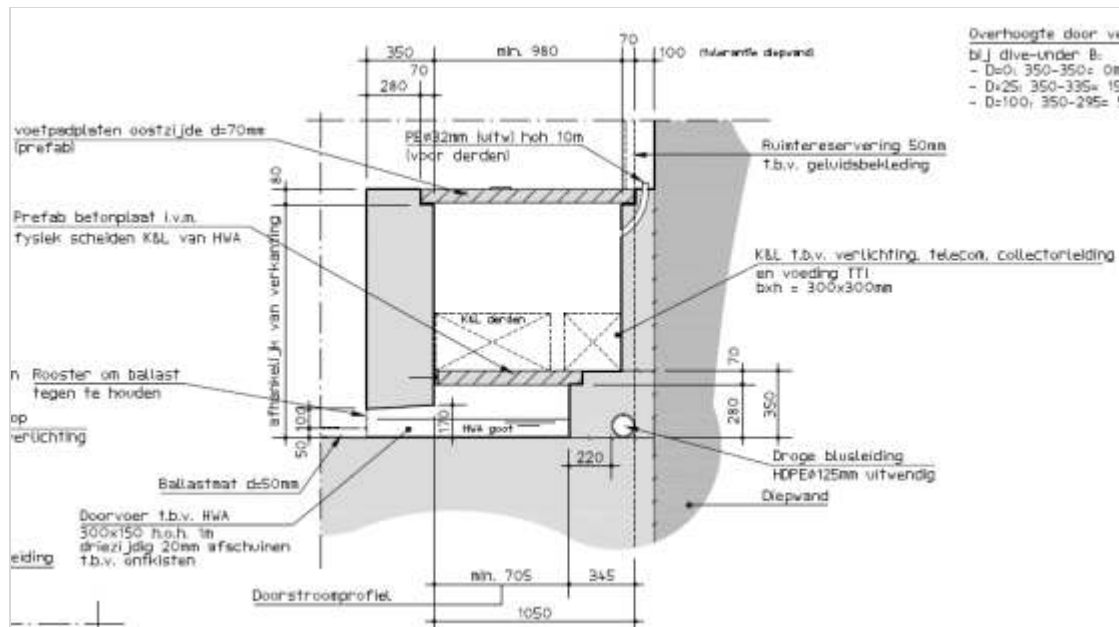
Figuur 398.1 - Afvoergoot onder vlucht/inspectiepad
