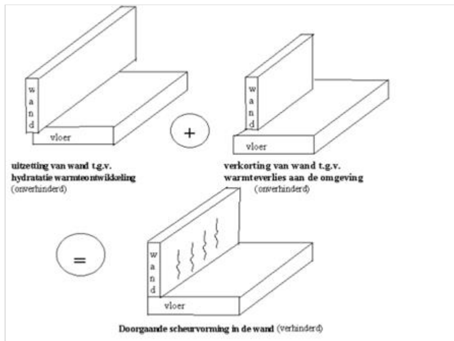
Figuur 664.2 - Principe van uitwendige verhindering van hydratatievervormingen
