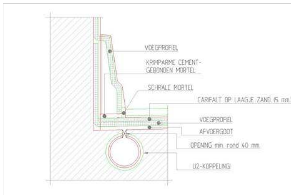
Figuur 256.1 - Voeg in aansluiting buitenwand – vloer; aan de voorzijde van de barrier is een doorlopend ACME profiel weergegeven; veelal wordt deze echter weg gelaten, in combinatie met een ruimere voeg tussen de barriers
