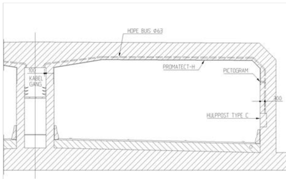
Figuur 281.1 - Doorsnede tunnel ter plaatse van hulppost type C; de mantelbuis voor het pictogram moet 3,2 m boven bk asfalt uitkomen
