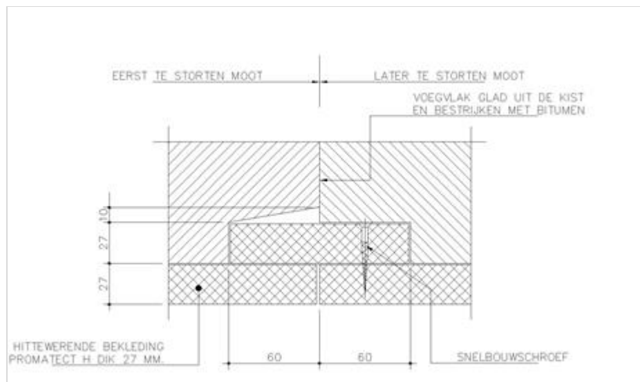
Figuur 268.1 - Detailontwerp hittewerende bekleding methode A;
