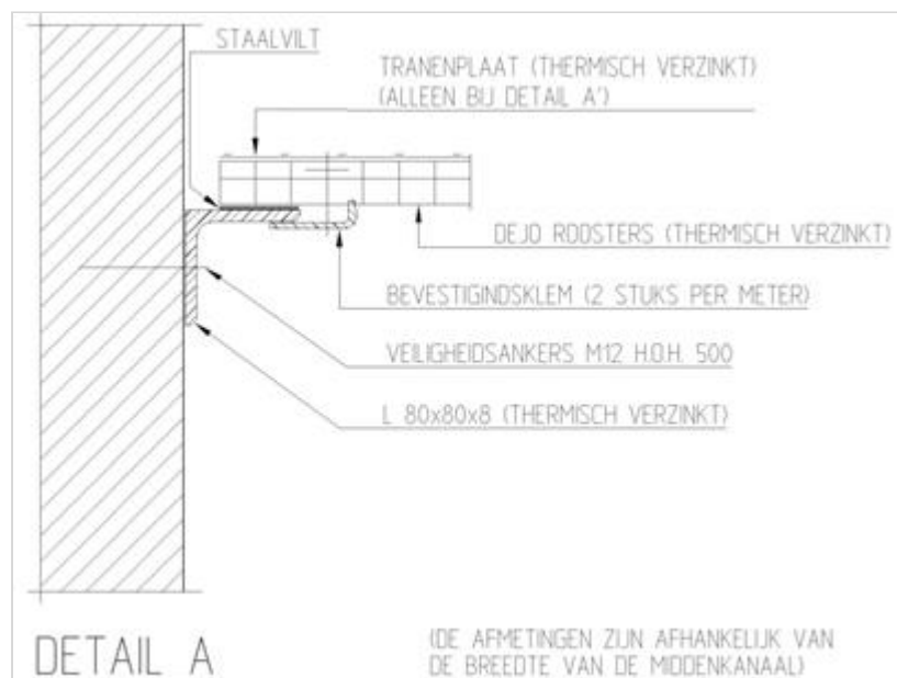
Figuur 509.1 - Roosters middentunnelkanaal
