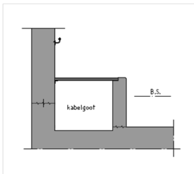
Figuur 500.1 - Principe doorsnede kabelgoot spoortunnel
