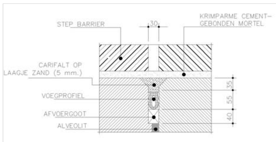
Figuur 258.4 - Voegprofiel step barrier buitenwand doorsnede C
