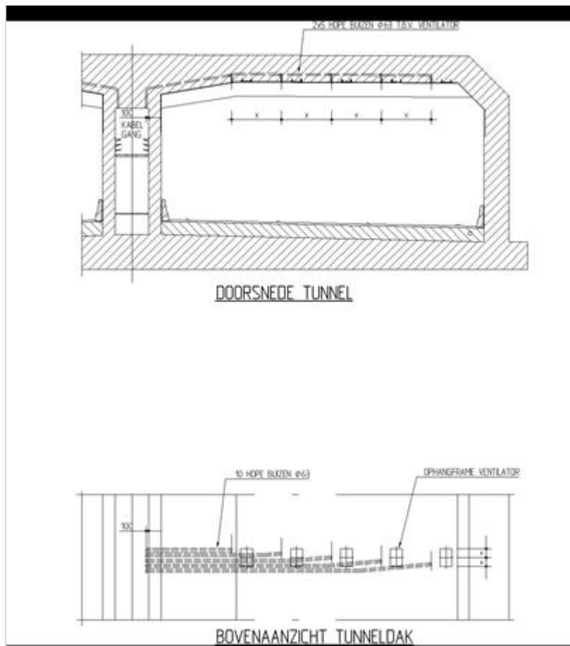
Figuur 294.1 - Doorsnede en bovenaanzicht tunnel ter plaatse van ventilator
