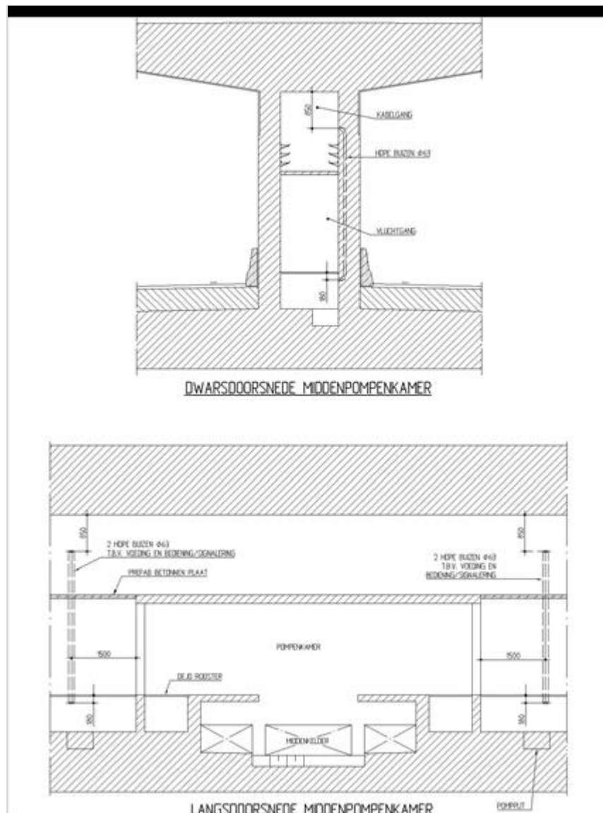
Figuur 300.1 - Dwars- en langsdoorsnede ter plaatse van middenpompkamer - pompput in de vloer
