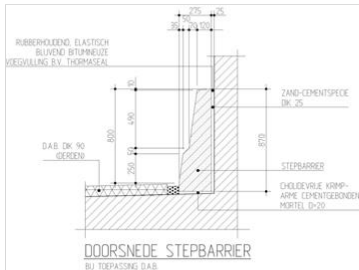
Figuur 452.1 - Doorsnede Stepbarrier bij toepassing DAB
