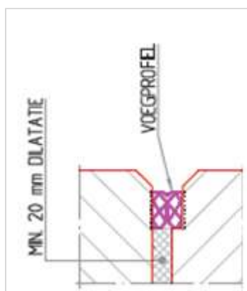
Figuur 253.1 - binnenzijde voeg vloer kabelkoker
