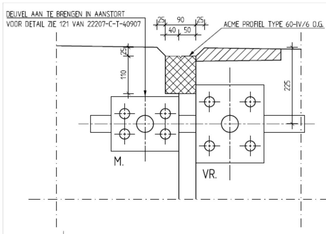
Figuur 370.7 - Horizontale stalen verdeuveling bij de zinkvoeg in de vloer van de HSL-tunnels
