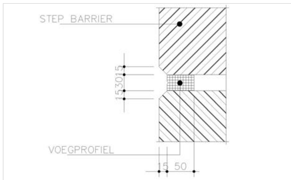
Figuur 258.3 - Voegprofiel step barrier buitenwand doorsnede B
