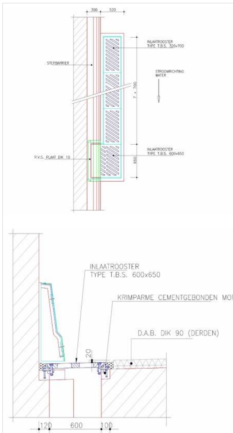
Figuur 408.1 - Inlaatroosters t.p.v. hoofdwaterkelder bij toepassing DAB
