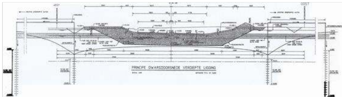
Figuur 188.5 - Half verdiepte ligging omlegging A 50 te Son - principe van de bemaling en de retourbemaling (figuren via Wolsink)
