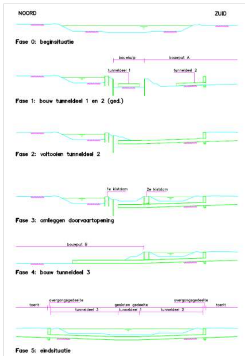
Figuur 212.1 - Fasering betonconstructie in bouwput met bemaling (tunnel Velsen)
