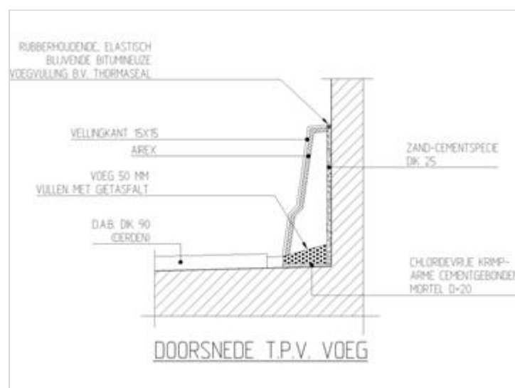
Figuur 453.1 - Doorsnede t.p.v. voeg bij toepassing DAB
