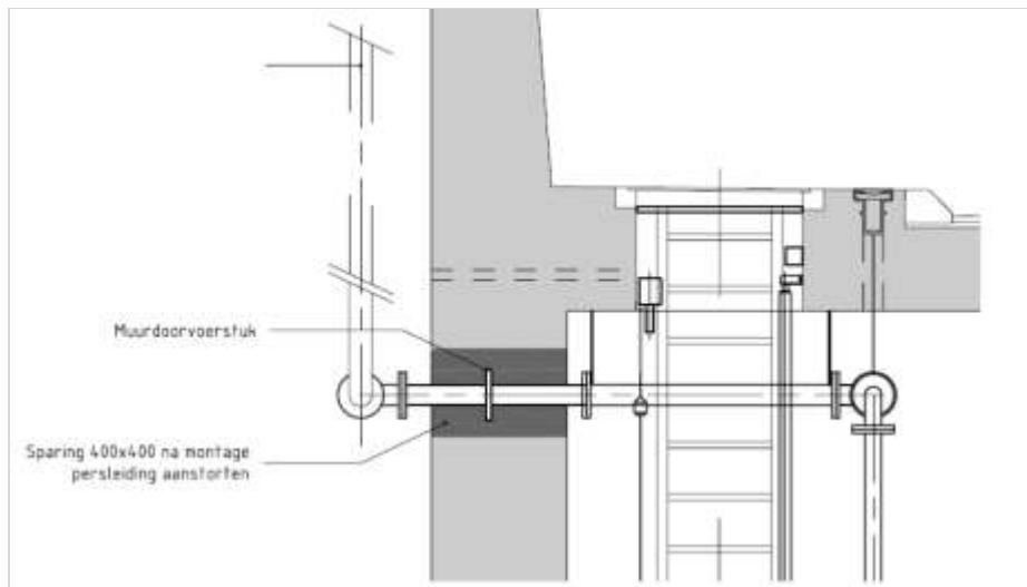
Figuur 301.1 - Muurdoorvoer persleiding
