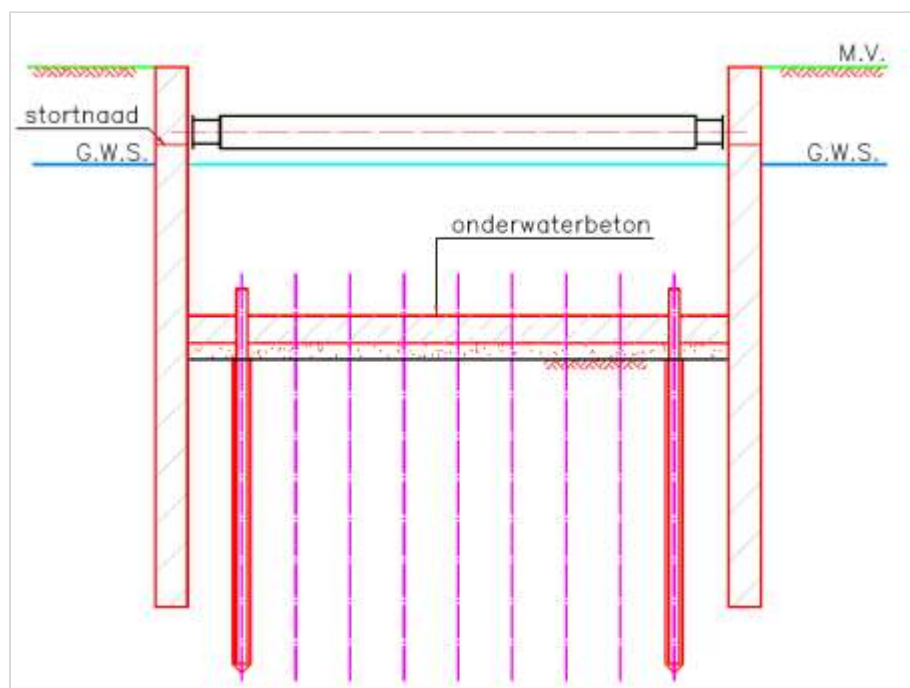
Figuur 181.3 - Bouwkuip met diepwanden en onderwaterbeton - fase 4
