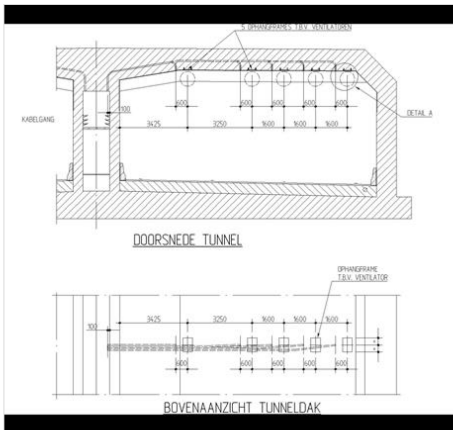
Figuur 295.1 - Doorsnede en bovenaanzicht tunnel ter plaatse van ophangframes ventilator
