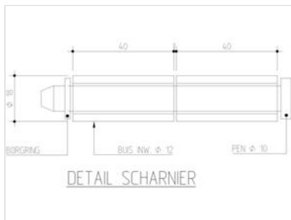
Figuur 457.1 - Aanzicht en details geleidebarrier t.p.v. inlaatput
