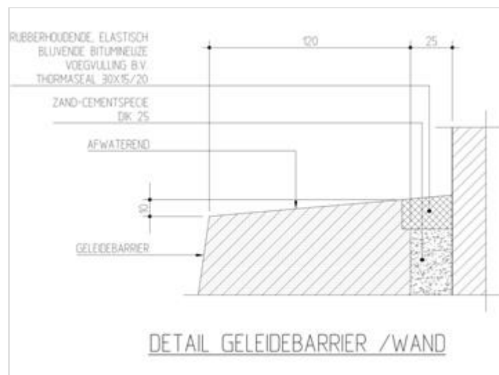
Figuur 454.1 - Detail geleidebarrier/wand
