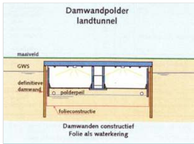
Figuur 228.4 - Folieconstructie bij gesloten tunnel
