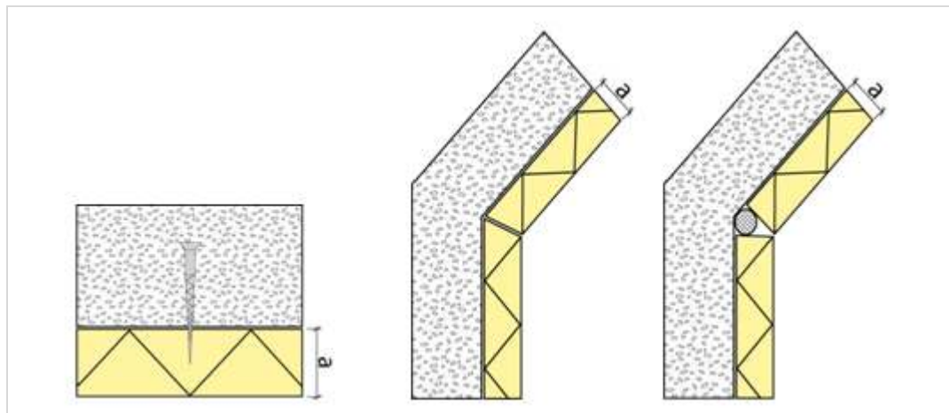
Figuur 315.1 - Snelbouwschroeven
