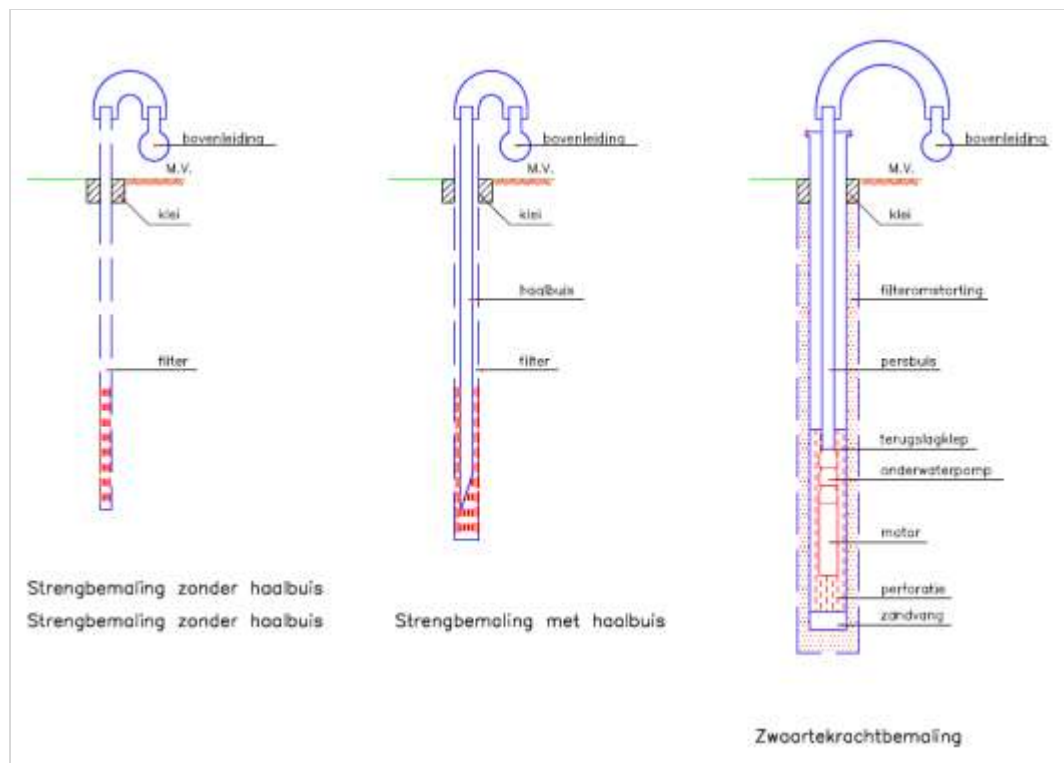
Figuur 166.2 - Typen bemaling
