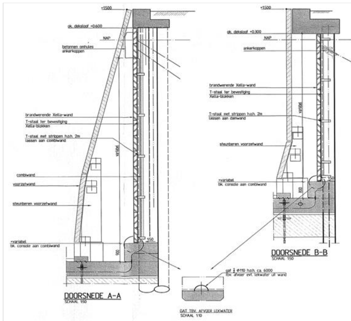
Figuur 498.2 - Absorberende constructie project A4 Leiderdorp
