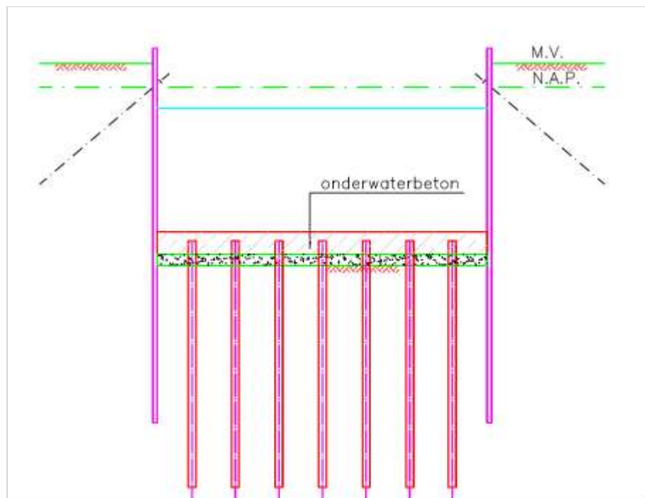
Figuur 177.4 - Bouwkuip met permanente damwanden en onderwaterbeton - fase 4
