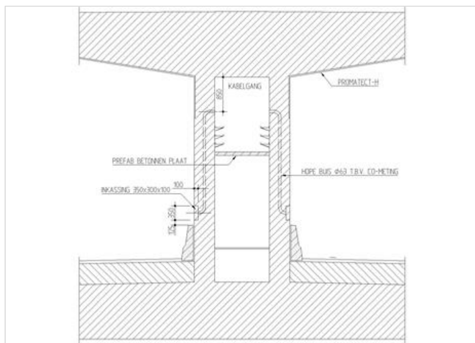
Figuur 283.1 - Doorsnede middenkanaal met mantelbuis voor CO-meetsysteem
