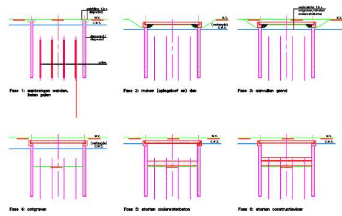
Figuur 214.1 - Fasering wanden/dak methode bij natte methode
