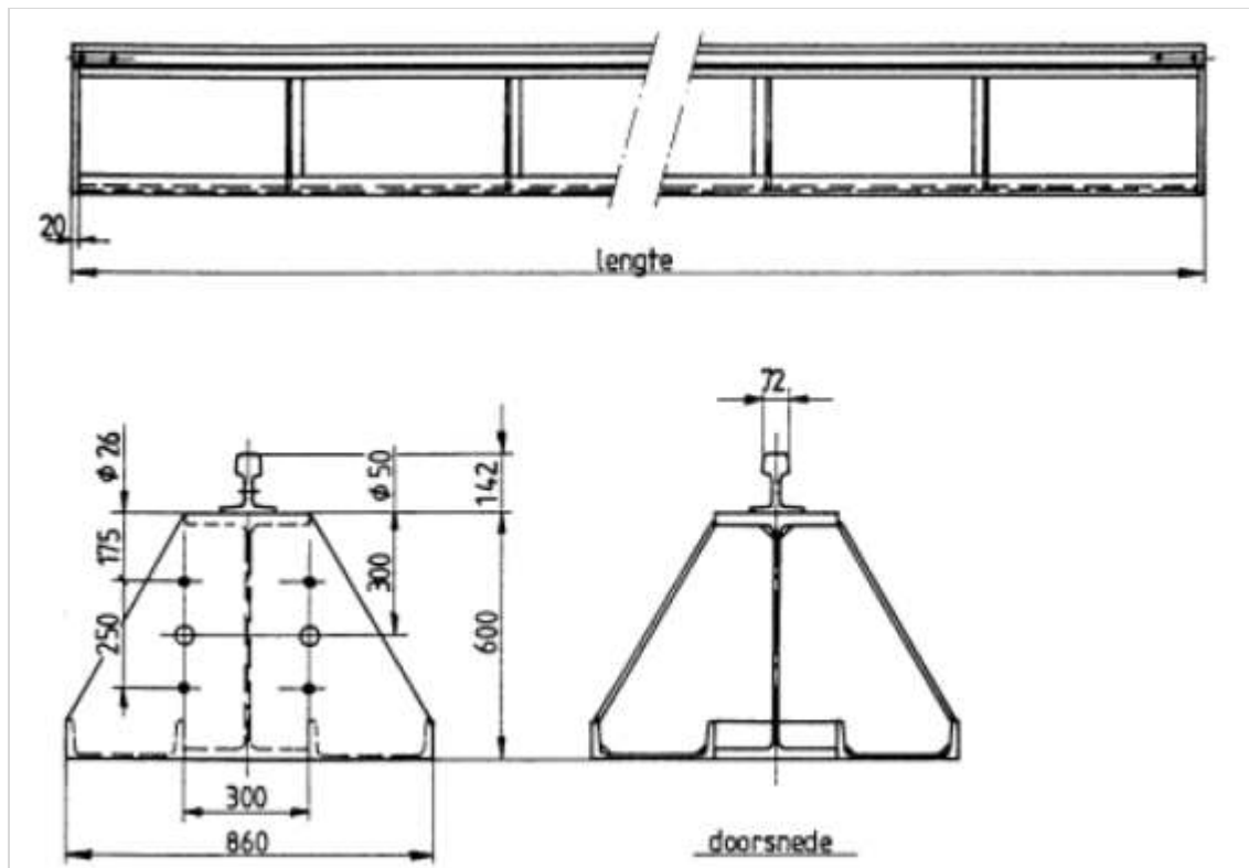
Figuur 639.1 - Voorbeeld railbalk
