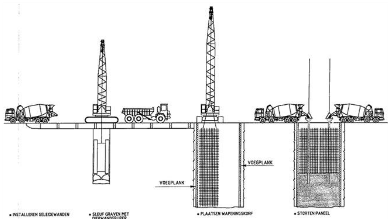
Figuur 555.1 - Methode diepwand
