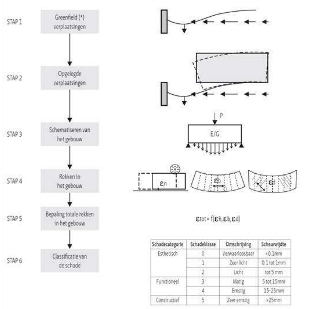
Figuur 153.1 - Schematisering van de LTSM benadering voor bouwkuip waarbij greenfield (en) staat voor maaiveldvervorming zonder gebouw
