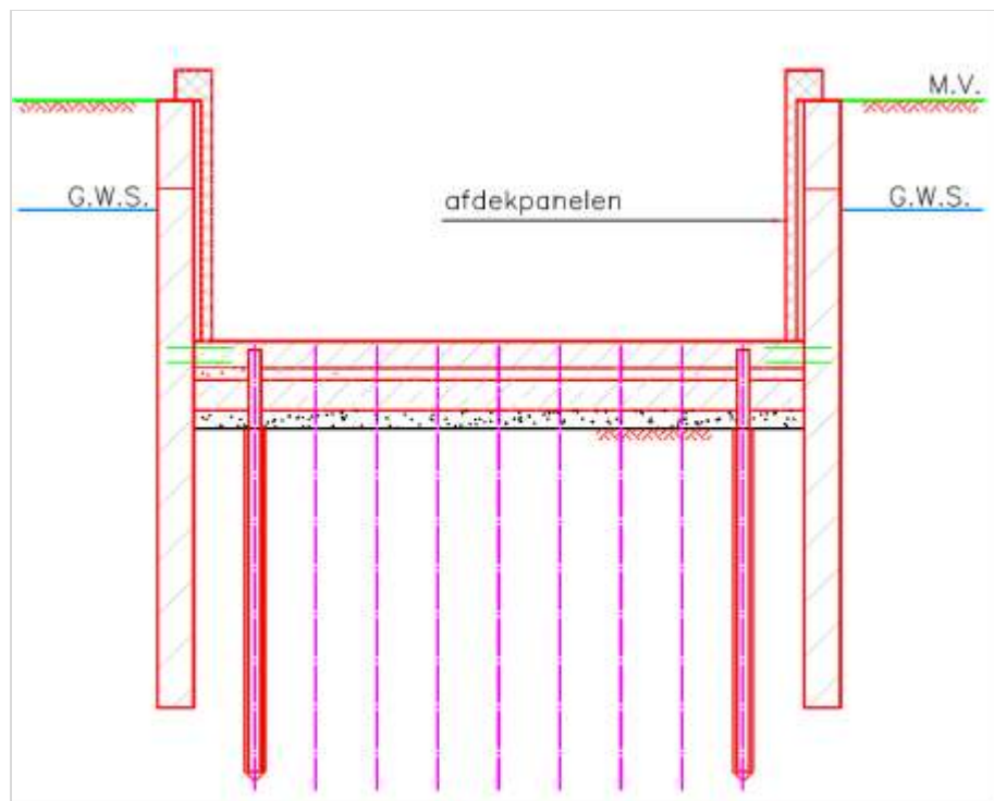
Figuur 181.6 - Bouwkuip met diepwanden en onderwaterbeton - fase 7
