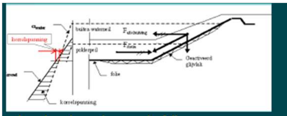
Figuur 235.1 - Mechanisme evenwicht folieconstructie
