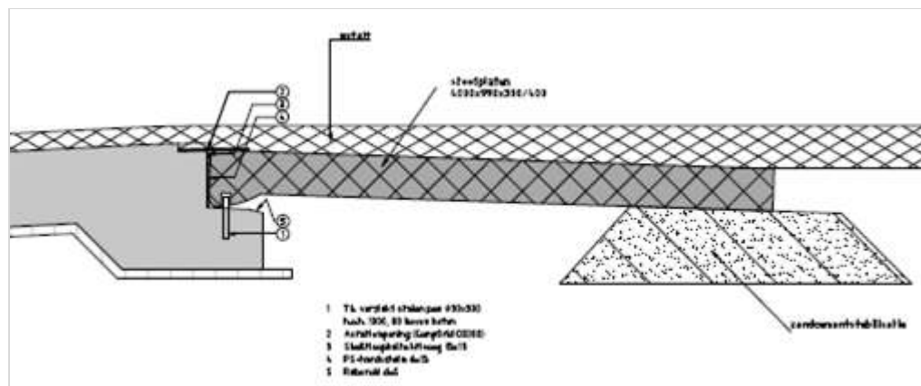
Figuur 470.1 - Detail stootplaat
