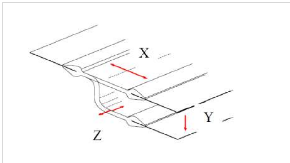
Figuur 269.3 - Rubbermetalen voegstrook
