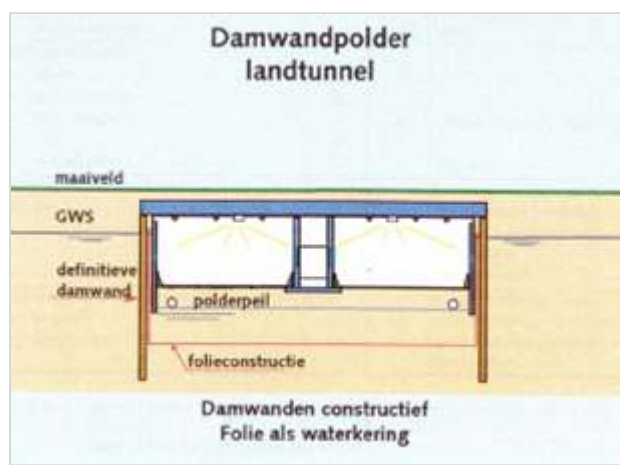
Figuur 231.4 - Folieconstructie bij gesloten tunnel
