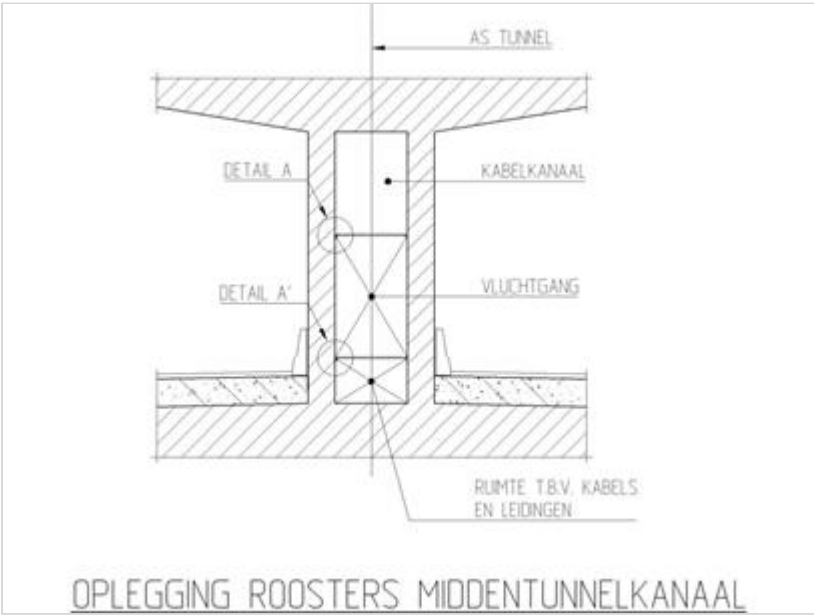
Figuur 468.1 - Aanzicht en details plaat in middenkanaal
