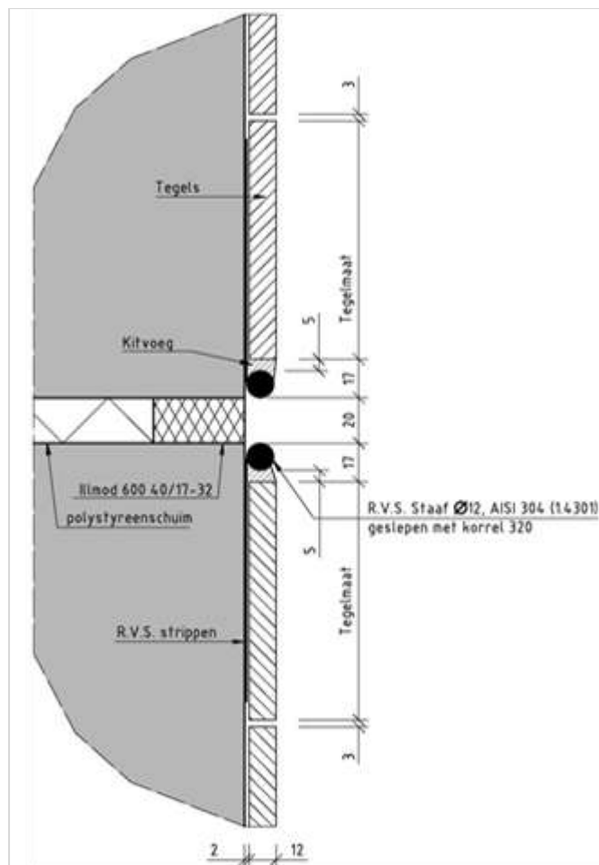
Figuur 264.2 - Detailontwerp tegelwerk - toepassing RVS staaf
