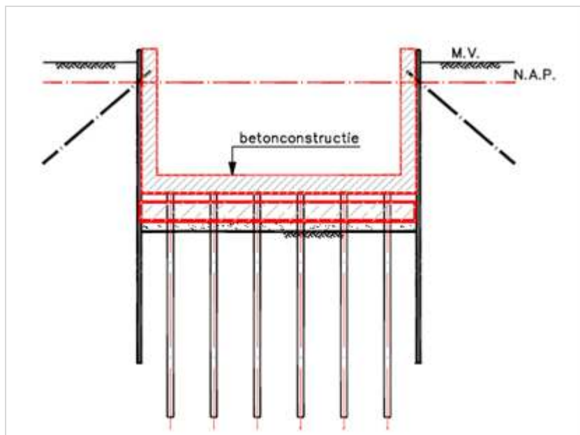
Figuur 172.6 - Bouwkuip met damwanden, onderwaterbeton (OWB) en trekpalen - fase 6
