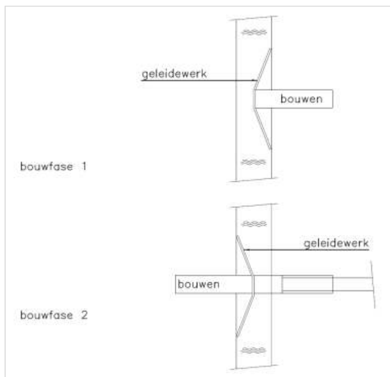
Figuur 210.3 - Principe fasering - variant B2
