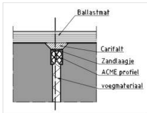
Figuur 266.3 - Dilatievoeg tunnelvloer onder ballastmat
