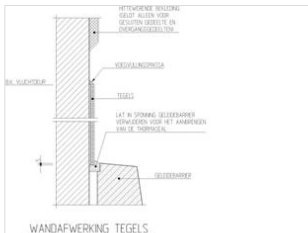
Figuur 507.1 - Principedetail wandafwerking tegels
