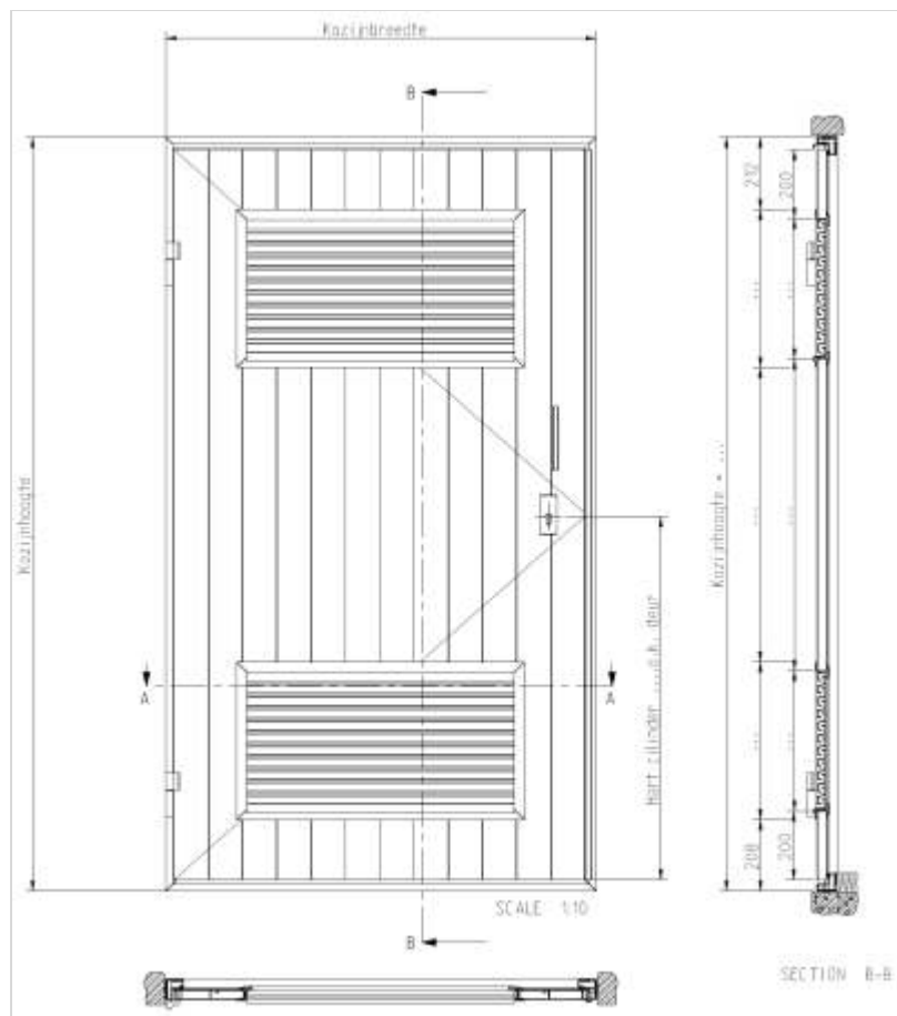
Figuur 439.1 - Trafodeur
