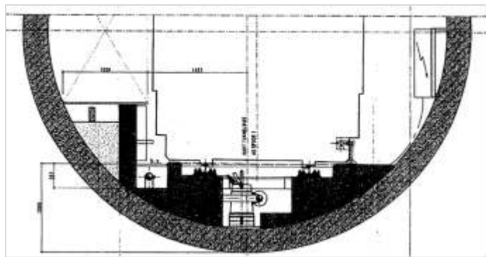
Figuur 400.1 - Pompput Boortunnel Statenweg Rotterdam
