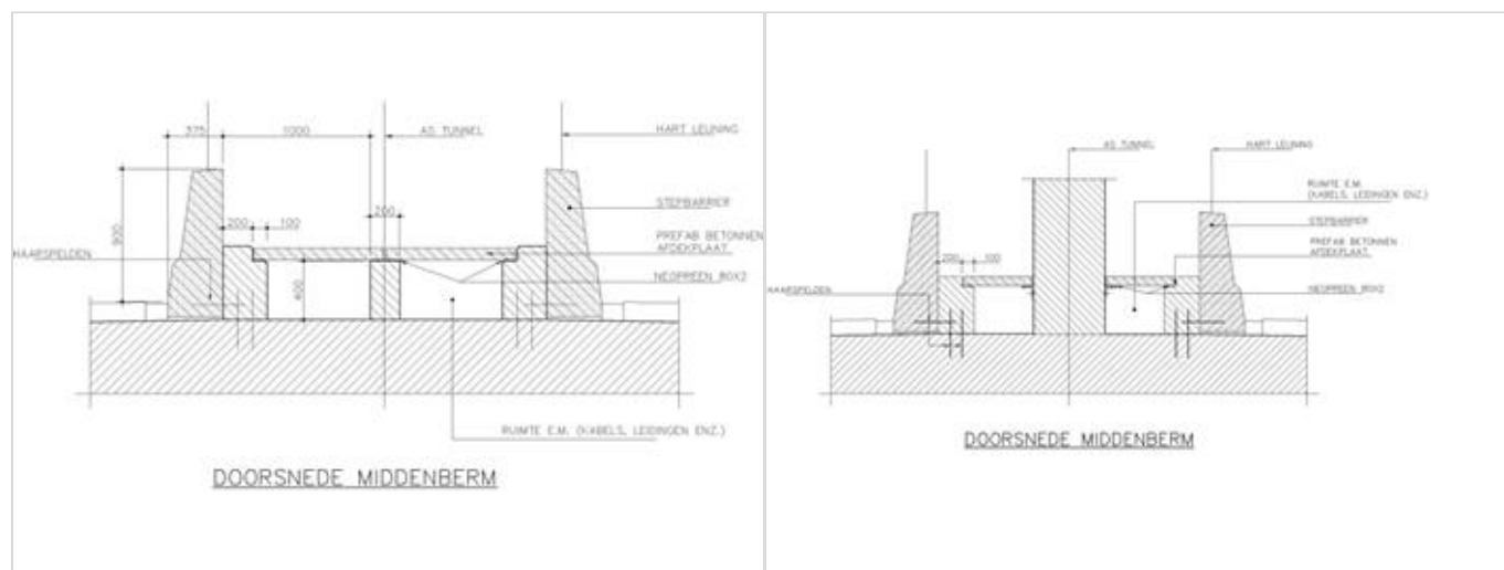
Figuur 469.1 - Doorsneden en detail afdekplaat in middenberm
