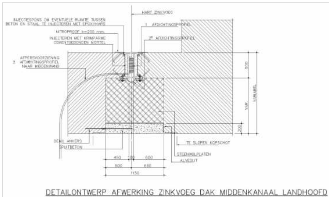
Figuur 335.1 Zinkvoeg met gezet profiel
