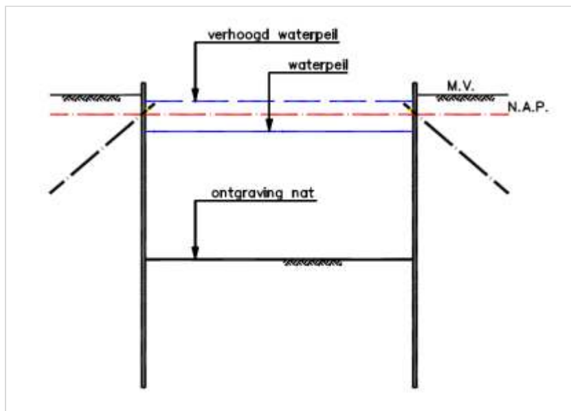
Figuur 172.2 - Bouwkuip met damwanden, onderwaterbeton (OWB) en trekpalen - fase 2
