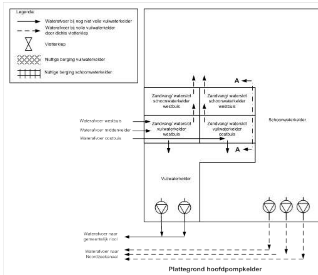
Figuur 412.5 - Schematische opzet hoofdwaterkelder
