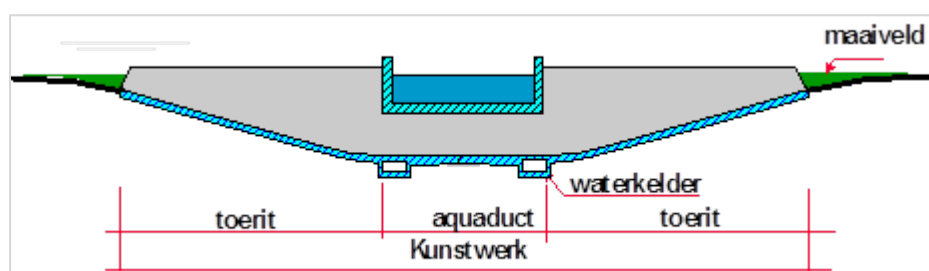
Figuur 8.1 - Aquaduct
