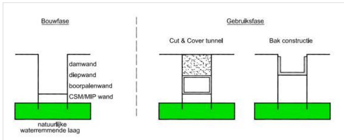
Figuur 46.2 - Bouwkuip met een natuurlijke waterremmende laag
