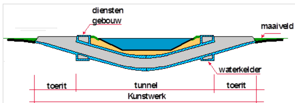
Figuur 7.1 - Tunnel onder een watergang
