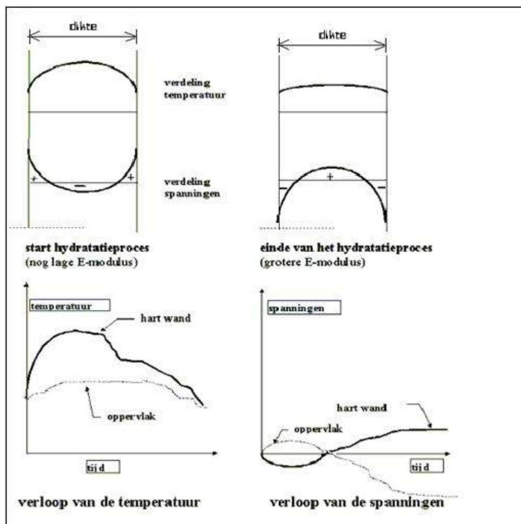
Figuur 664.1 - Principe van inwendige verhinderend van hydratatievormingen
