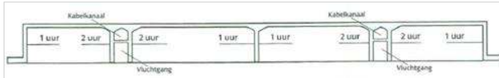
Figuur 380.1 - Hittewerendheid A2 Leidsche Rijntunnel
