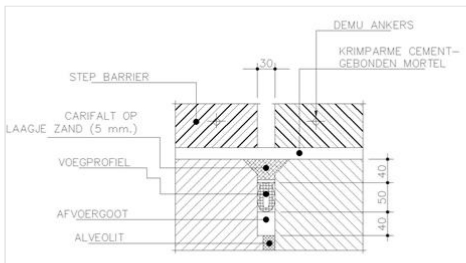
Figuur 259.4 - Voegprofiel step barrier middenberm doorsnede C
