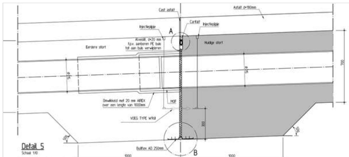
Figuur 412.3 - HWA-leiding bij dilatatievoeg
