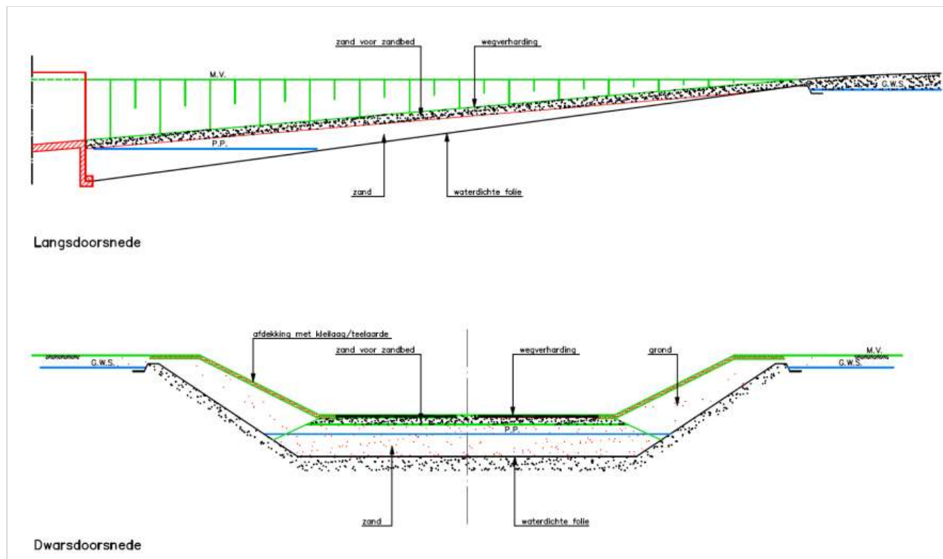
Figuur 188.1 - Kunststoffolie in den droge aangebracht - langs- en dwarsdoorsnede
