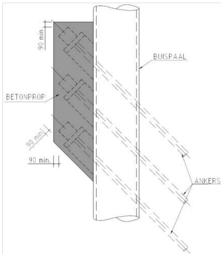
Figuur 498.3 - Voorzetwanden in afspatongevoelig beton (toegepast bij tunnel Swalmen A73)
