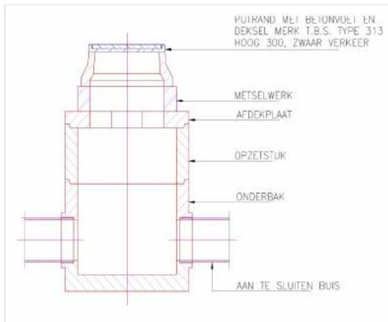
Figuur 390.1 - Inspectieput met afdekplaat
