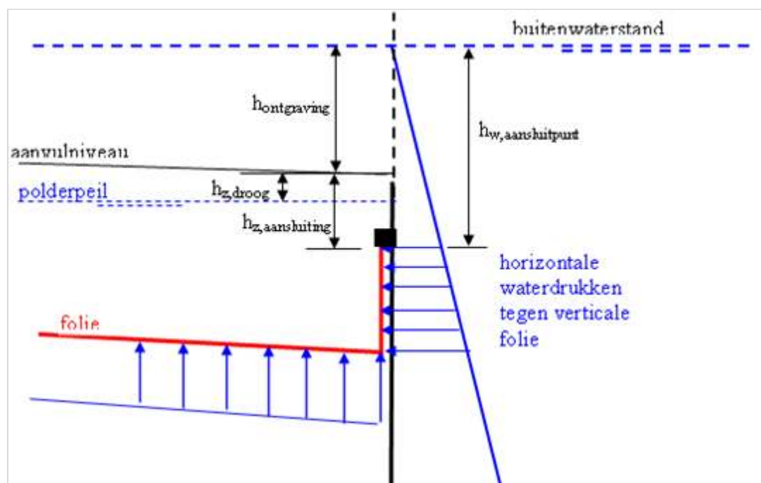
Figuur 236.1 - Waterdrukverschillen tegen de folie
