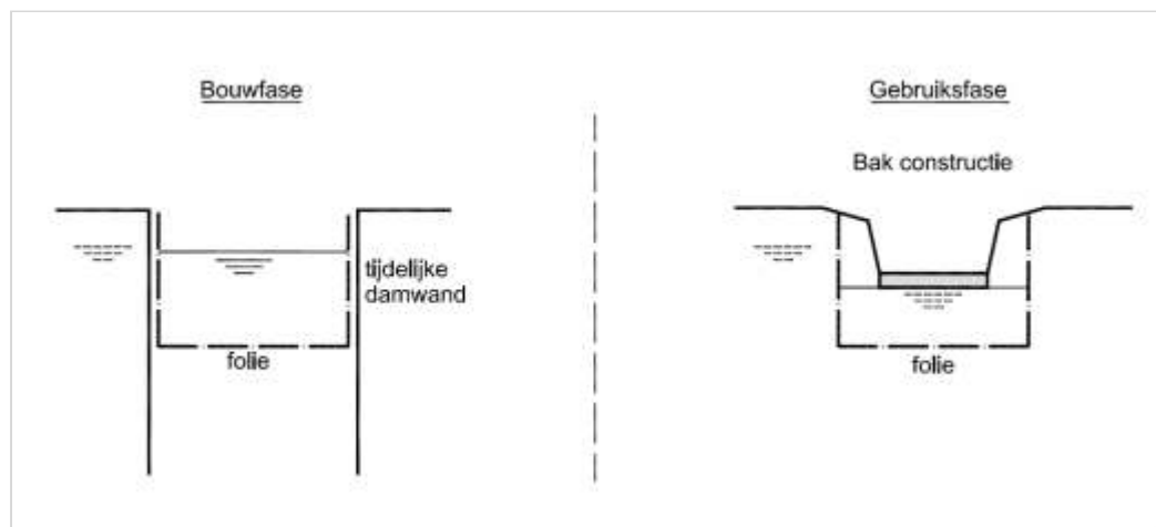
Figuur 46.4 - Polderconstructie met bouwkuip en folie
