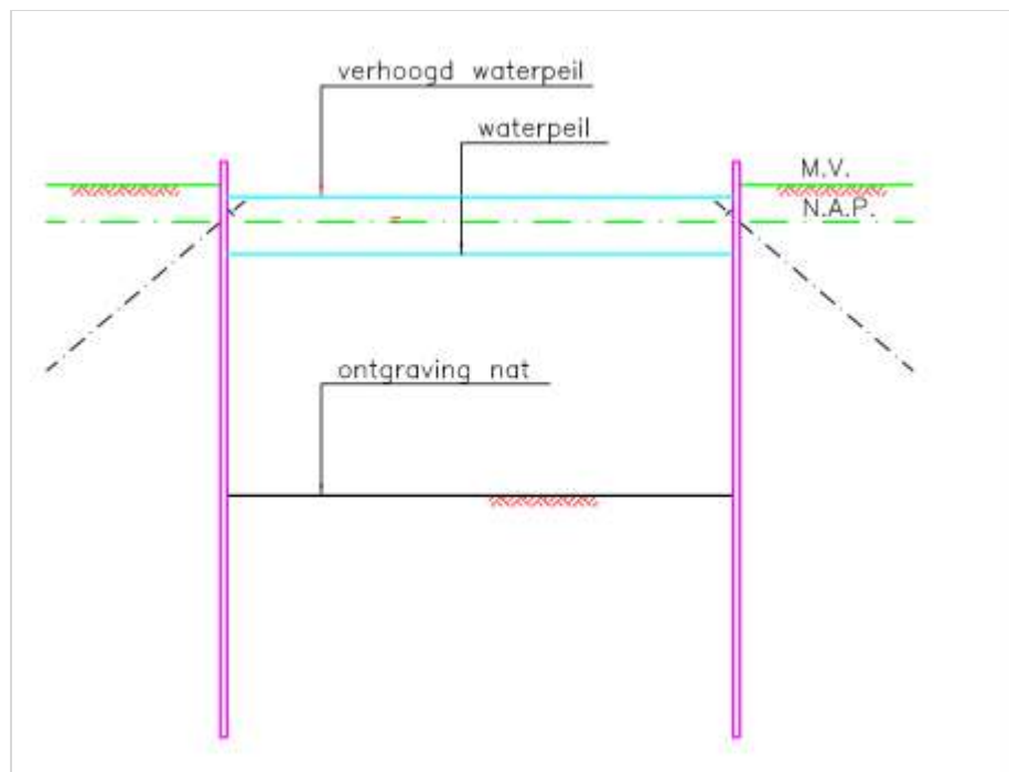
Figuur 177.2 - Bouwkuip met permanente damwanden en onderwaterbeton - fase 2
