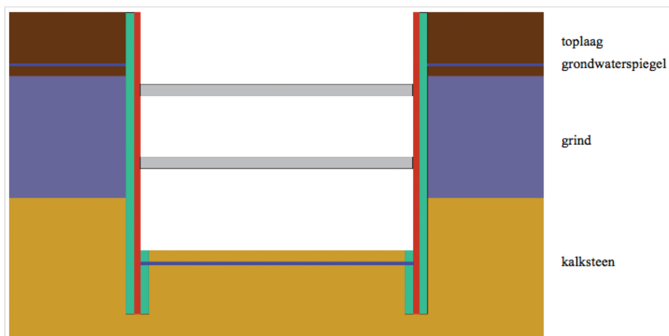
Figuur 159.2 - Bouwput A2 tunnel te Maastricht met gestempelde damwanden in cement-bentoniet schermen (zie [82] )
