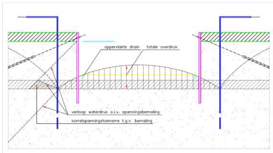
Figuur 166.3 - Gecombineerde spannings- en strengebemaling
