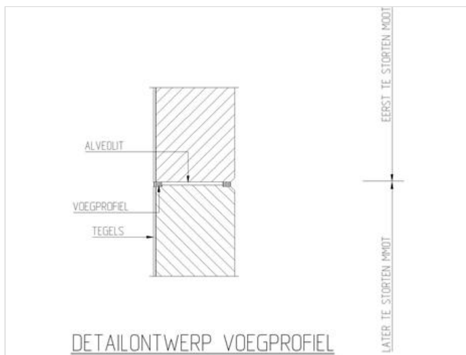
Figuur 254.2 - Voeg in middenwand met tegelwerk *)
