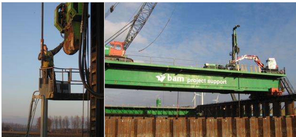
Figuur 623.2 - Inbrengen van GEWI palen vanaf traverse
