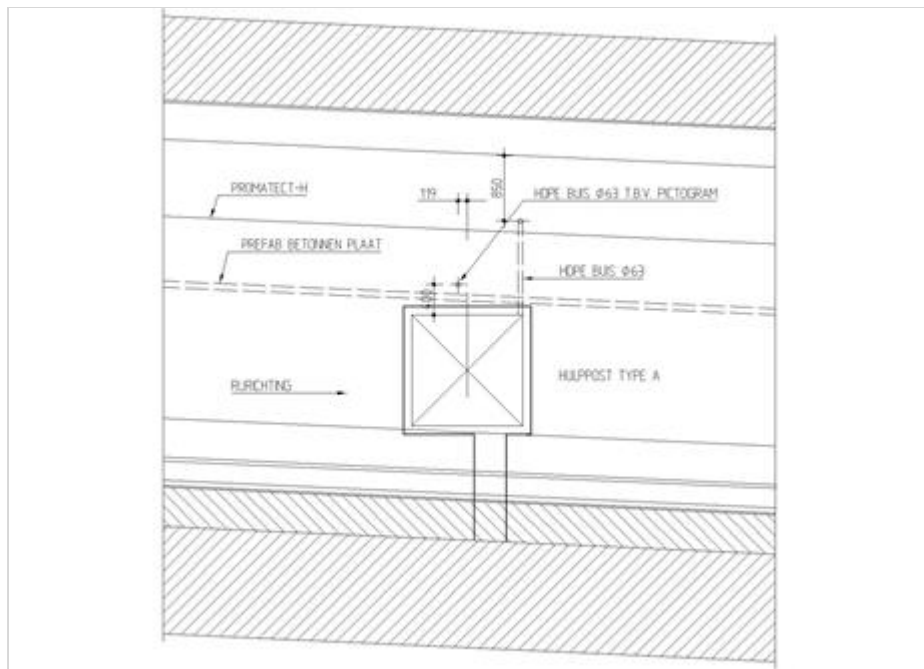
Figuur 280.2 - Aanzicht hulpmaat type A
