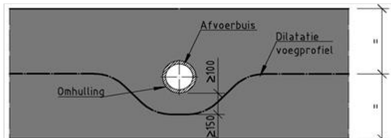
Figuur 257.3 - Dilatatievoegprofiel nabij buisleiding in dak
