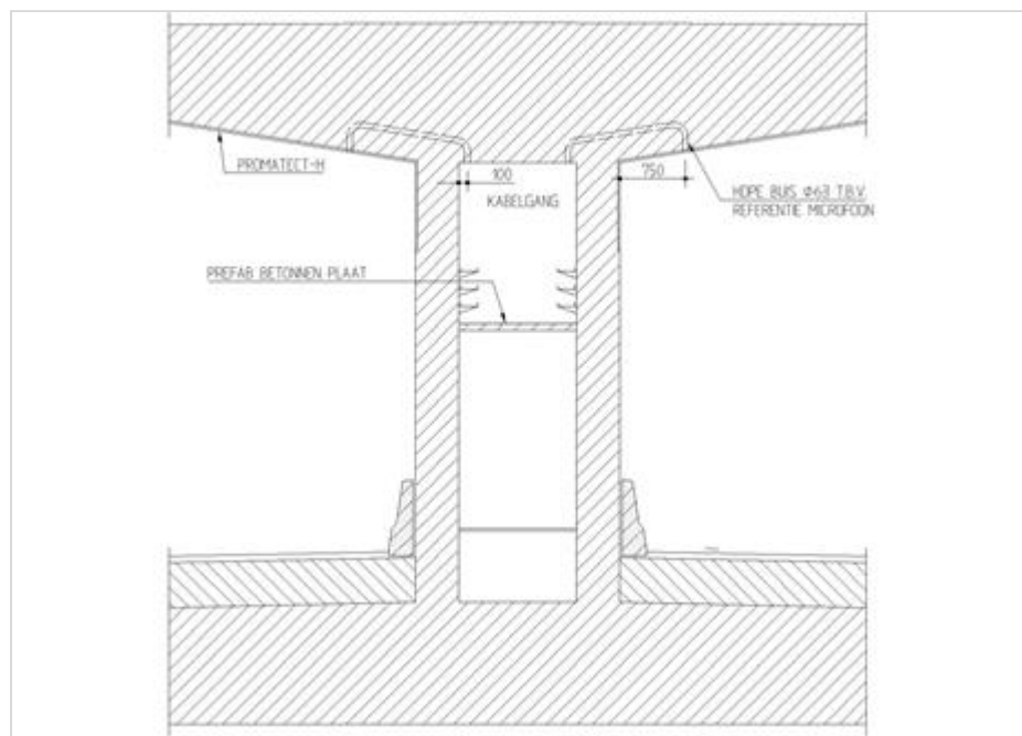
Figuur 286.1 - Doorsnede middenkanaal met mantelbuis voor referentiemicrofoon
