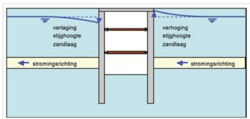
Figuur 141.1 - Resultaat verstoring grondwaterstroming
