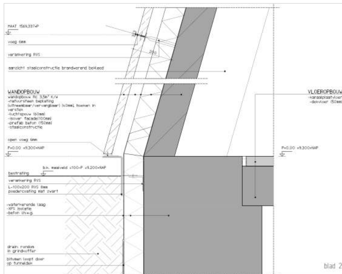
Figuur 440.1 - Gevelaansluiting met vloer
