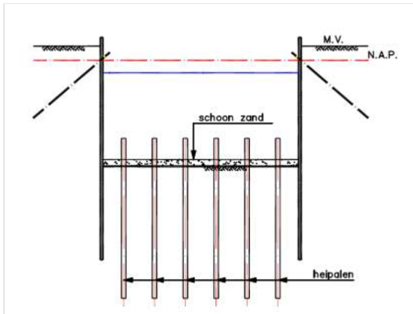
Figuur 172.3 - Bouwkuip met damwanden, onderwaterbeton (OWB) en trekpalen - fase 3
