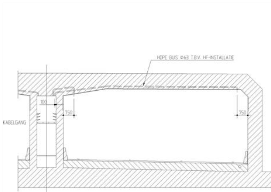
Figuur 296.1 - Doorsnede tunnel ter plaatse van radiocommunicatie installatie
