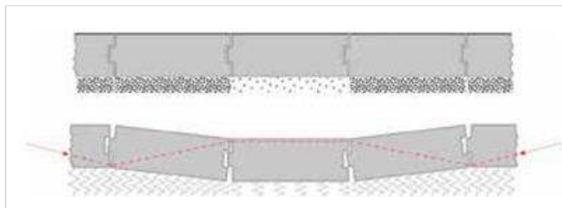
Figuur 100.3 - Verloop druklijn als gevolg van verschilzakking.
