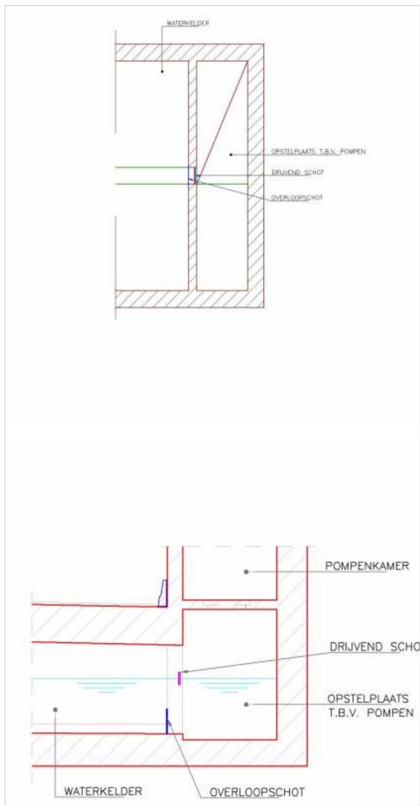
Figuur 405.1 - Principe-indeling hoofdwatertank met bezinkbassin
