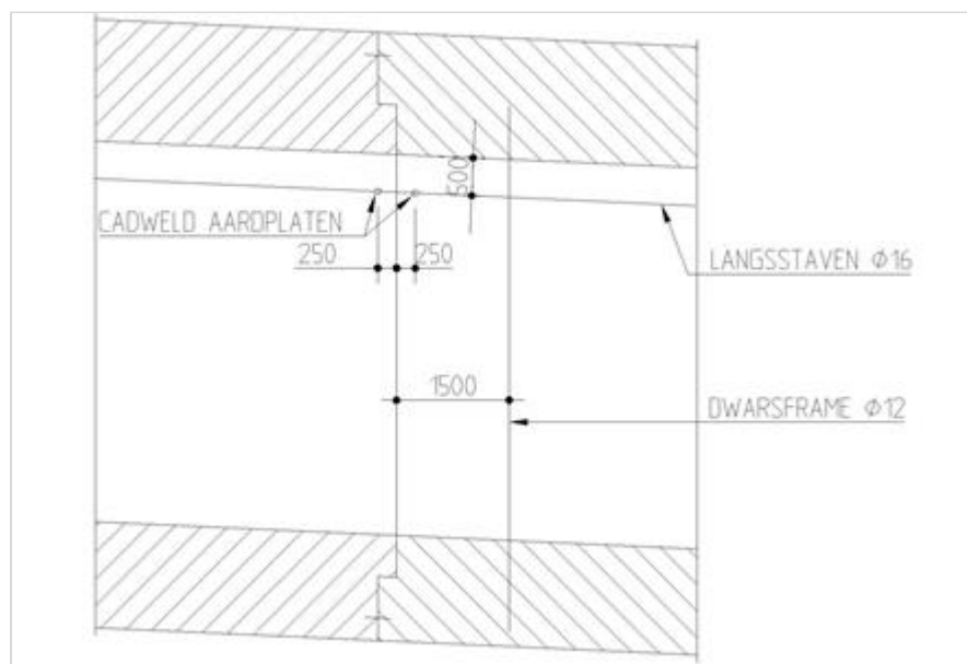
Figuur 288.2 - Aanzicht middenwandkanaal
