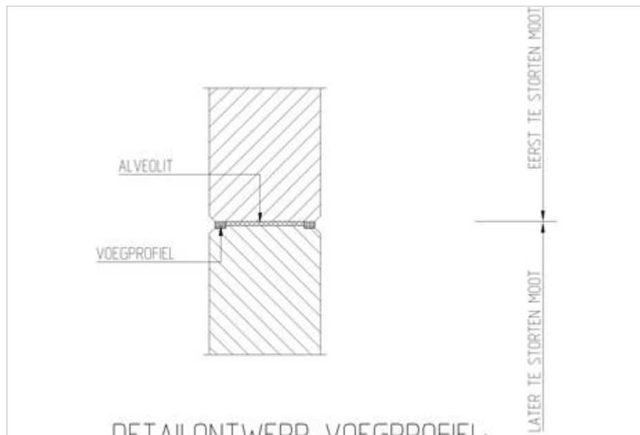
Figuur 254.1 - Voeg in middenwand zonder tegelwerk *)
