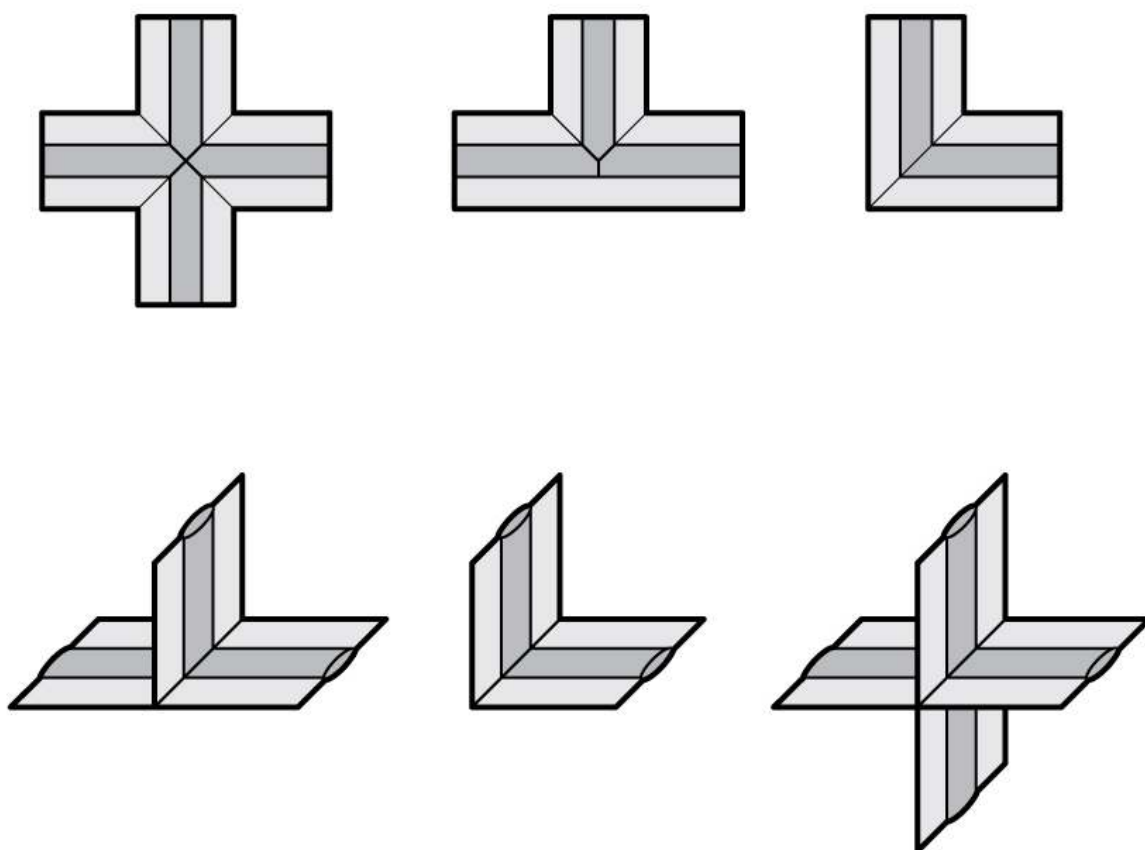
Figuur 93.1 - Vormstukken
