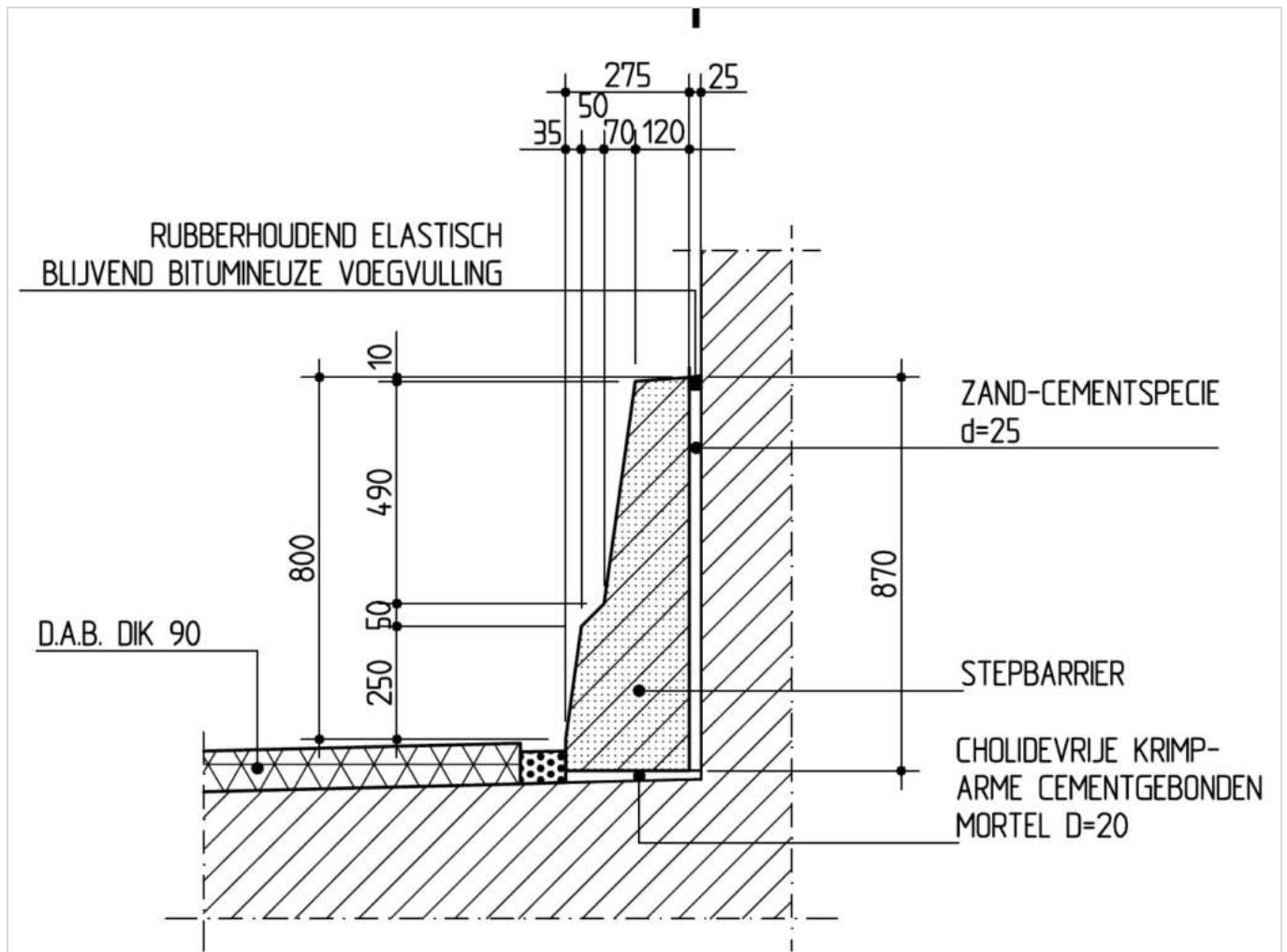
Figuur 452.1 - Doorsnede Stepbarrier bij toepassing DAB
