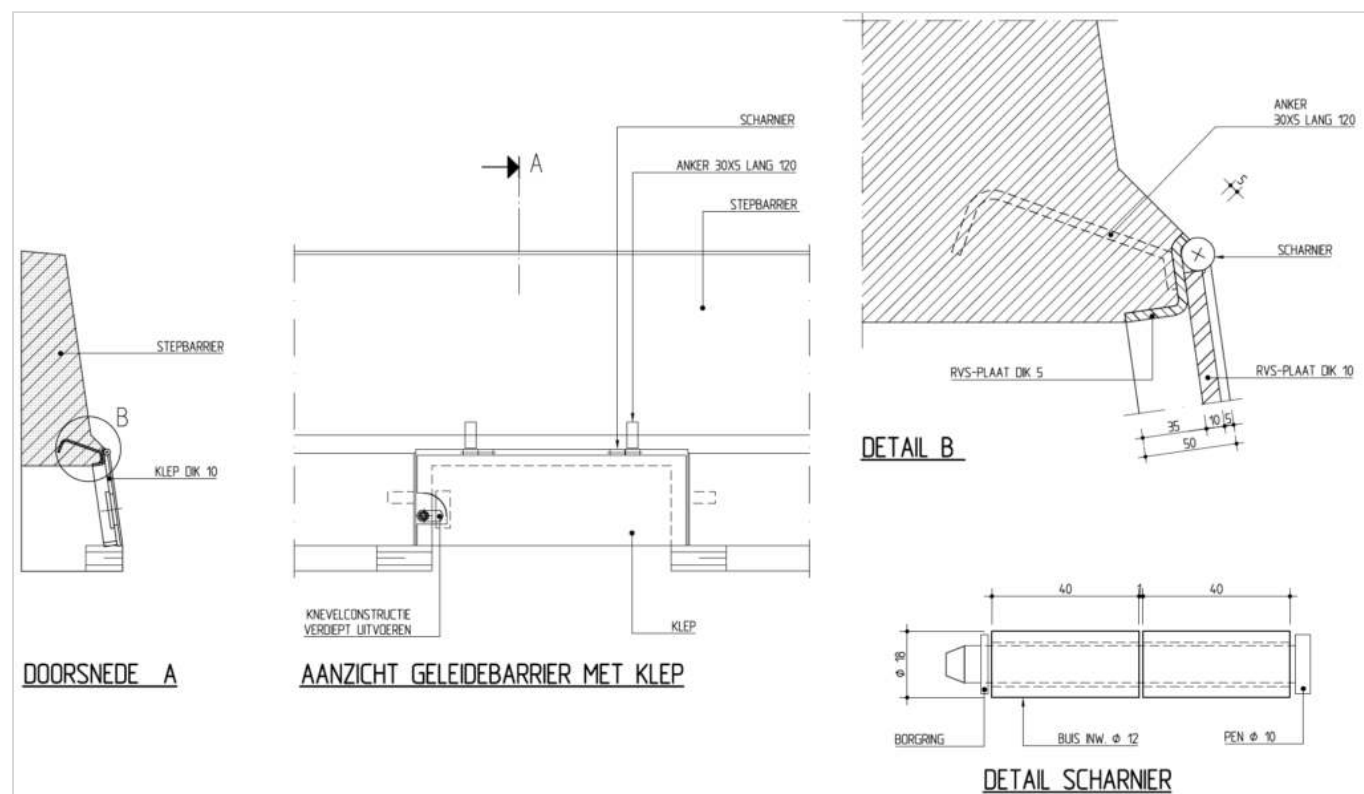
Figuur 457.1 - Aanzicht en details geleidebarrier t.p.v. inlaatput
