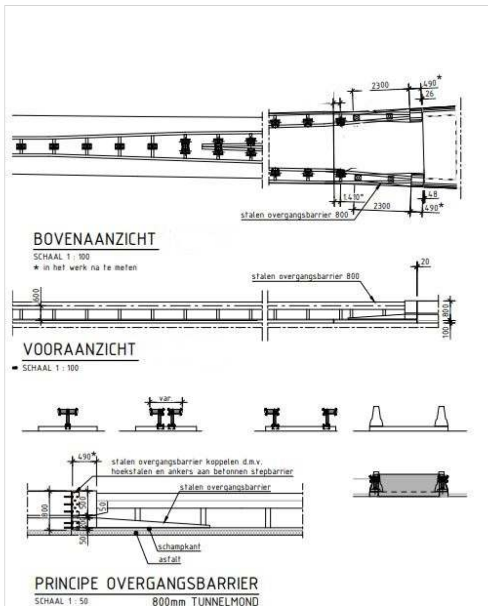
Figuur 459.1 - Detail principe overgang stepbarrier enkele geleideriaal 800mm
