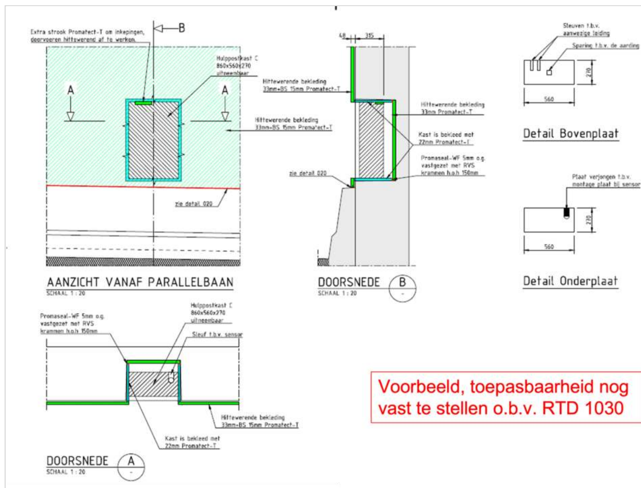
Figuur 498.14 - Detaillering bij hulpkast C: 60 min. brandwerendheid
