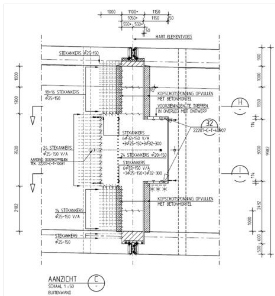
Figuur 370.1 - Tanden tussen de mootvoegen in de wanden van de HSL tunnel onder de Oude Maas.
