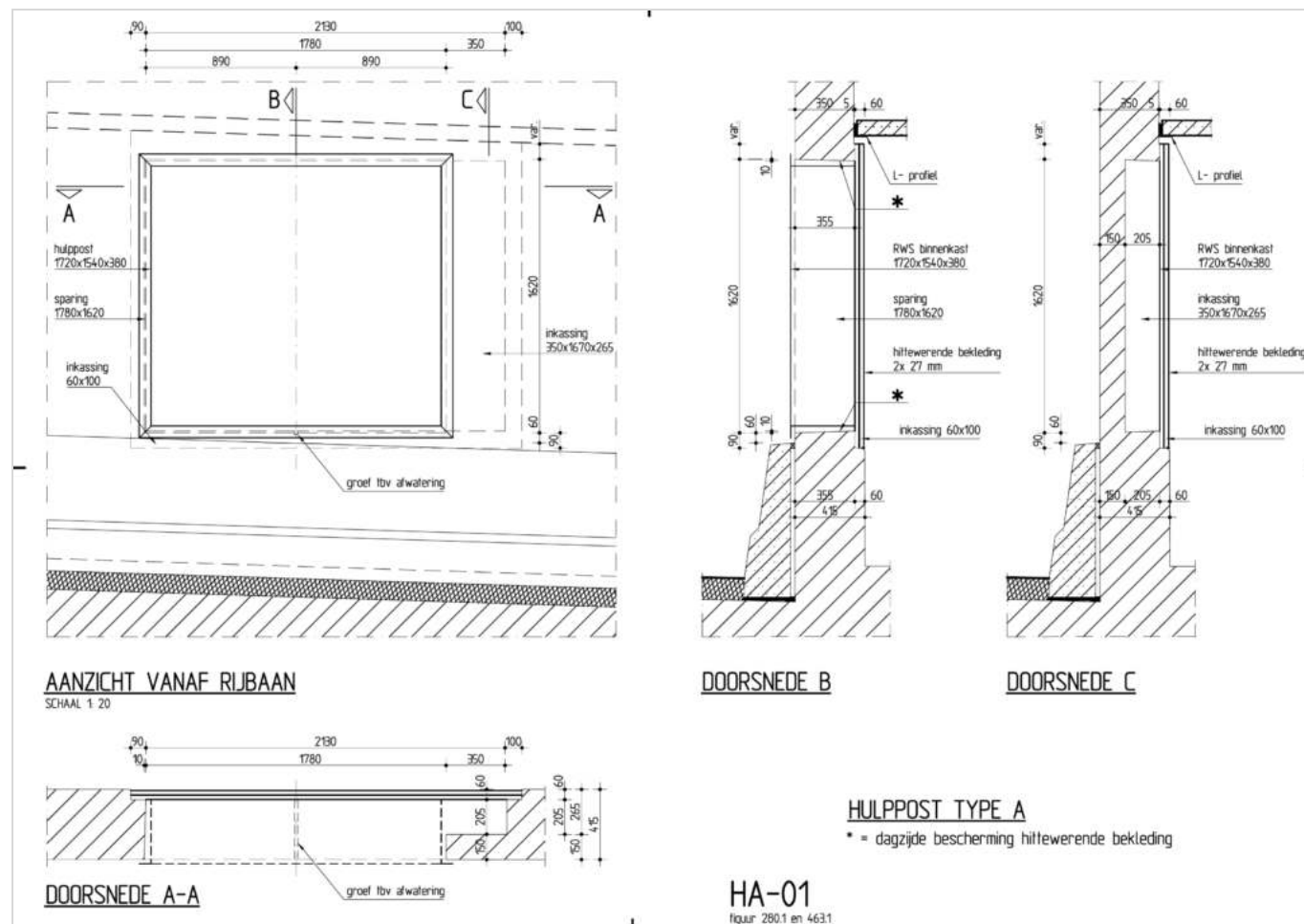
Figuur 463.1 - Afdichting achterzijde hulppost type A en nis brandblusleiding
