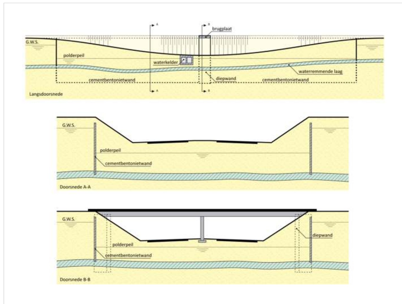
Figuur 201.1 - Kunstmatige polder met cement-bentoniet wand (voorbeeld)
