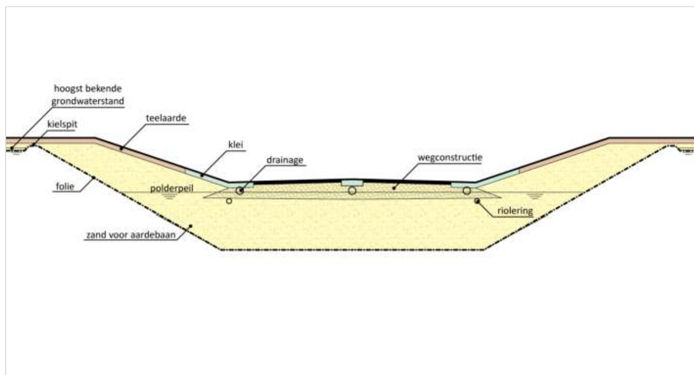
Figuur 228.1 - Oplossing met taluds
