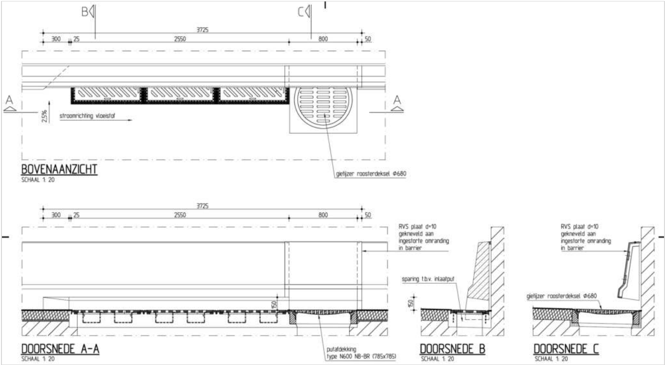
Figuur 409.1 - Inlaatrooster hoofdwatertank bij toepassing ZOAB
