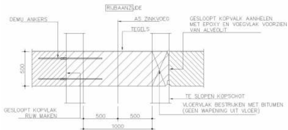
DEATILONTWERP AFWERKING ZINKVOEG MIDDENWAND ( BIJ TOEPASSING STALEN DEUK IN VLOER VERKEERSKOKER )
