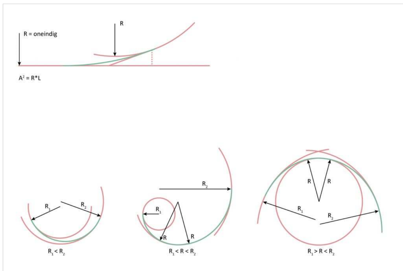
Figuur 19.1 - Clothoïde
