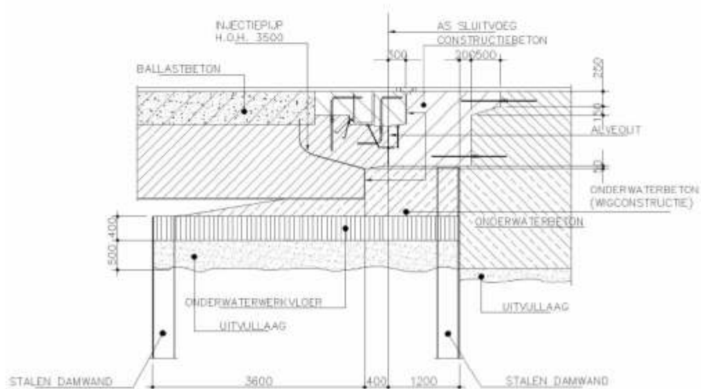
DETAILONTWERP AFWERKING VLOER ( OF STAAL )
