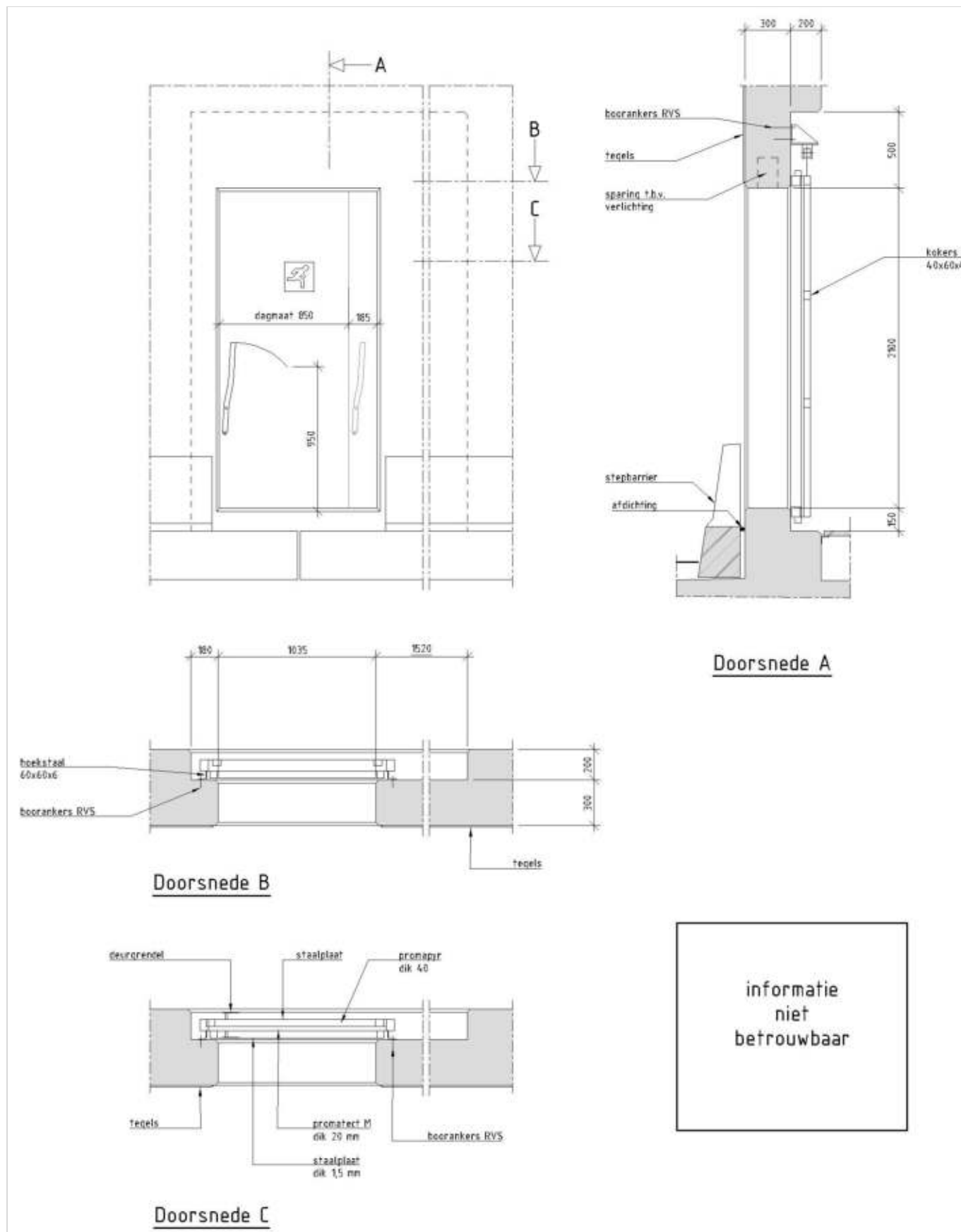
Figuur 490.1 - Kozijn en deur vluchtdoor (schuifdeur)
