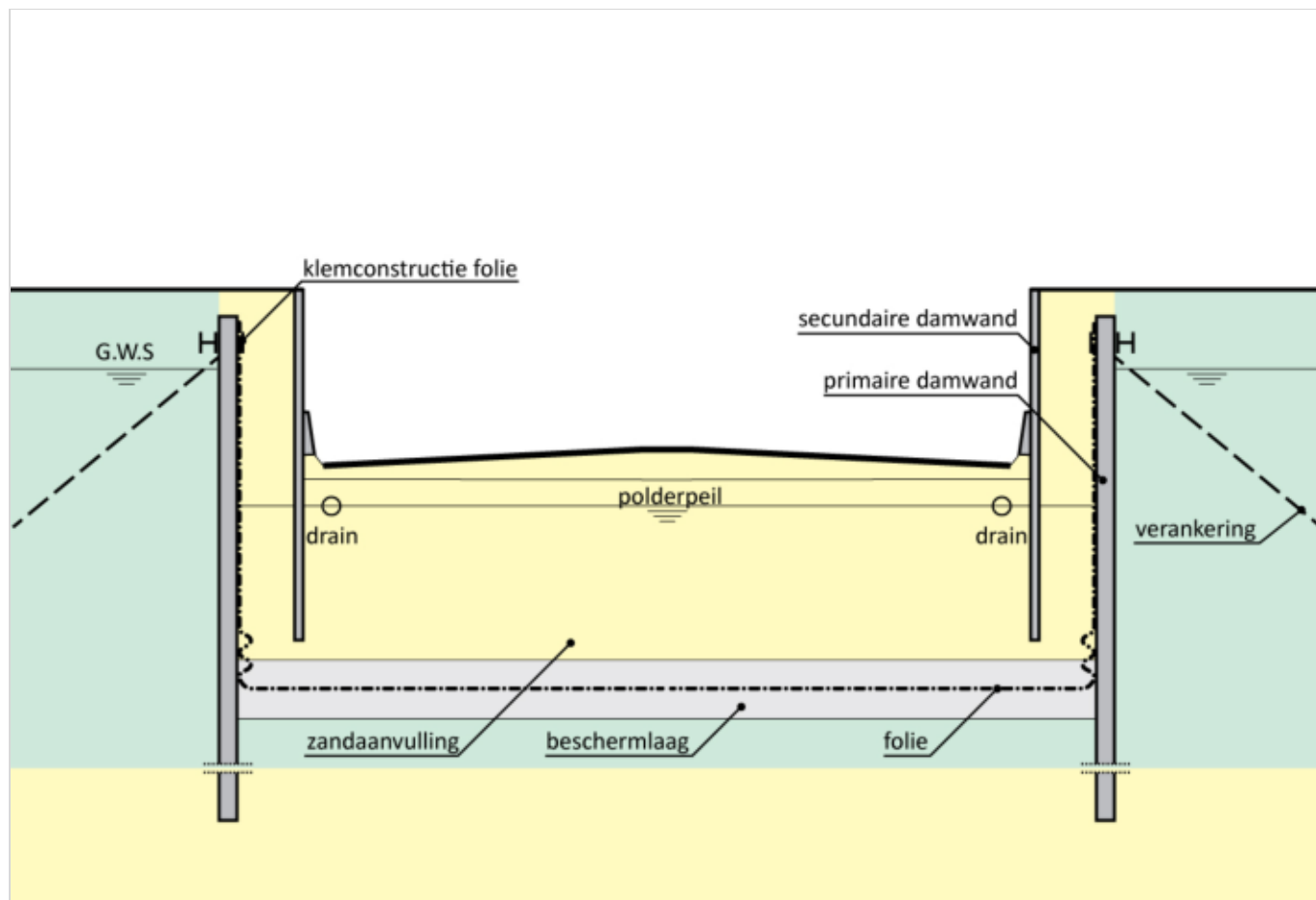
Figuur 228.3 - Smalle constructievarianten
