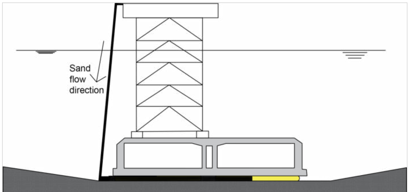
Figuur 241.2 - Zand jetting
