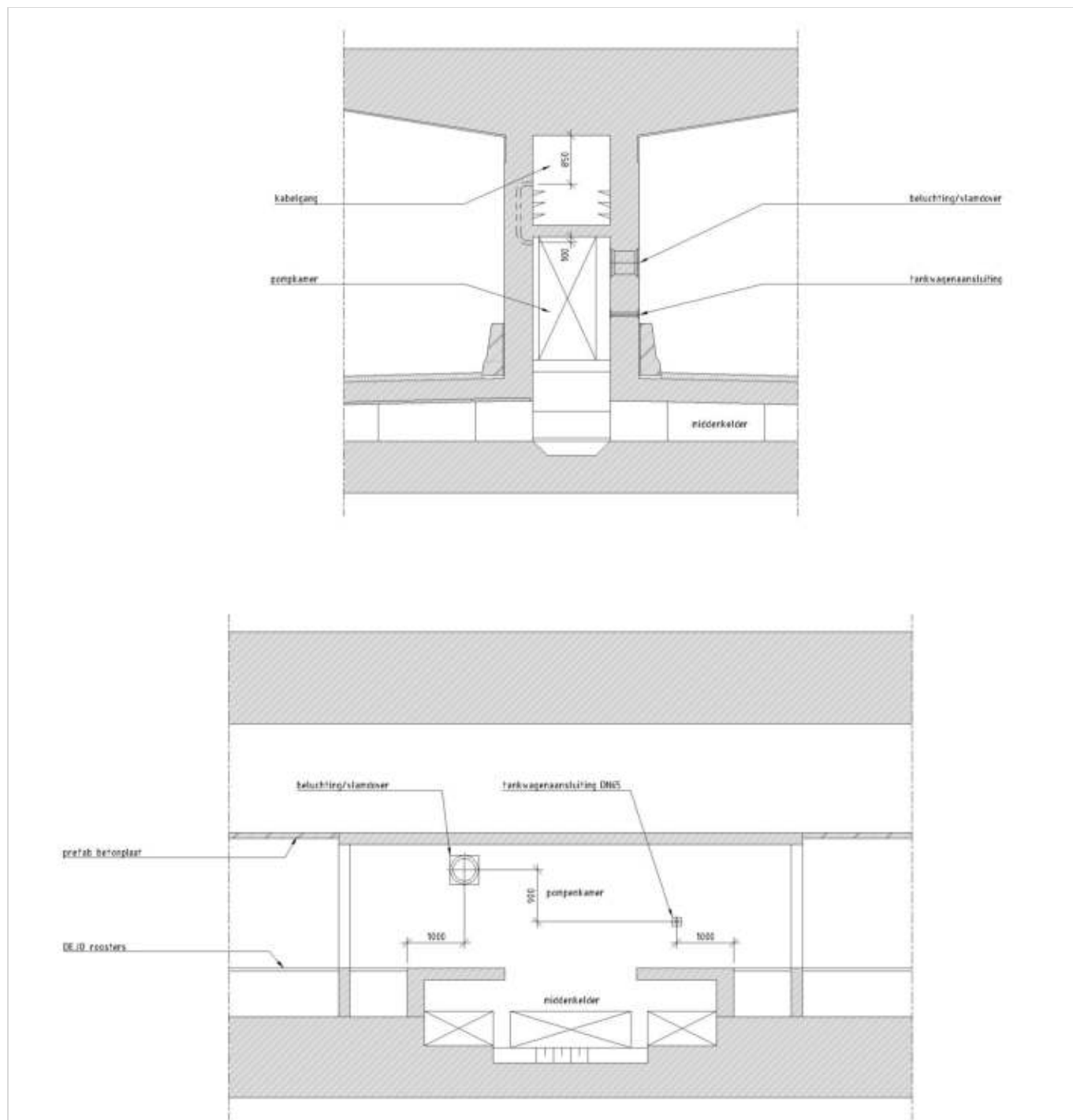
Figuur 302.1 - Dwars- en langsdoorsnede middenpompkamer - vlamdoover en tankwagenaansluiting
