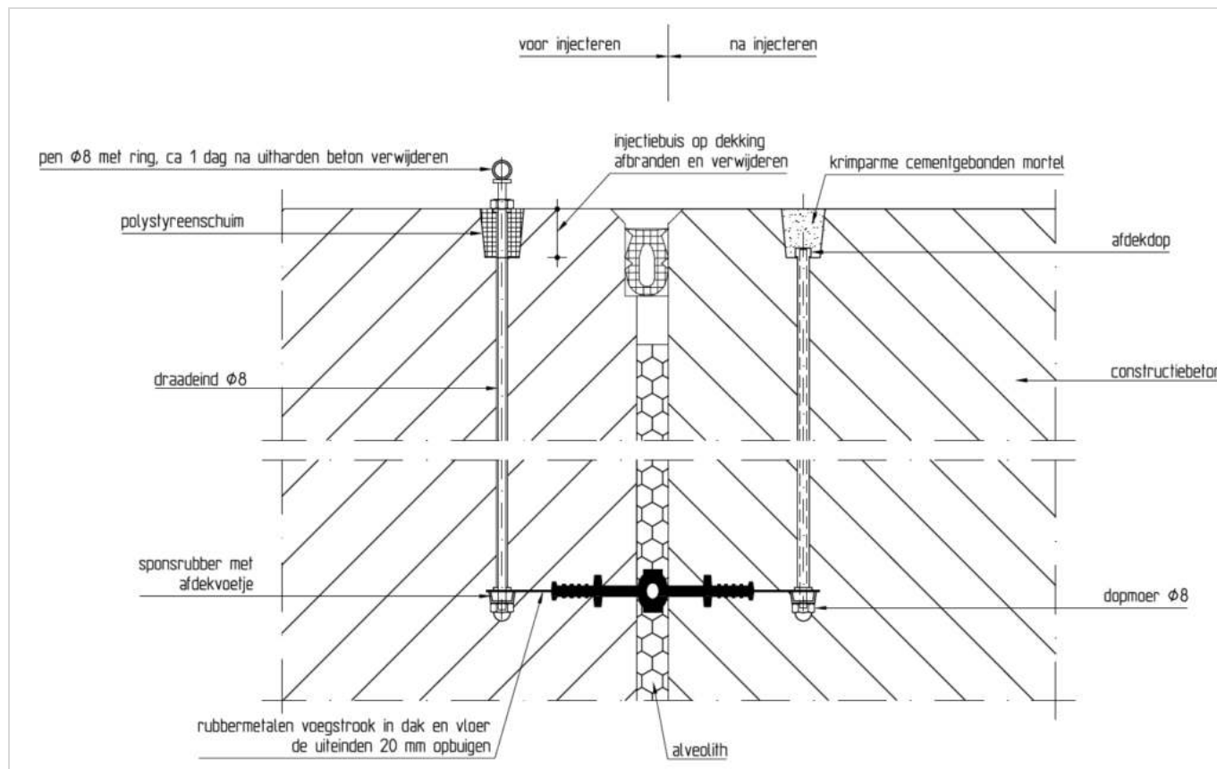
Figuur 269.1 - Detailontwerp rubbermetal voegstrook zonder tand
