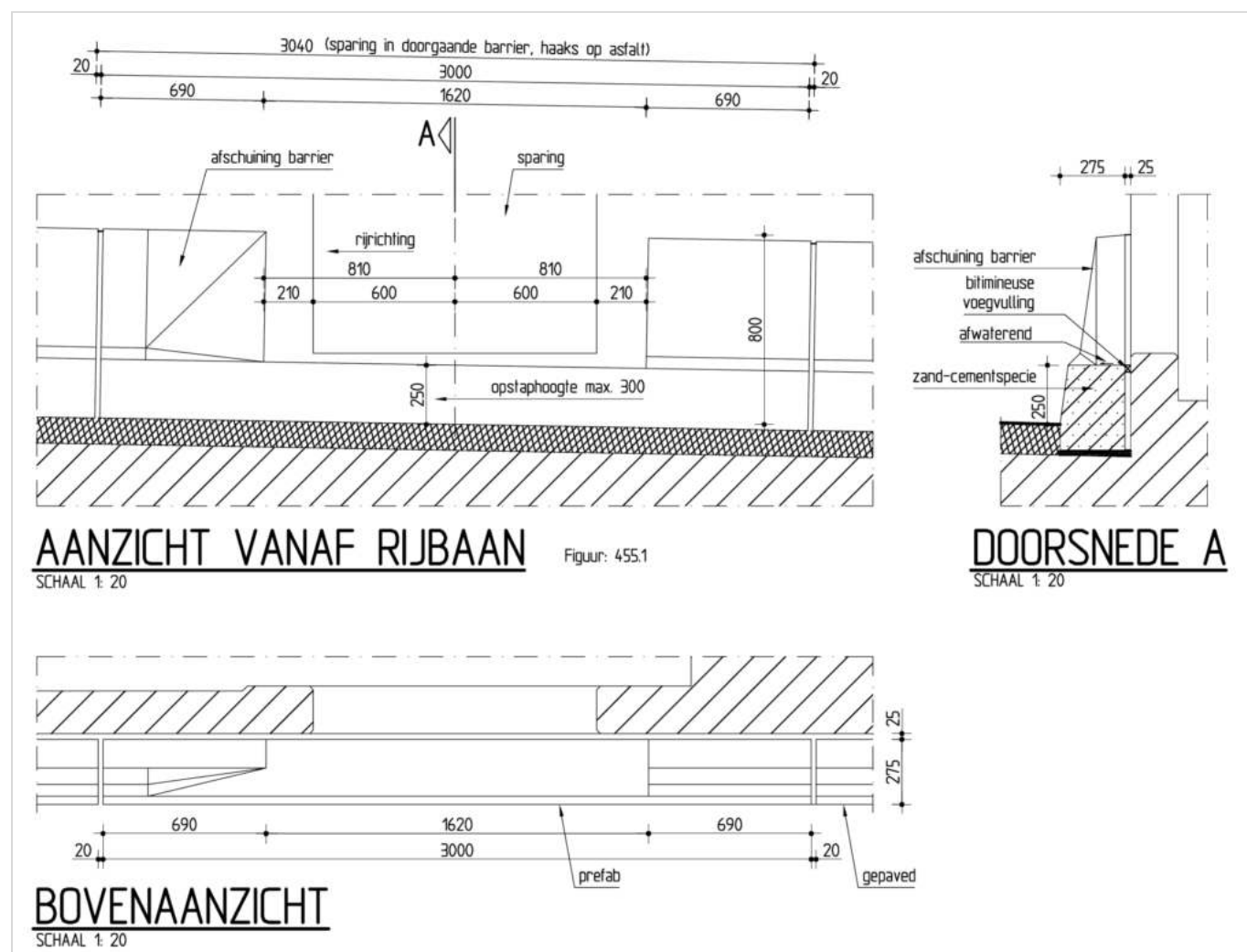
Figuur 455.1 - Geleidebarrier t.p.v. vluchtdeur
