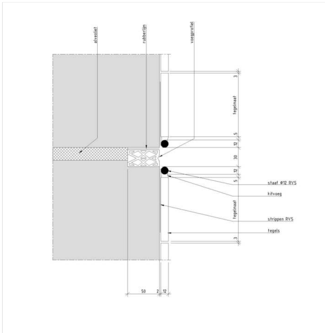
Figuur 264.2 - Detailontwerp tegelwerk - toepassing RVS staaf
