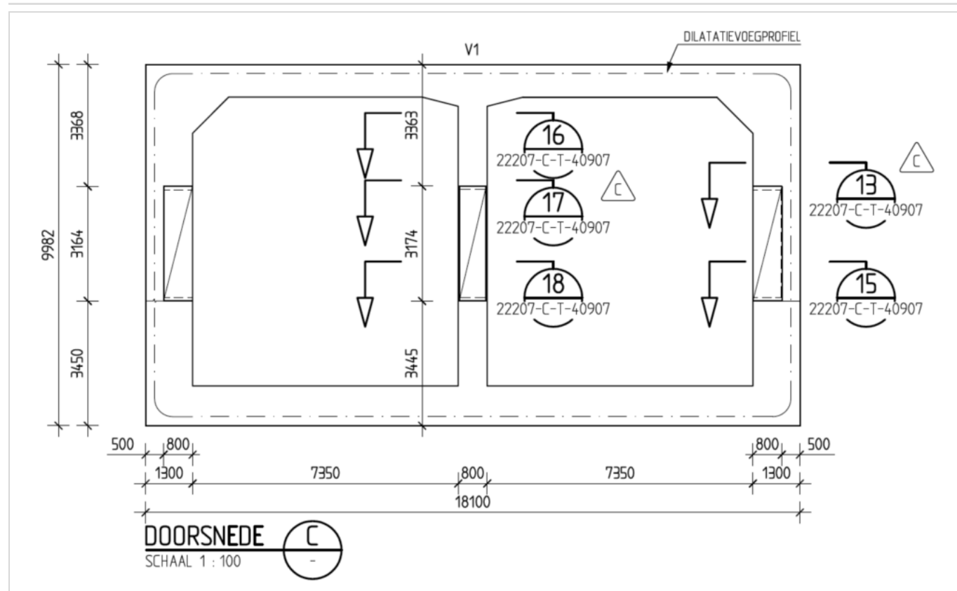
Figuur 370.1 - Tanden tussen de mootvoegen in de wanden van de HSL tunnel onder de Oude Maas.
